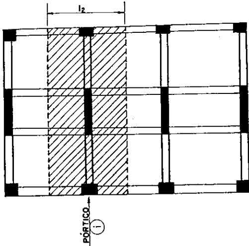
a) PLANTA TÍPICA DA ESTRUTURA ORIGINAL ANALISADA
