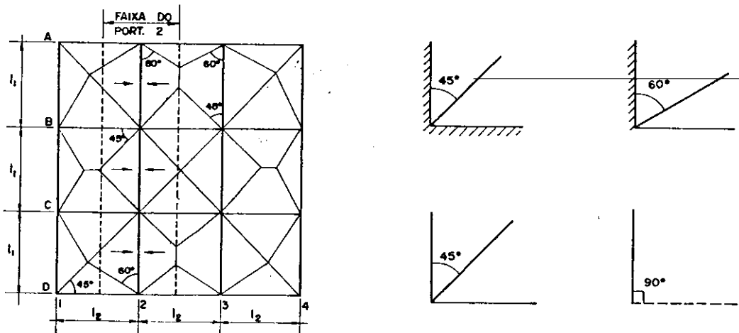
FIG. I.12 - ESQUEMA DE DISTRIBUIÇÃO DE CARGAS PARA AS VIGAS EQUIVALENTES, SEGUNDO CRITÉRIO DA NB-1/78.
