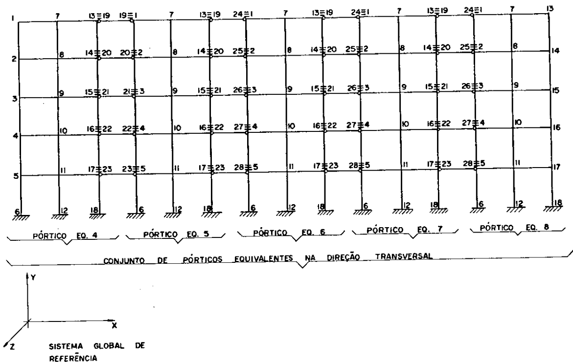
FIG. II.3 - NUMERAÇÃO DOS PONTOS NODAIS, DO CONJUNTO DE PÓRTICOS EQUIVALENTES NA DIREÇÃO TRANSVERSAL.
