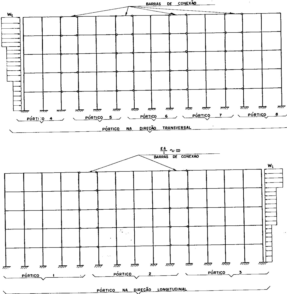
FIG. I.16 - ESQUEMA DA ASSOCIAÇÃO EM SÉRIE DOS PÓRTICOS EM UMA MESMA DIREÇÃO, ATRAVÉS DE BARRAS DE CONEXÃO, SIMULANDO A INDEFORMABILIDADE DA LAJE, PARA A IDEIA LIZAÇÃO DO CONJUNTO DE PÓRTICOS PLANOS DA FIGURA I.10
