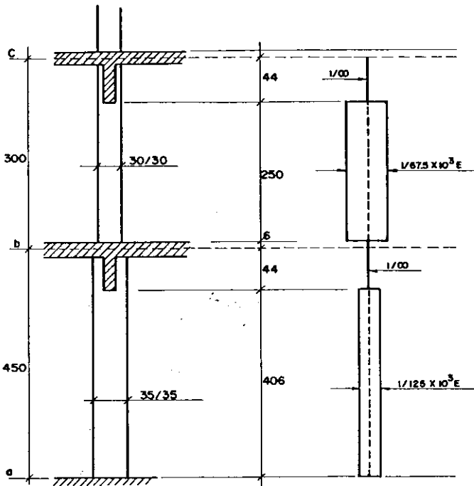
DIAGRAMA DE VARIAÇÃO DE 1/EI
