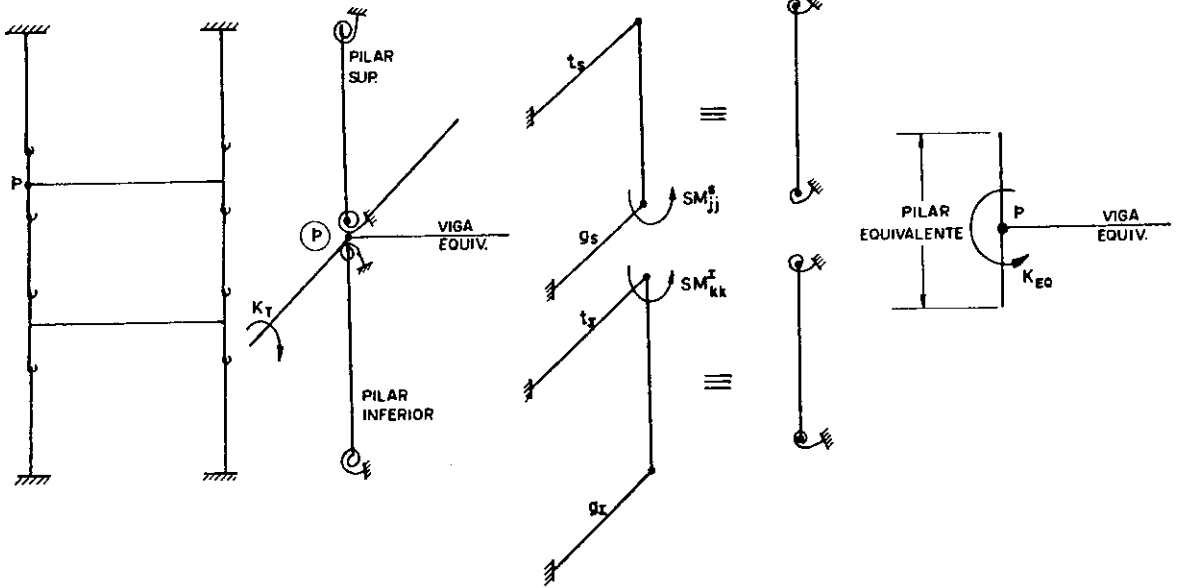
FIG. I.11 - ESQUEMA PARA CONSIDERAÇÃO DA RIGIDEZ DA MOLA EQUIVALENTE, AO SE ASSOCIAR EM SÉRIE O PILAR DA ESTRUTURA ORIGINAL E À VIGA TRANSVERSAL AO PÓRICO EM ANÁLISE, (NÓ p).
