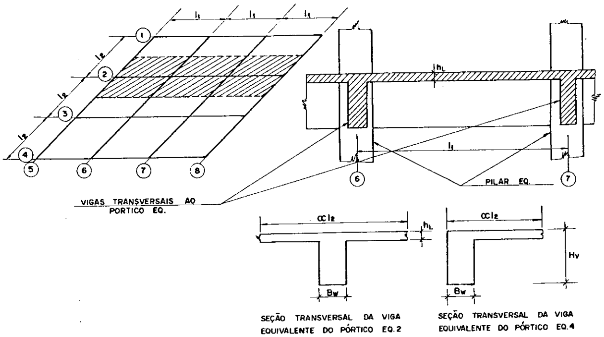
FIG. I.2 - LARGURA DE FAIXA, COM A QUAL SE DEFINIU O PÓRICO EQUIVALENTE E AS SEÇÕES TRANSVERSAIS DAS VIGAS EQUIVALENTE.
