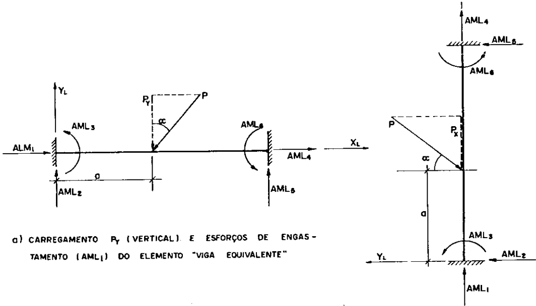
b) CARREGAMENTO P_x (VERTICAL) E ESFORÇOS DE ENGASTAMENTO PERFEITO (AML 1 ) DO ELEMENTO "PILAR EQUIVALENTE"
