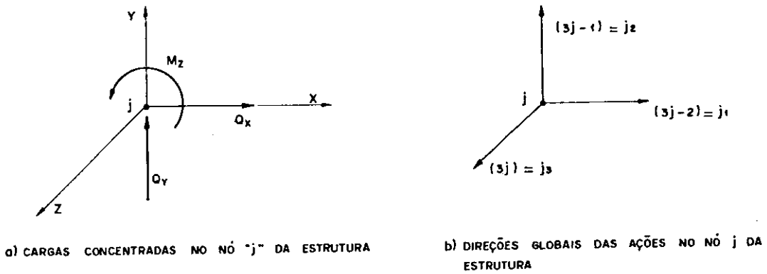
FIG. IV.7 - DIREÇÕES DAS CARGAS APLICADAS DIRETAMENTE NOS NÓS.
