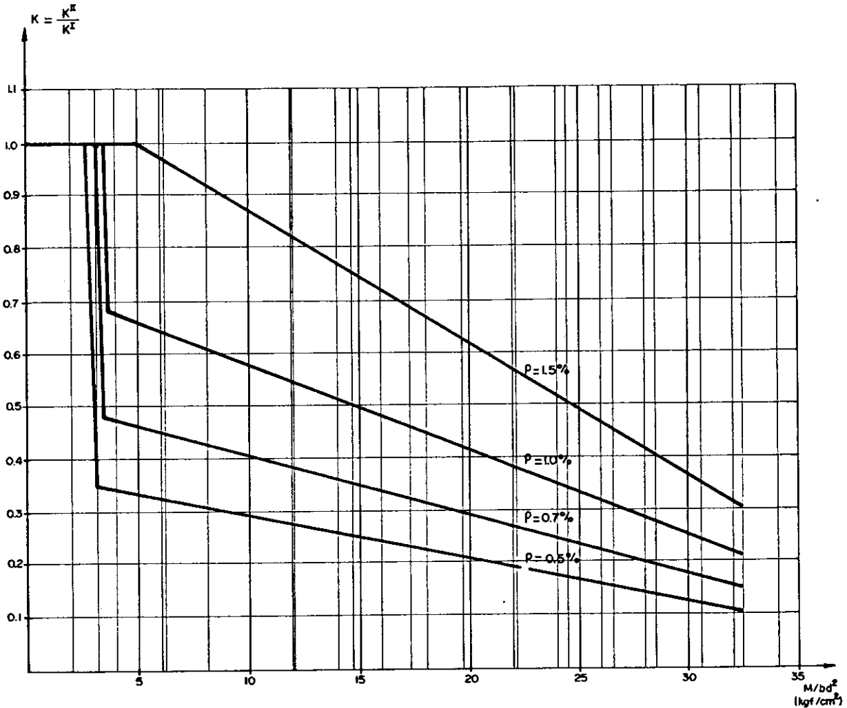
FIG. A1-2 - RELAÇÃO ENTRE AS RIJEZAS À FLEXÃO, NO ESTÁDIO II E NO ESTÁDIO I, RESPECTIVAMENTE, EM FUNÇÃO DO AUMENTO DE SOLICITAÇÃO E DA TAXA DE ARMADURA.
