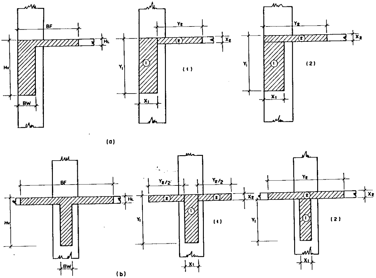
FIG. I.10 - SEÇÕES TRANSVERSAIS PARA DETERMINAÇÃO DO MOMENTO DE INÉRCIA Á TORÇÃO.
