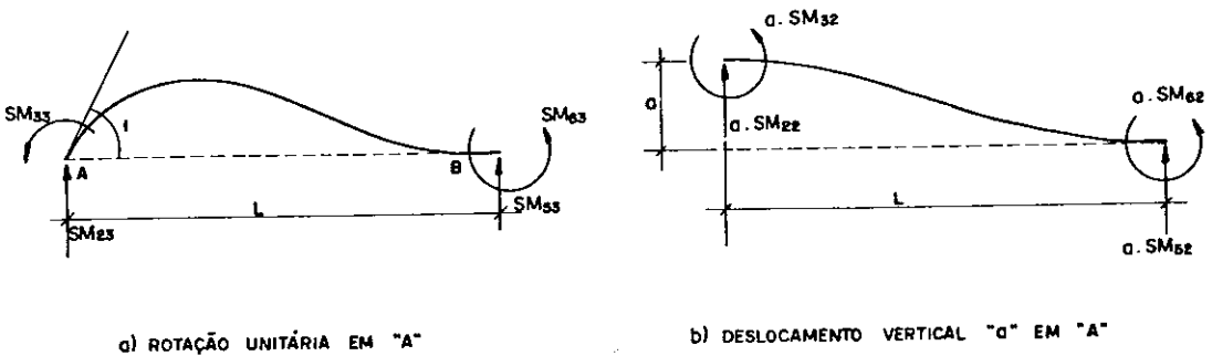
a) ROTAÇÃO UNITÁRIA EM "A"
