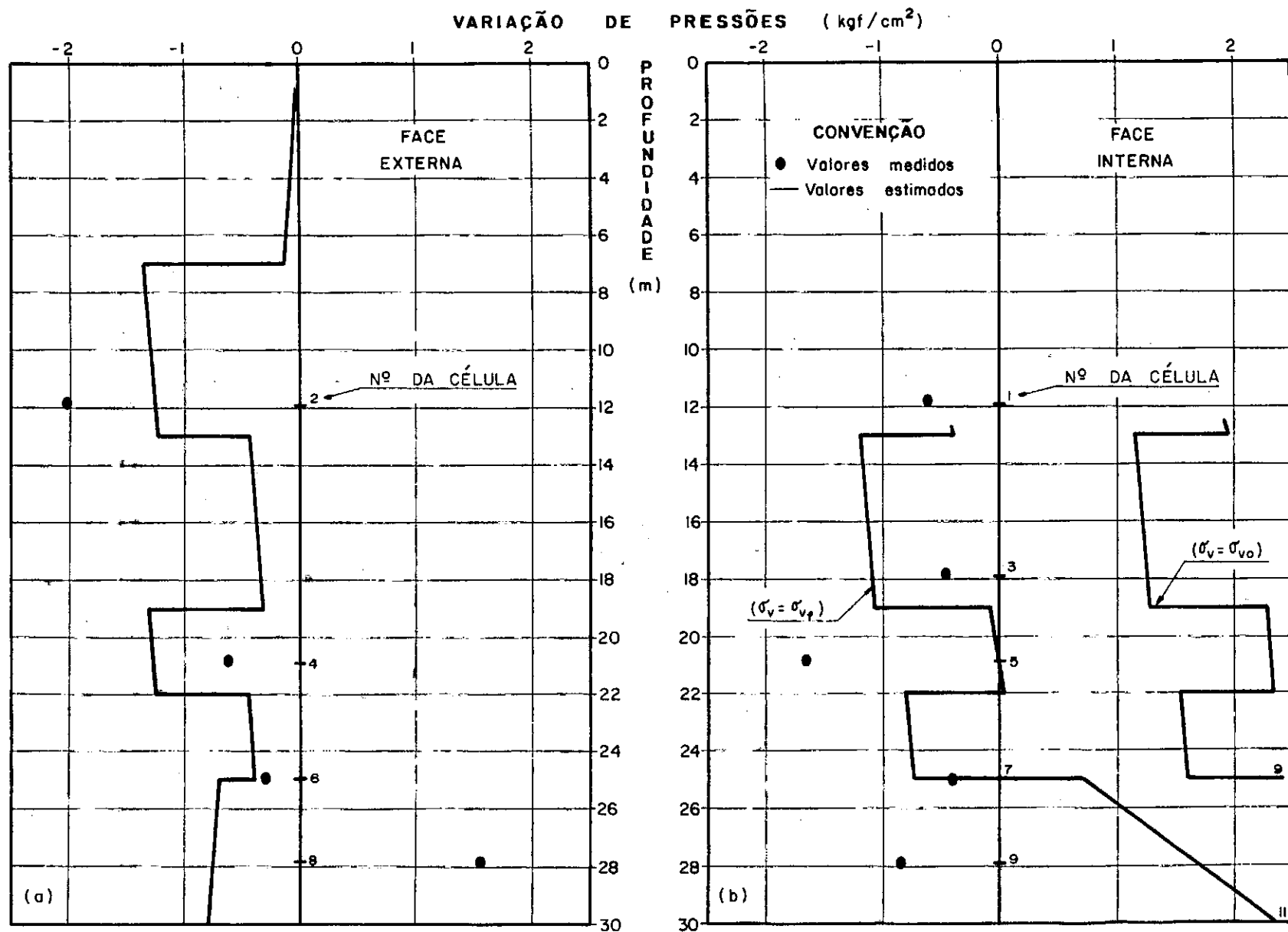
FIG. 57 - Variação de pressões medidas e estimadas devido a escavação da vala.
