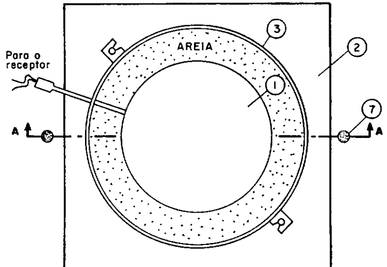
CORTE BB
