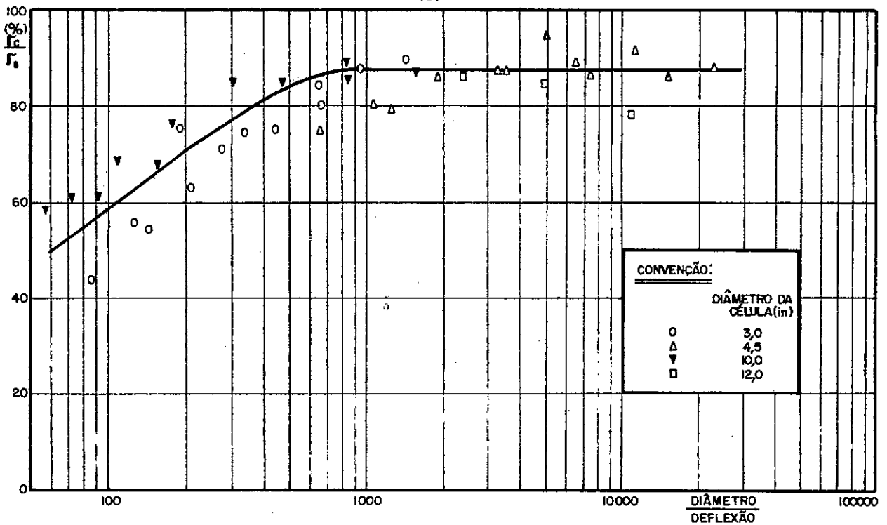
Fig. 33 — Influência do ressalto e da rigidez de células instaladas em frente (Wes, 1944).
