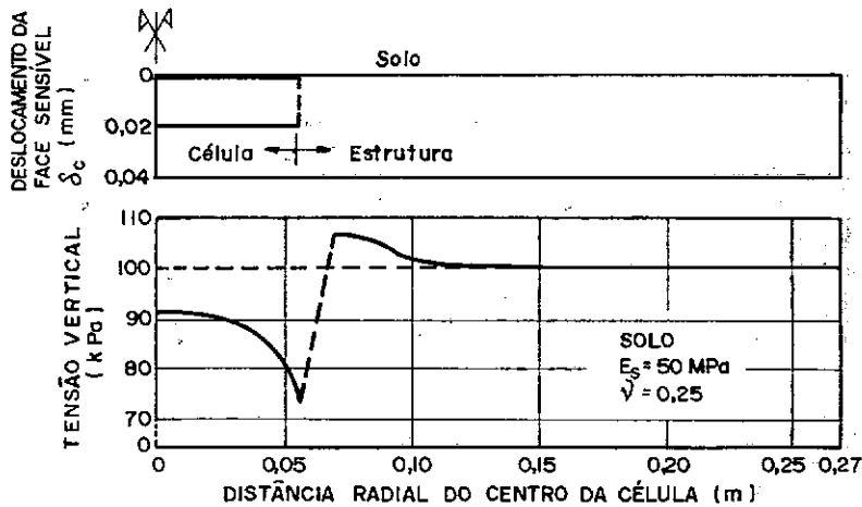
FIG. 17 — Distribuição teórica de tensões sobre célula tipo pistão em fronteira rígida (CARDER, 1976).
