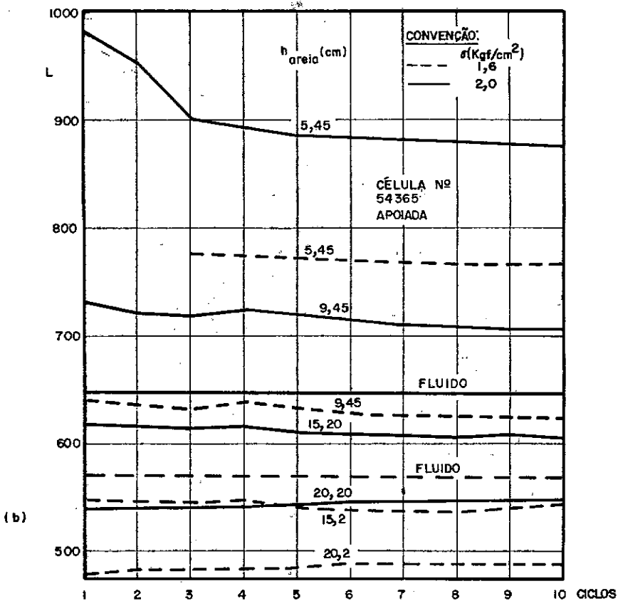
Fig. 46 — Influência da espessura de areia nas leituras com \sigma=1,6 ; 2,0; 3,0 e 4,0 \text{kgf/cm}^2 aplicada na superfície da areia.
