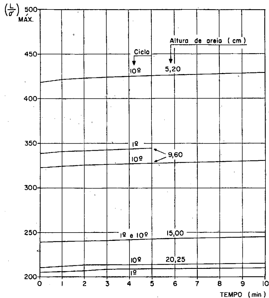
FIG. 50—Influência do tempo de aplicação de carga e dos ciclos de carregamento na calibração da célula nº 54365 envolta em parafina.
