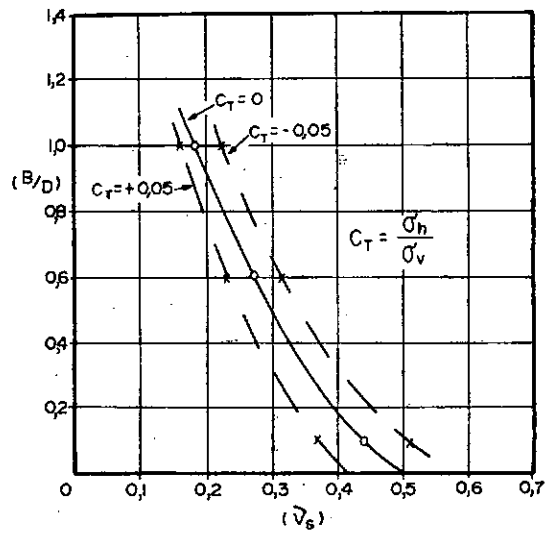
FIG. 32 - Curvas para limitar a sensibilidade transversal ( BROWN , 1977 ).
