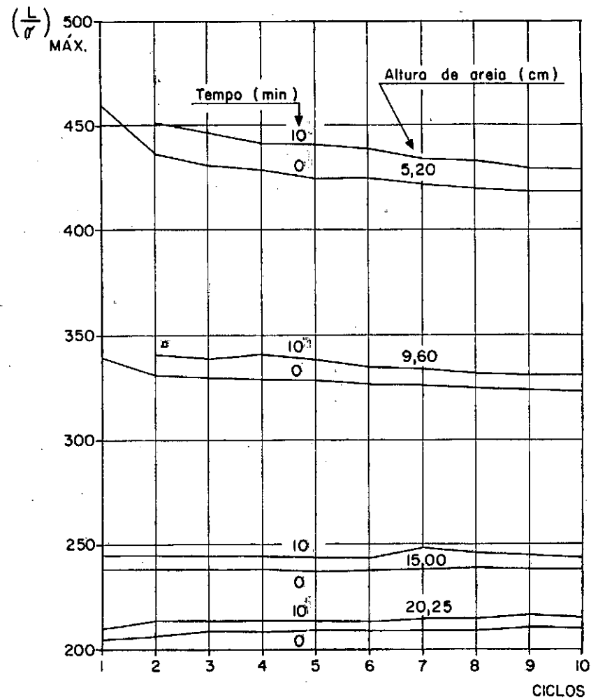
FIG. 50—Influência do tempo de aplicação de carga e dos ciclos de carregamento na calibração da célula nº 54365 envolta em parafina.
