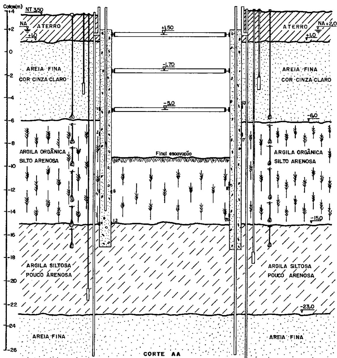
Fig.39 — Localização da instrumentação no lote 3 (Uruguiana).
