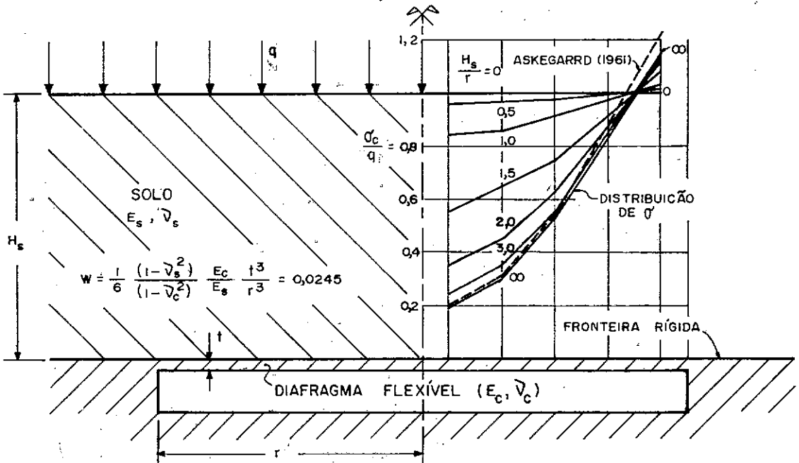
FIG. 21 - Distribuição teórica de tensões sobre diafragma flexível em fronteira rígida (STAIN, 1971).
