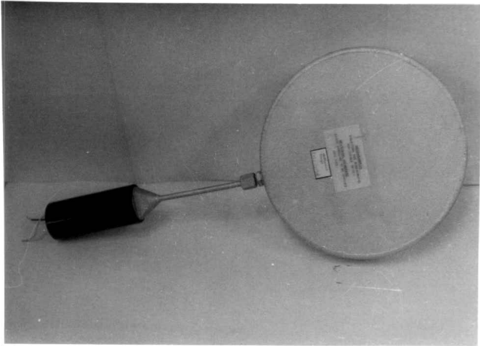
Foto 2 - Lote 9 (Botafogo) - Célula de Pressão Total Tipo Fluido Confinado Acústico.
