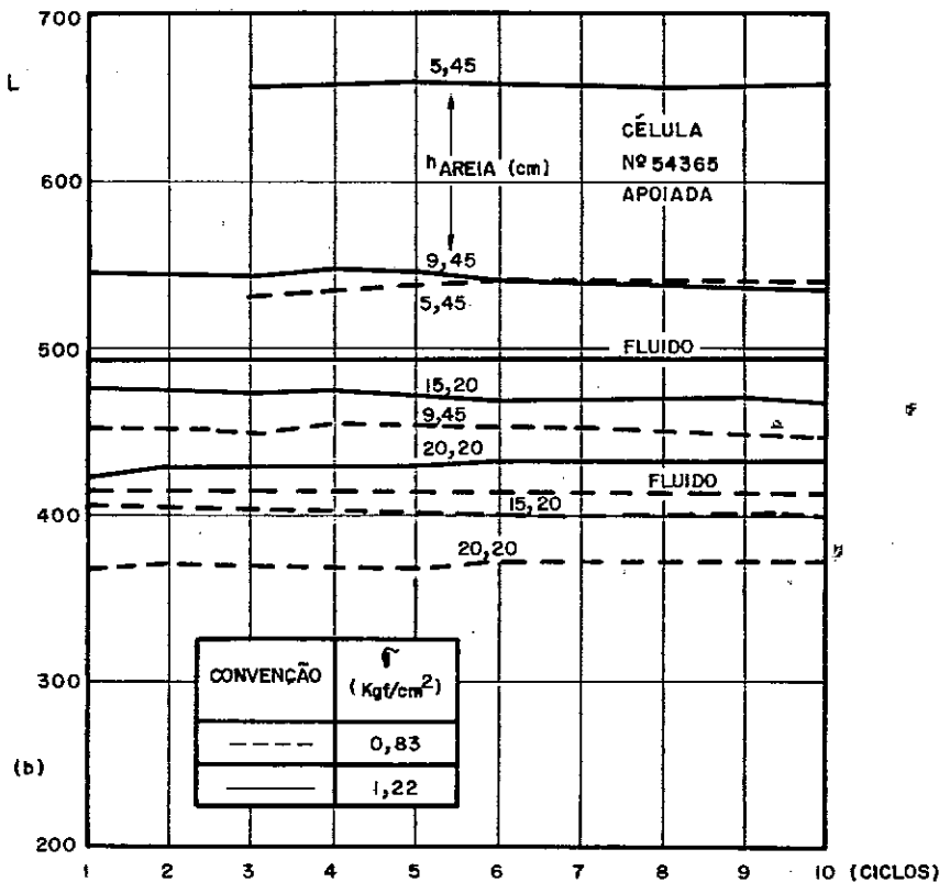
fig. 47 — Influência da espessura de areia nas leituras com f = 0,83 e 1,22 \text{ kgf/cm}^2 aplicado na superfície da areia.
