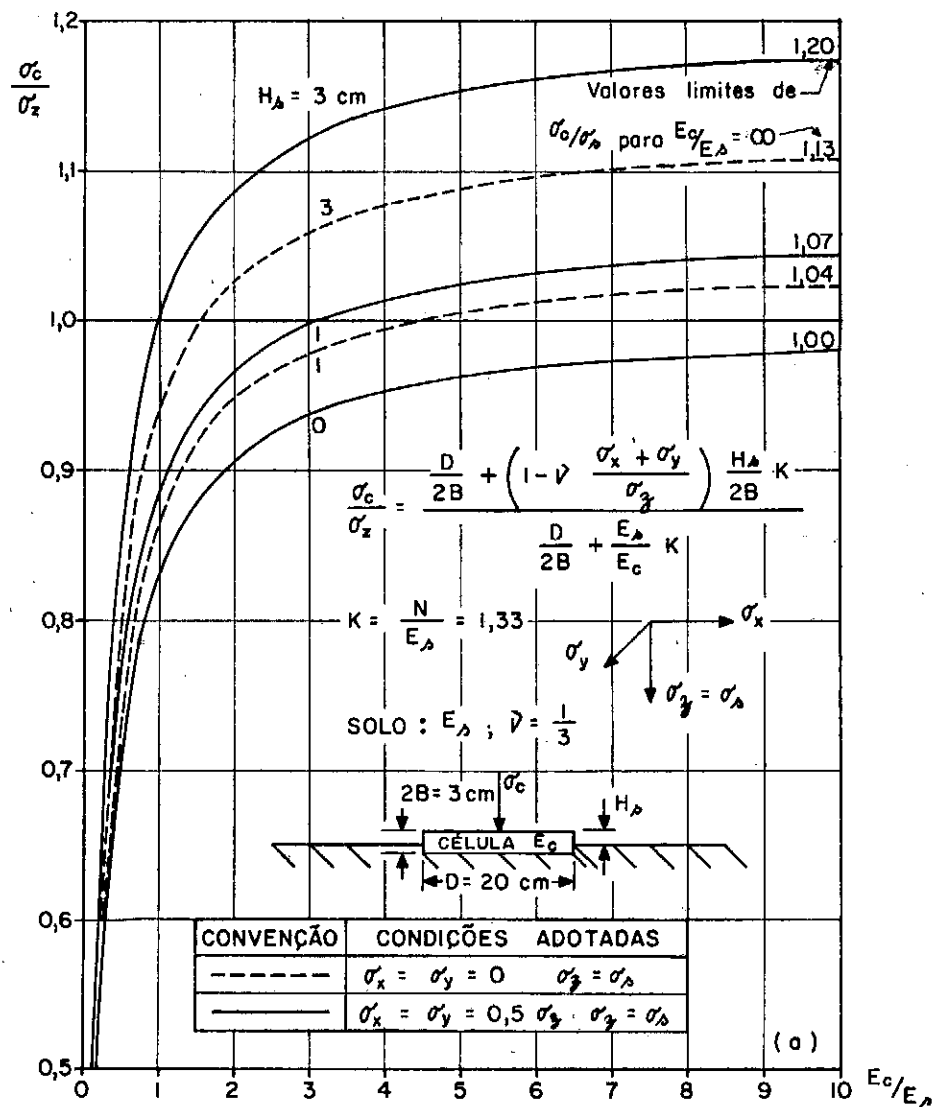
FIG. 16 — Relação \sigma_c/\sigma_\lambda para células em fronteira rígida (HVORSLEV, 1974 - modificado.)
