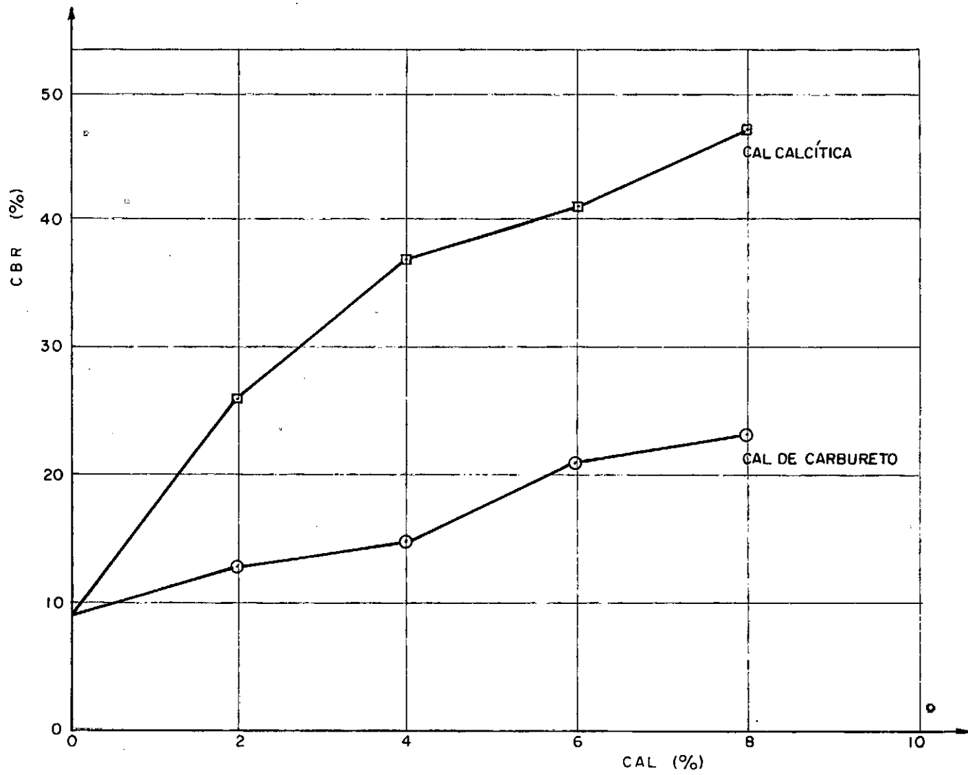
FIG.11.3 — Variação do CBR do solo em relação ao teor de cal usada, umidade 20 %, rompimento após cura e imersão
