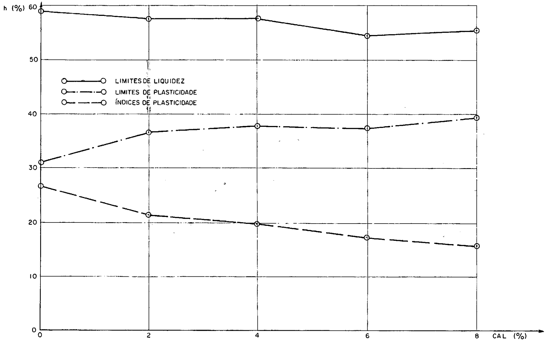
FIG.7.1 —Variação dos limites de Atterberg para solo-cal calcítica, a 0%, 2%, 4%, 6% e 8%, em relação ao peso do solo seco, a um tempo de cura de 2 horas
