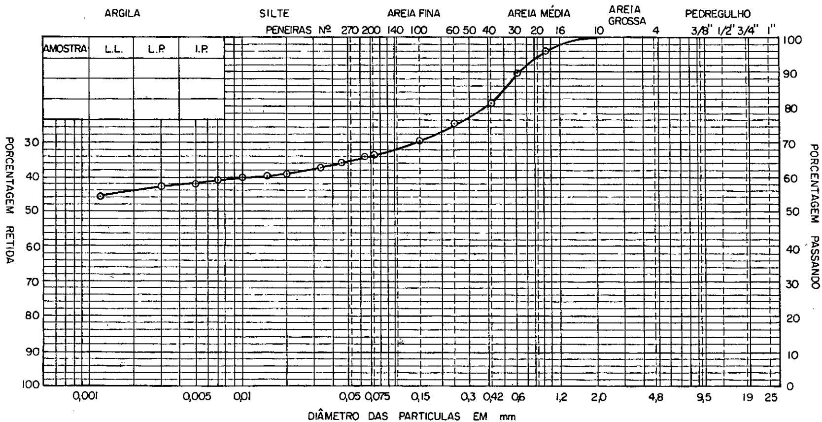
FIG. 4.1 — Análise granulométrica
