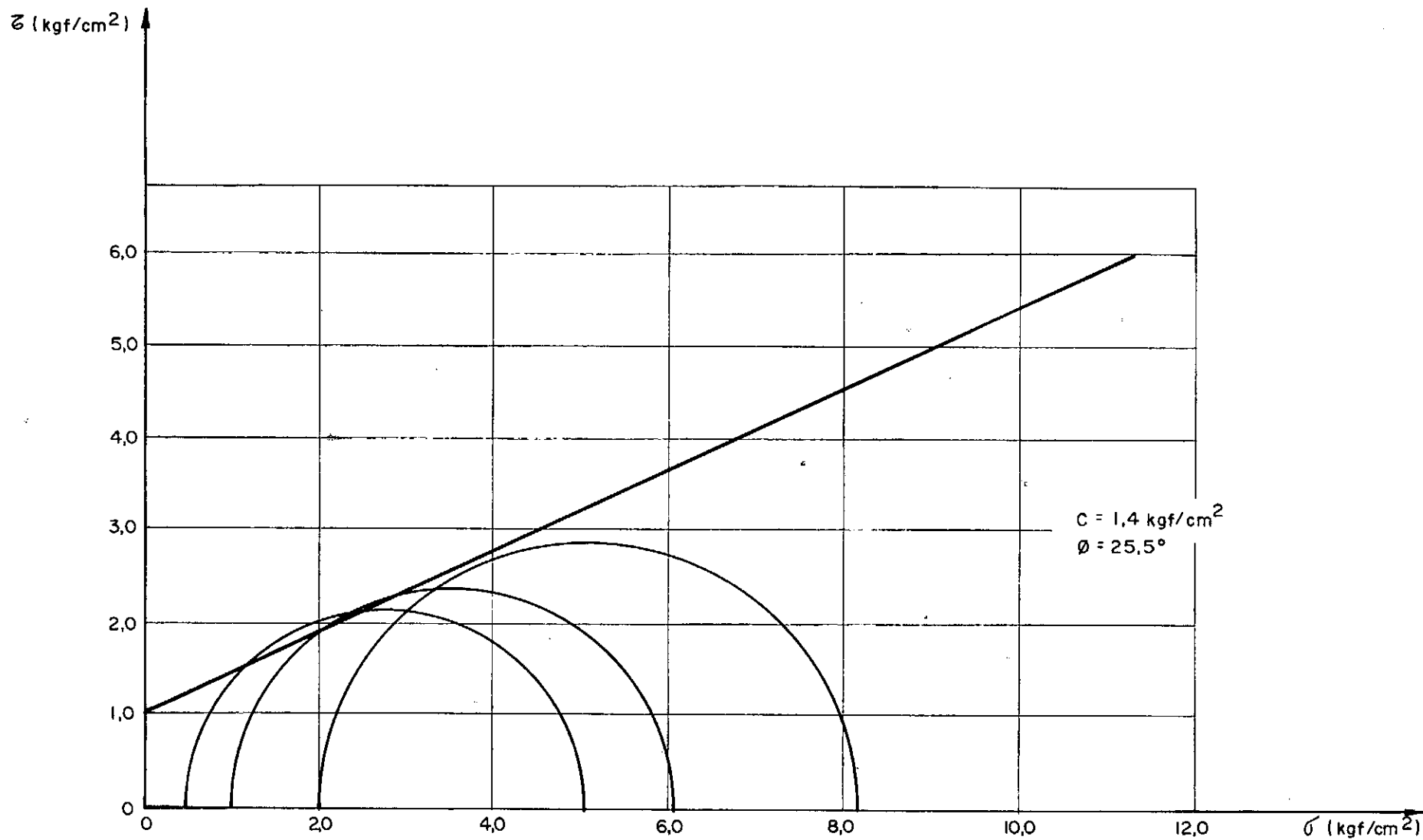
FIG. 13.7 — Envoltória de Mohr. Ensaio C.U. Pressões totais. Solo - cal calcítica
