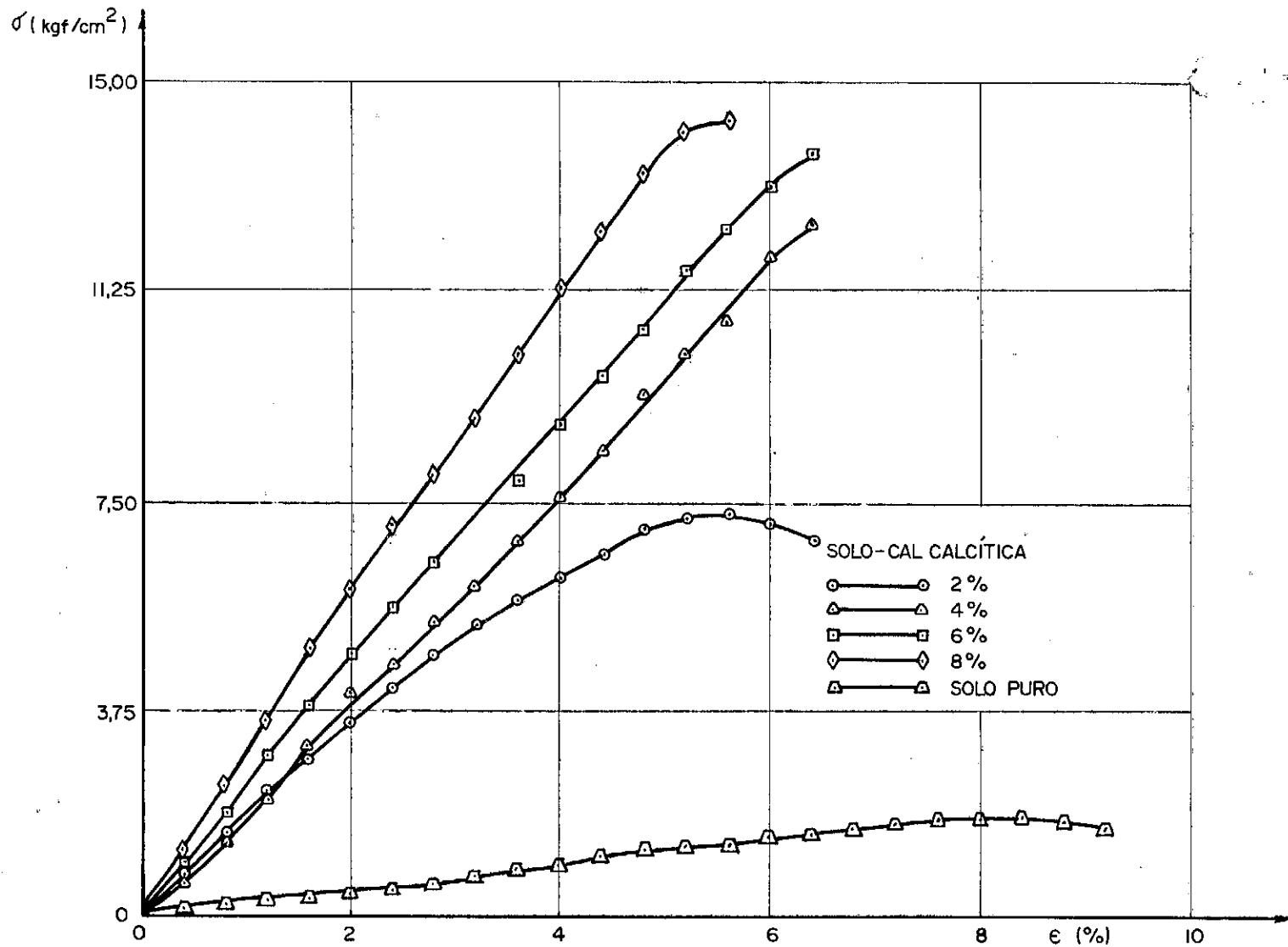
FIG.12.5 — Tensão versus deformação do solo-cal calcífrica, no ensaio de resistência à compressão não confinada, a uma cura de 7 dias
