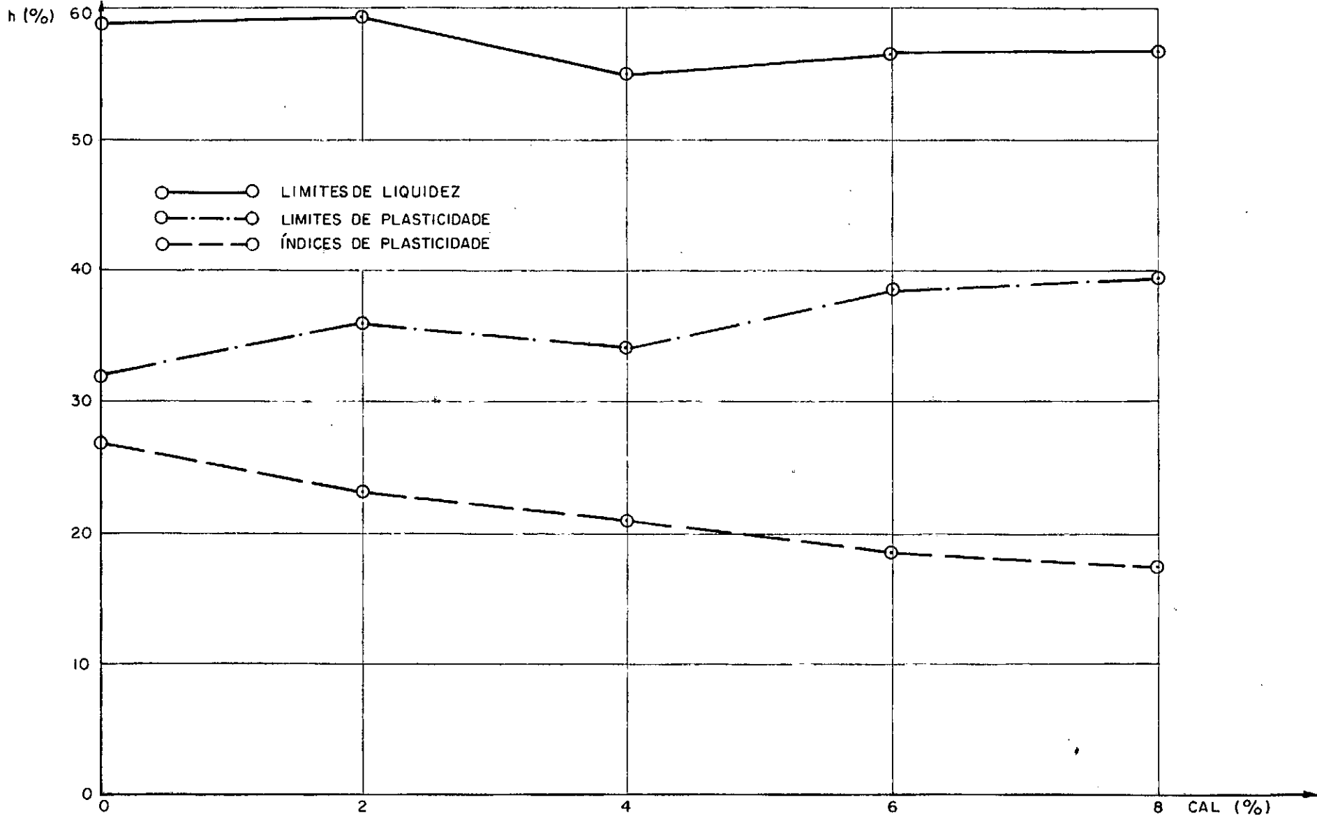
FIG.7.2 —Variação dos limites de Atterberg p/ solo puro e solo-cal de carbureto, a 2%, 4%, 6% e 8%, em relação ao peso de solo seco, a um tempo de cura igual a 2 horas
