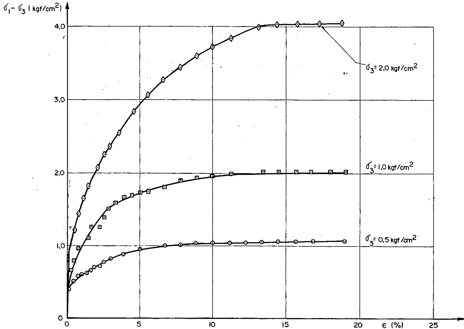
FIG.13.3 — Curvas tensão-deformação, para solo-cal de carbureto, a tensões confinantes iguais a 0,5 kgf/cm 2 , 1,0 kgf/cm 2 e 2,0 kgf/cm 2
