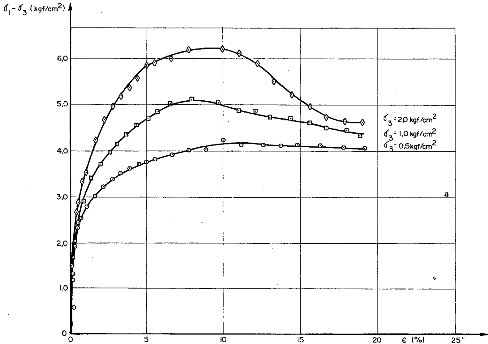
FIG. 13.4 — Curvas tensão-deformação, para solo-cal calcífica, a tensões confinante iguais a 0,5 kgf/cm 2 , 1,0 kgf/cm 2 e 2,0 kgf/cm 2
