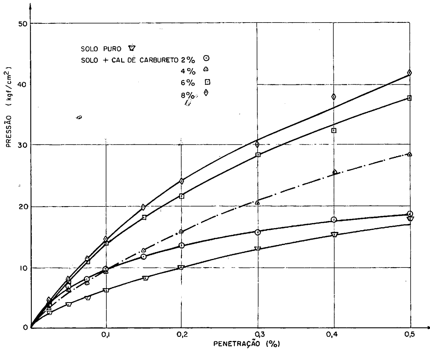
FIG. II.1 — Curva de pressão versus penetração do solo puro e solo-cal de carbureto
