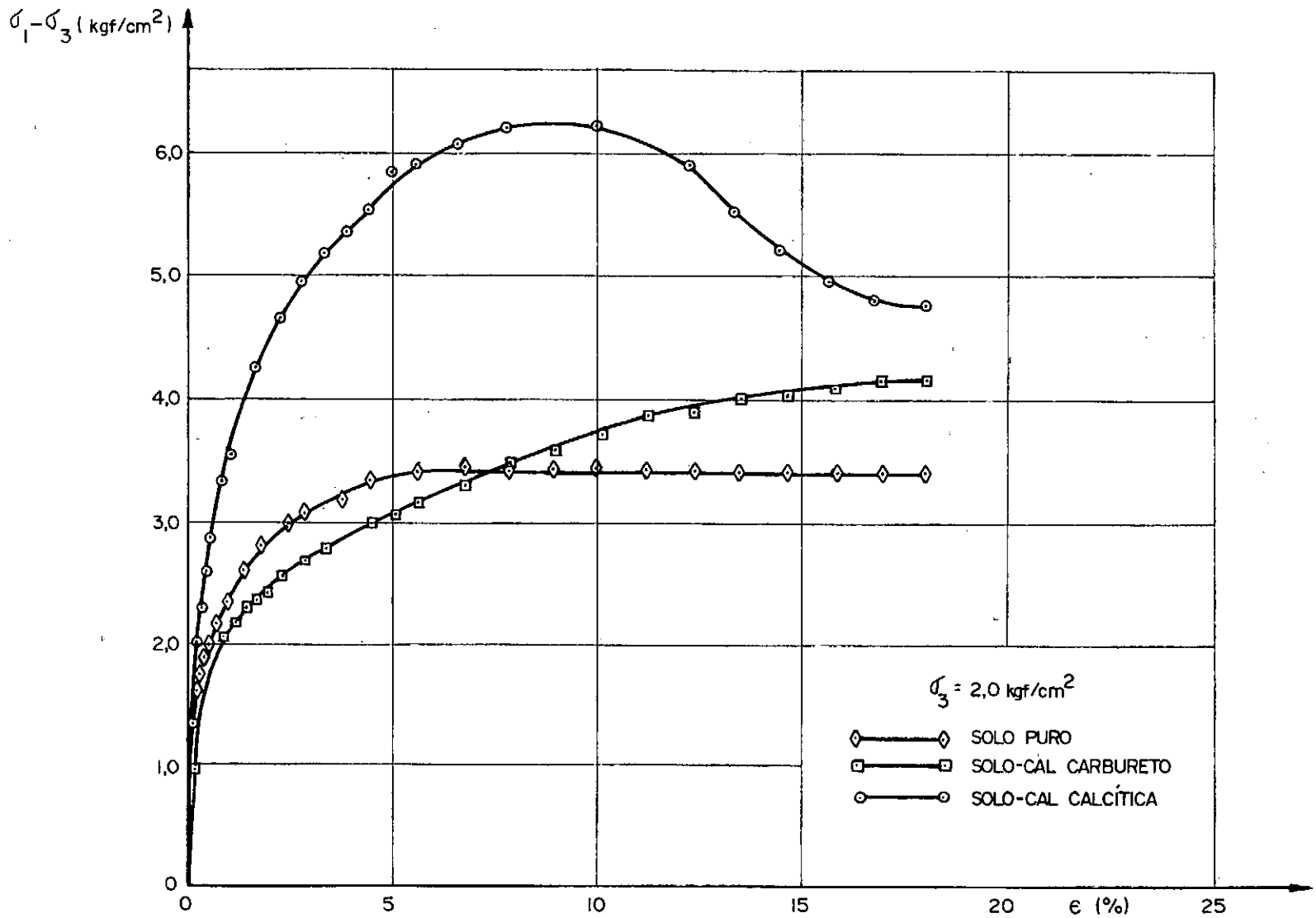
FIG.13.1 — Curvas tensão-deformação. Ensaio de compressão triaxial CU., para o solo puro, solo-cal de carbureto e solo-cal calcíca
