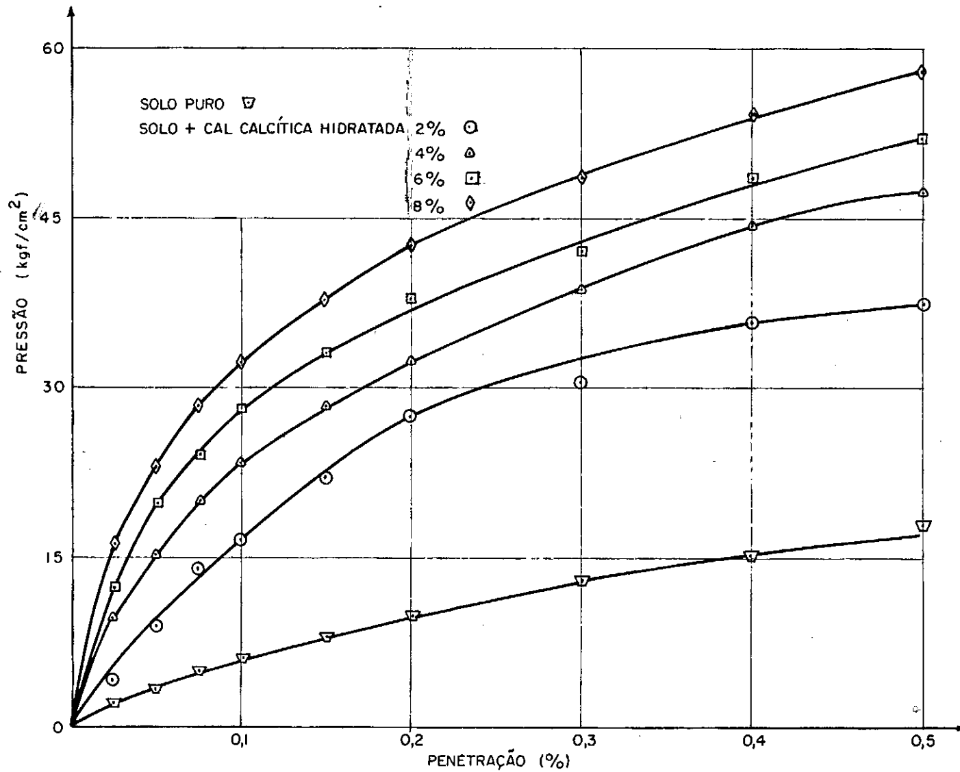
FIG. 11.2 — Curva de pressão versus penetração do solo puro e solo-cal calcíca hidratada
