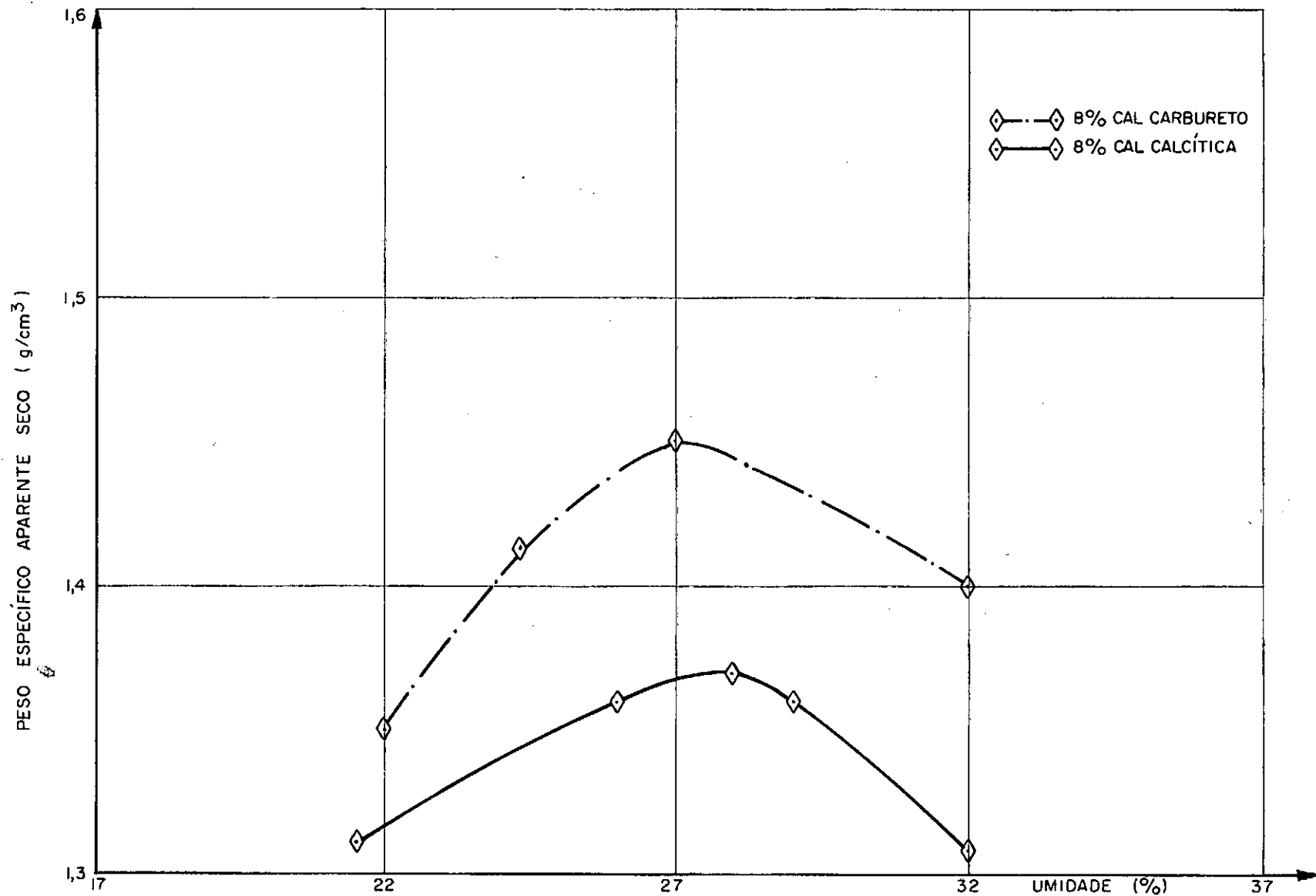
FIG. 10.6 — Relação entre o peso específico aparente seco e umidade de compactação para o solo-cal calcíca e solo-cal carbureto, ambos a 8%
