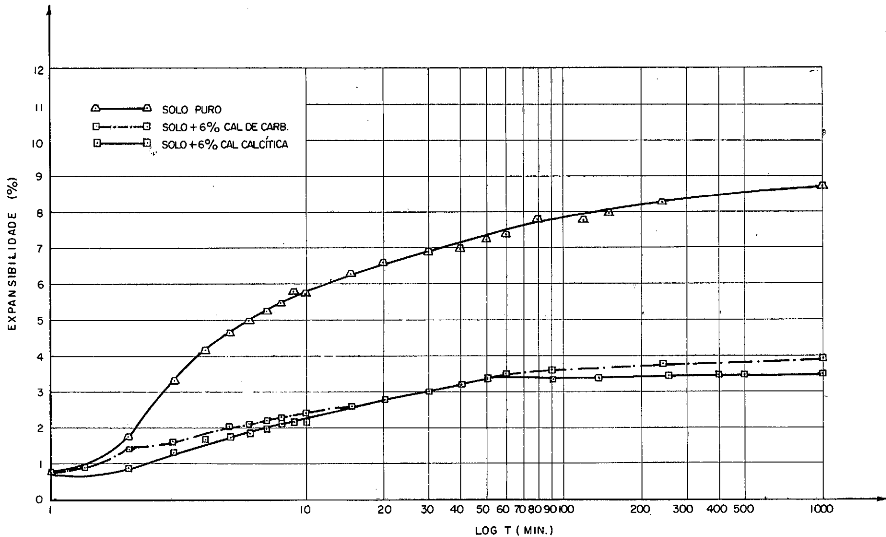
FIG.9.4 — Expansibilidade em função do tempo. Solo puro, solo-cal de carbureto e solo-cal calcífica, ambas a 6% .
