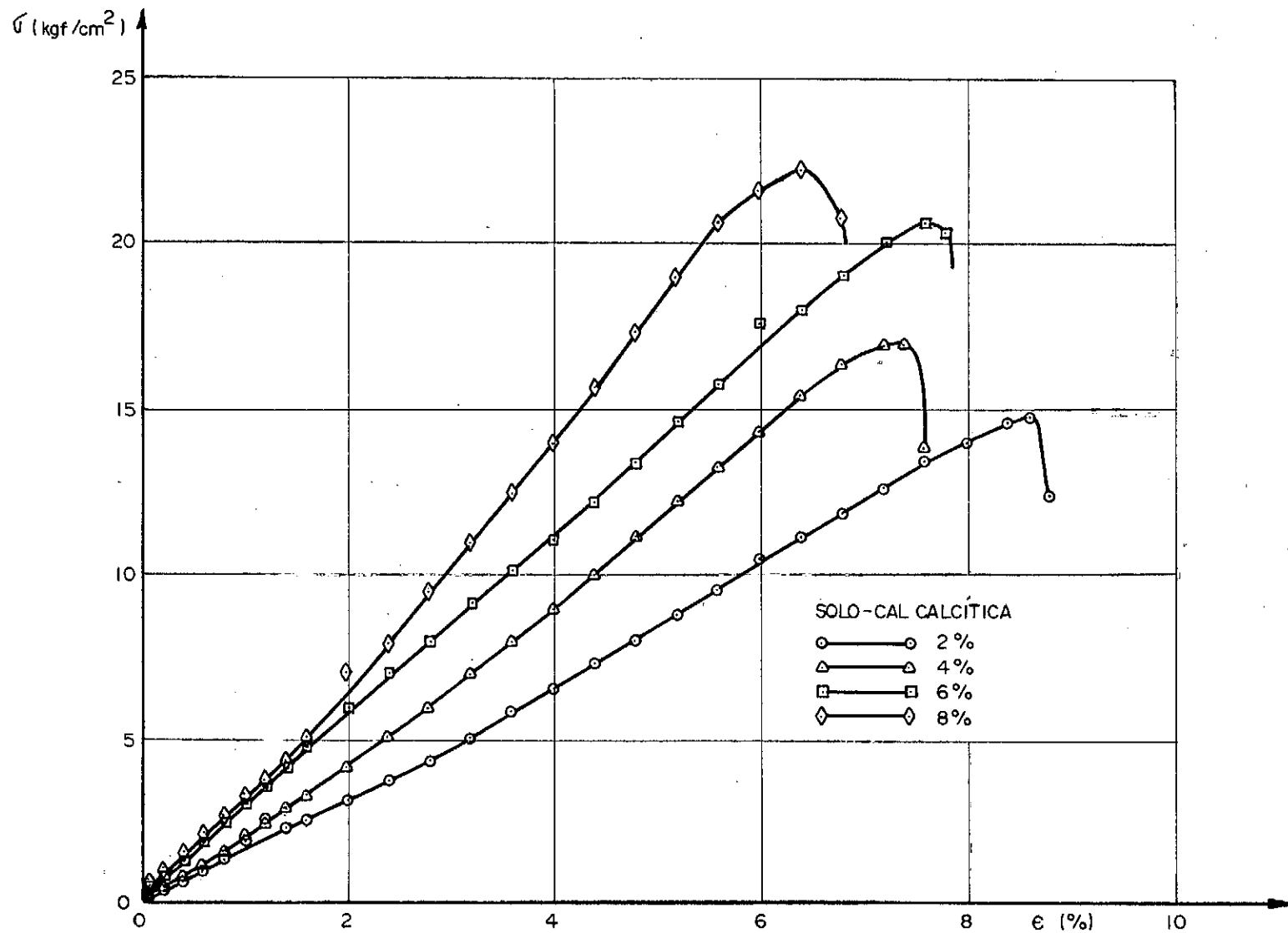
FIG.12.7 – Tensão versus deformação do solo-cal calcífica, no ensaio de resistência à compressão não confinada, a uma cura de 28 dias
