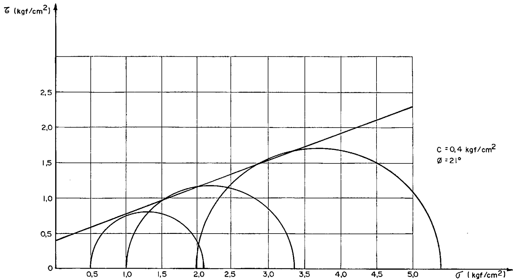
FIG. 13.5 — Envoltória de Mohr. Ensaio C.U. Pressões totais. Solo puro
