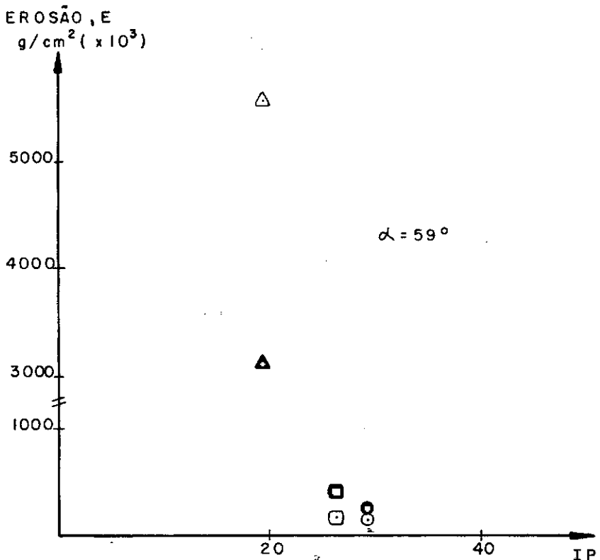
FIGURA: VII-5-EROSÃO x ÍNDICE DE PLASTICIDADE.
