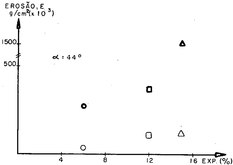
FIGURA VII-12-EROSÃO x EXPANSIBILIDADE (LNEC)
