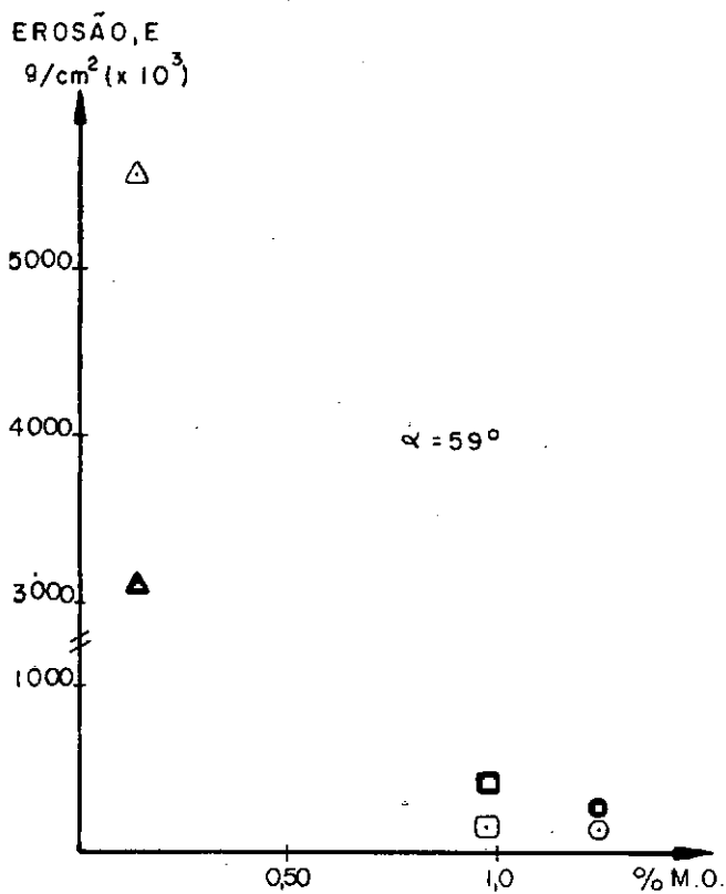
FIGURA: VII-11-EROSAÇÃO x % MATÉRIA ORGÂNICA NO SOLO.
