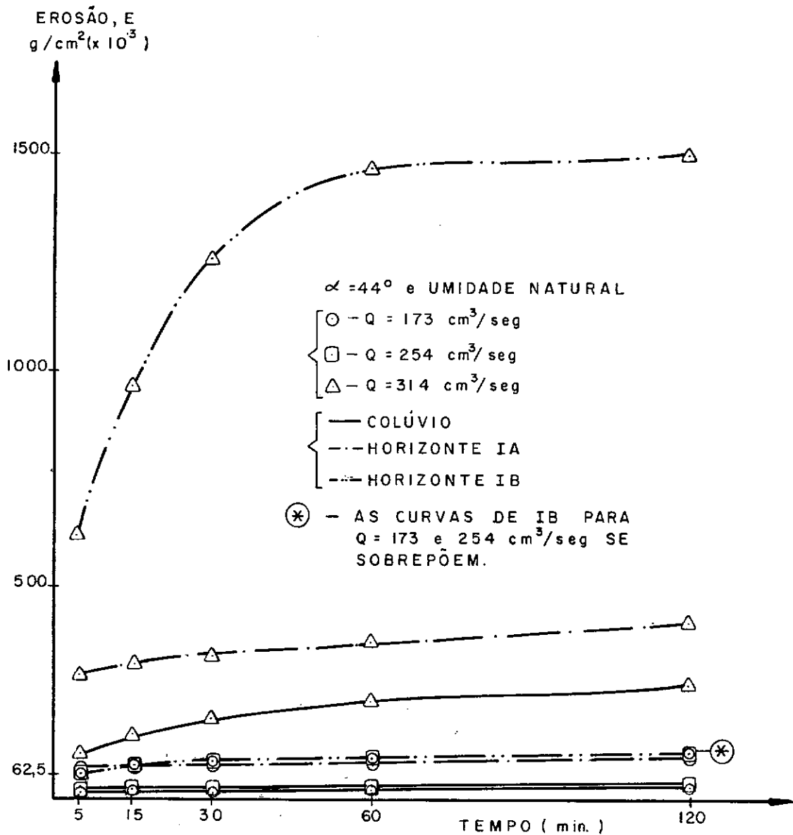
FIGURA :VI 5-EROSÃO x TEMPO - HORIZONTES :COLÚVIO IA e IB. INFLUÊNCIA DA VAZÃO NA EROSAO.
