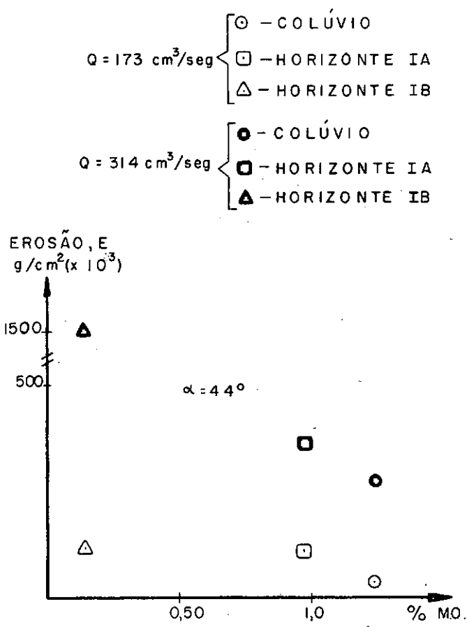
FIGURA: VII-10-EROSAÇÃO x % MATÉRIA ORGÂNICA NO SOLO.
