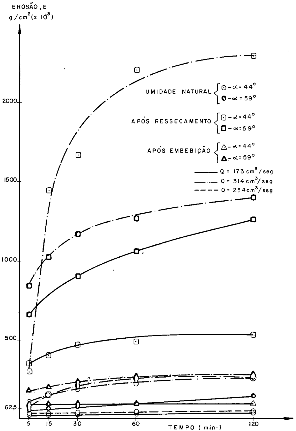
FIGURA : VI · 7 - EROSÃO x TEMPO - HORIZONTE : COLÚVIO
