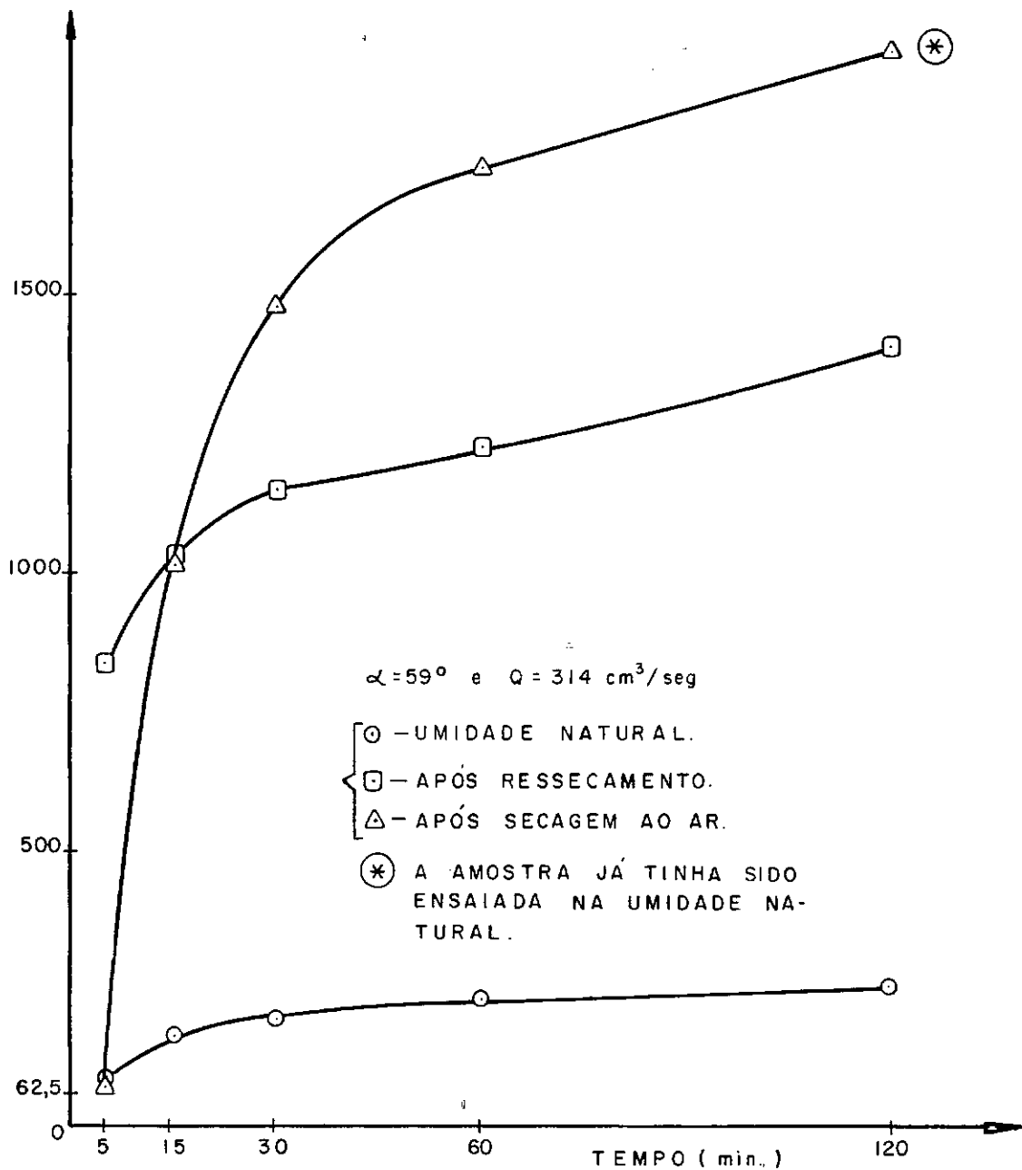
FIGURA: VI-14-EROSÃO x TEMPO - HORIZONTE : COLÚVIO. INFLUÊNCIA DO CICLO: ENSAIO-SECAGEM-ENSAIO.
