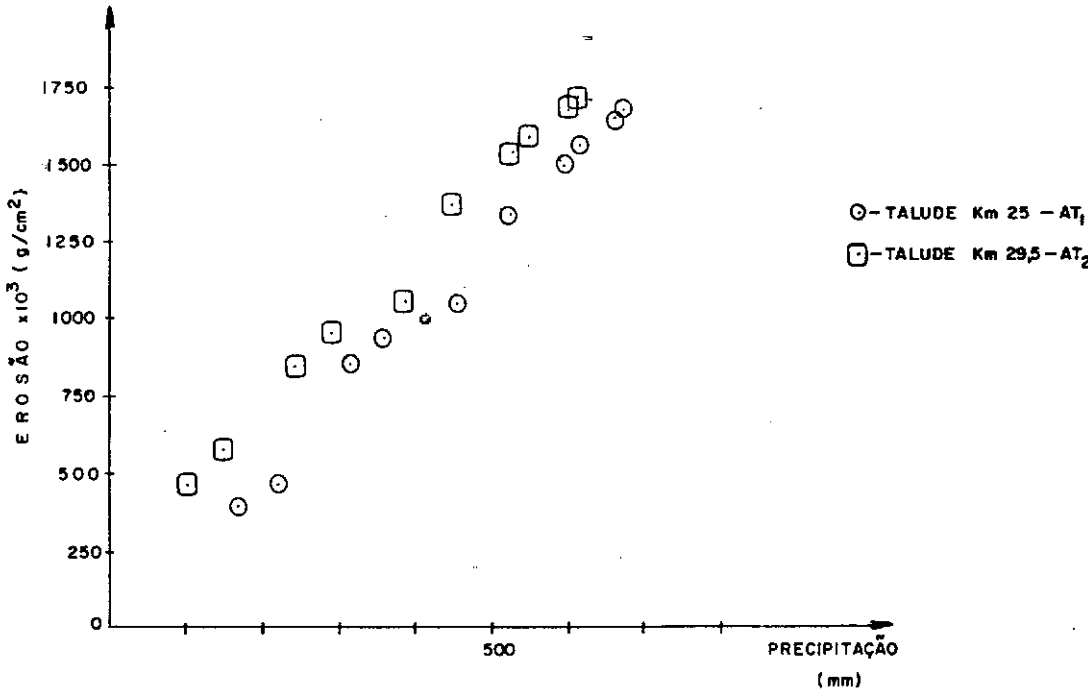
FIG. VIII. 3 - EROSÃO x PRECIPITAÇÃO (ACUMULADAS)
