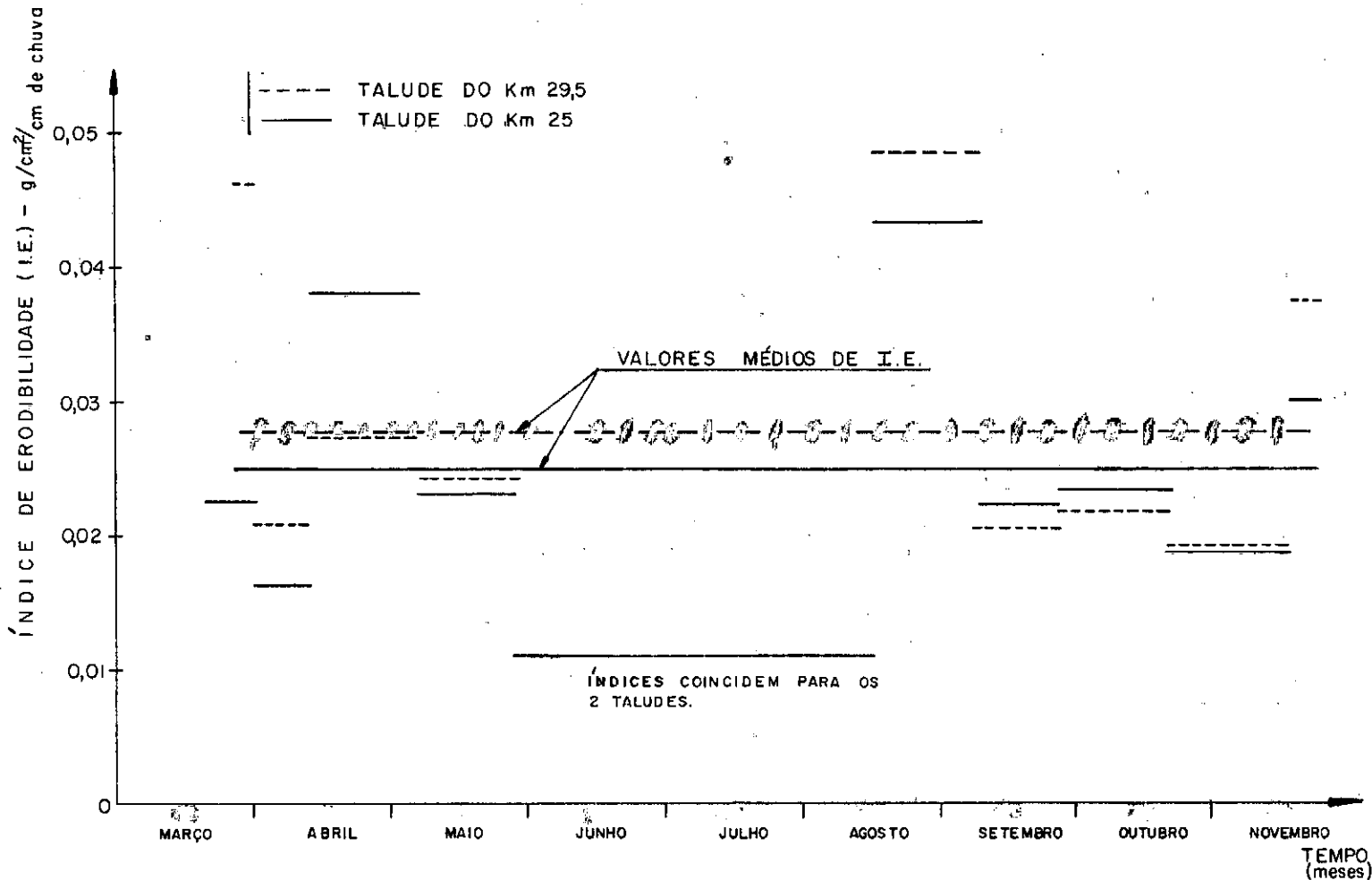
FIG. VIII.1 - ÍNDICE DE ERODIBILIDADE x TEMPO VARIACÃO DO I.E. ENTRE CADA PERÍODO DE OCORRÊNCIA.
