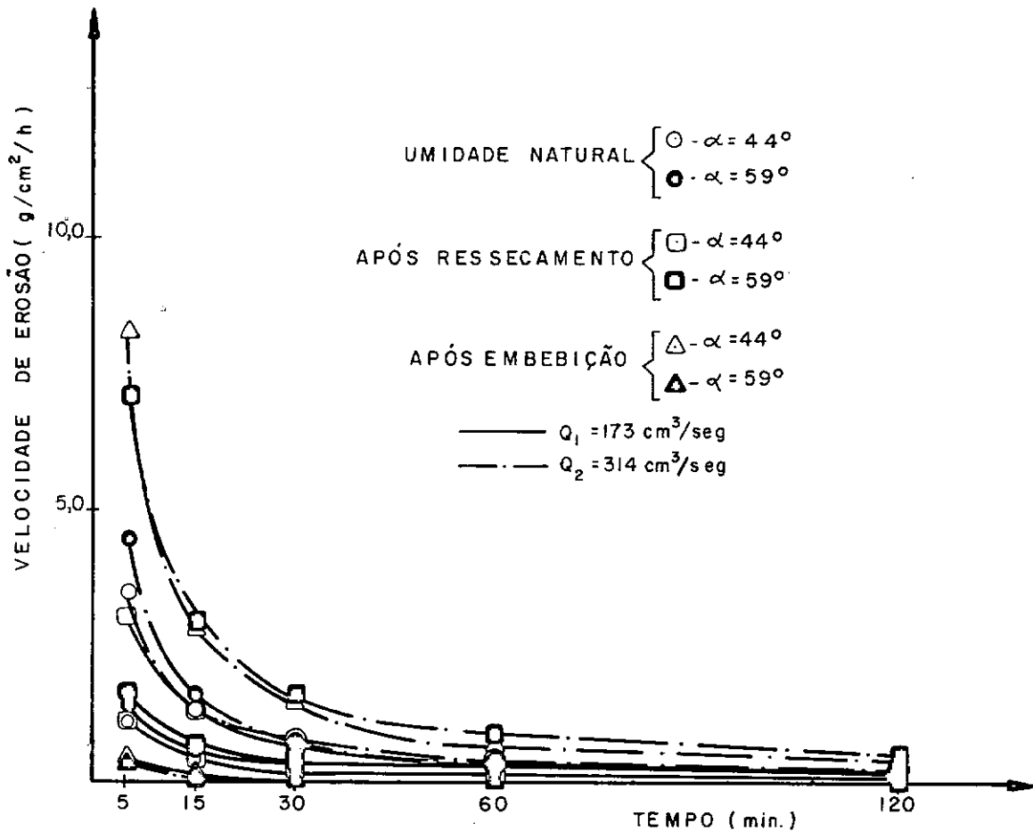
FIGURA: VI · II - VELOCIDADE DE EROÇÃO x TEMPO. HORIZONTE IA
