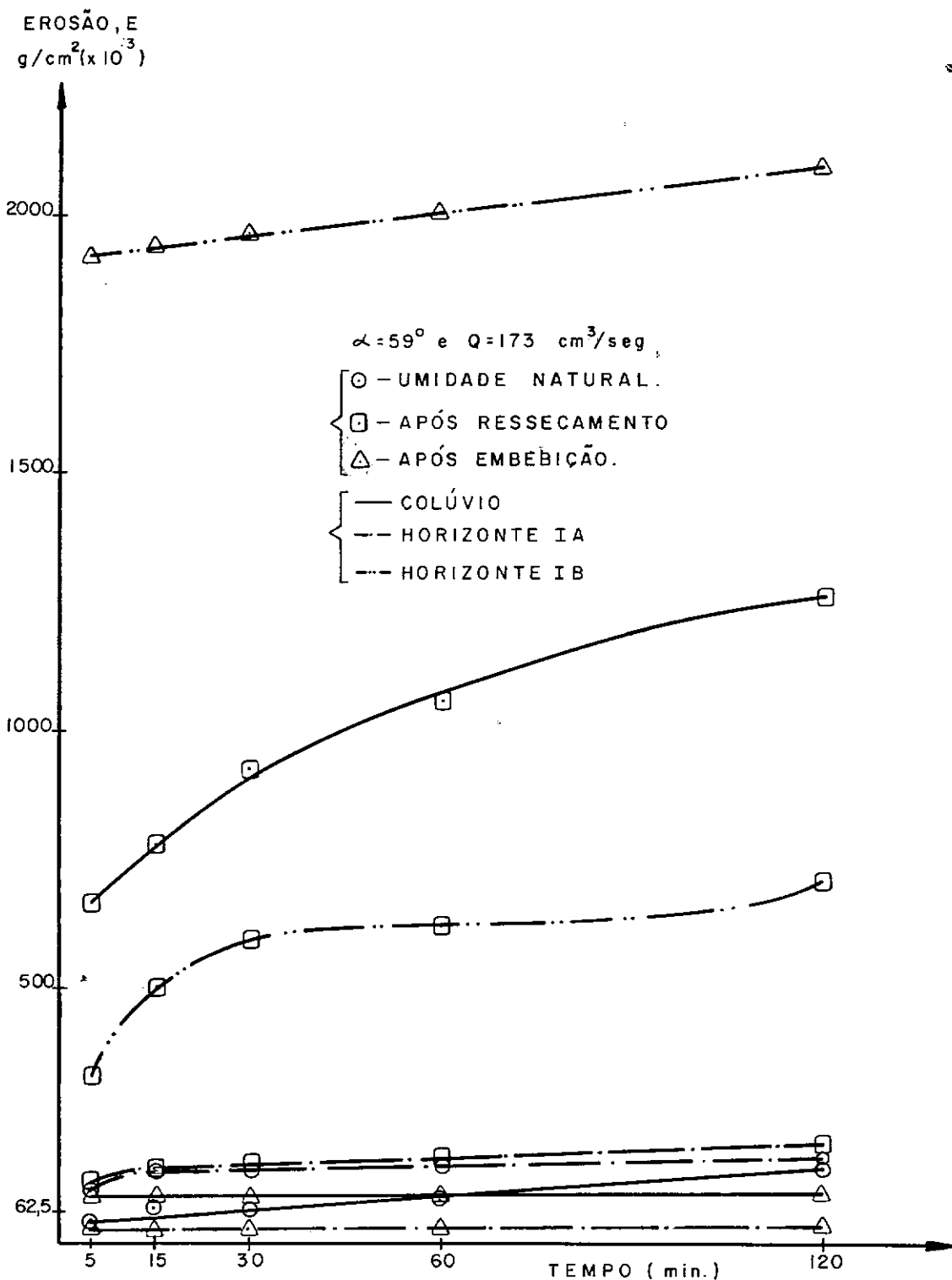
FIGURA : VI-3-EROSÃO x TEMPO - HORIZONTES : COLÚVIO IA e IB INFLUÊNCIA DAS CONDIÇÕES DE UMIDADE DAS AMOSTRAS NA EROSÃO.
