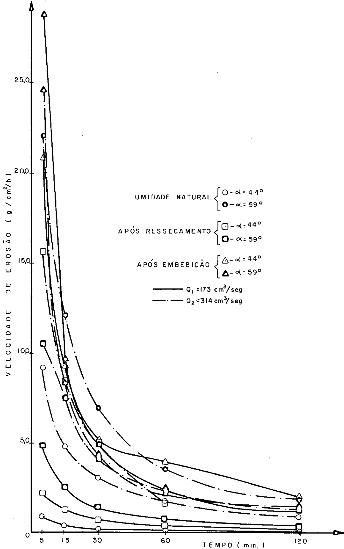
FIGURA : VI · 12-VELOCIDADE DE EROSÃO x TEMPO-HORIZONTE IB.
