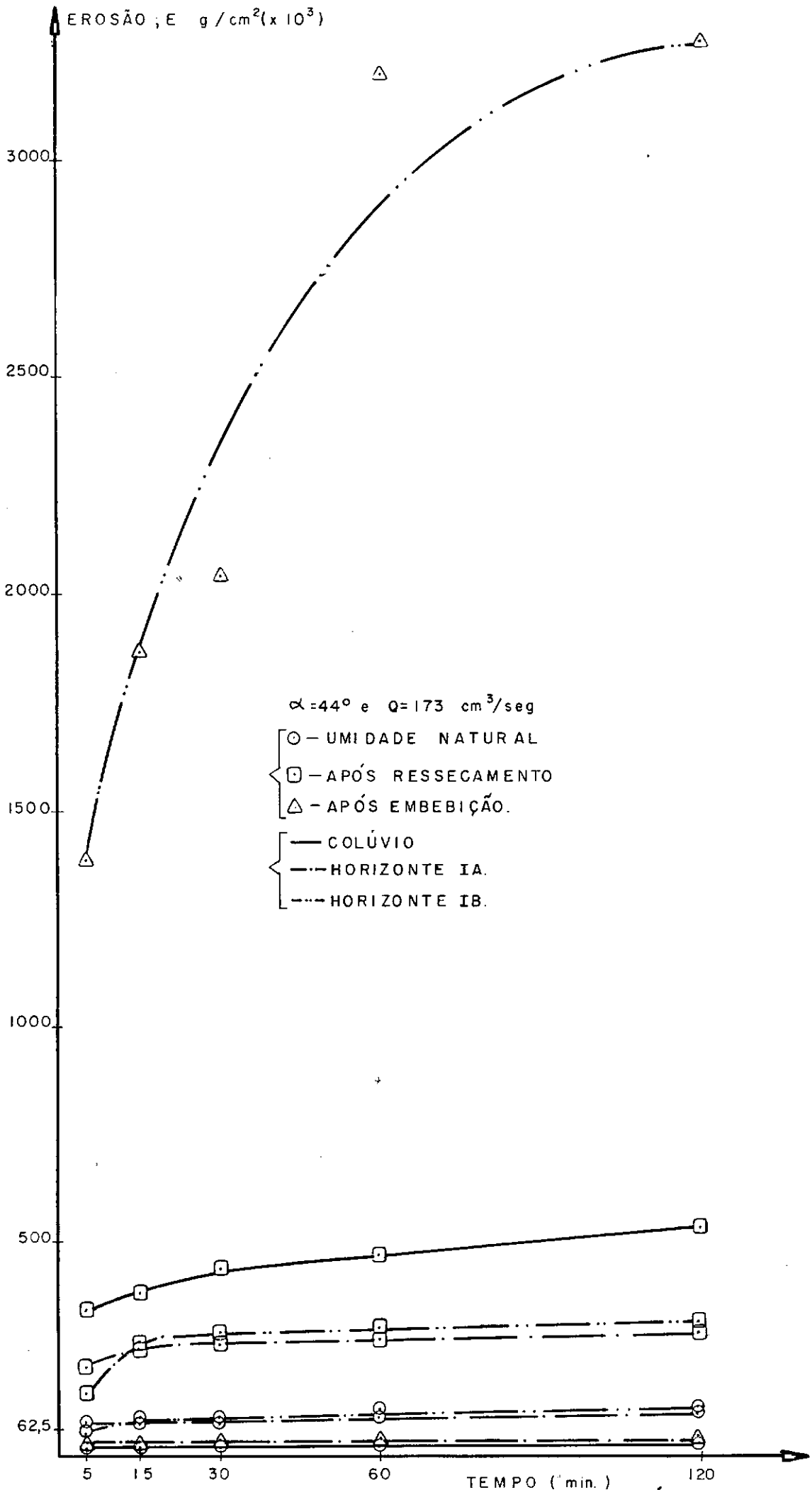
FIGURA : VI.1 - EROSIÃO x TEMPO - HORIZONTES: COLÚVIO IA e IB INFLUÊNCIA DAS CONDIÇÕES DE UMIDADE DAS AMOSTRAS NA EROSIÃO.
