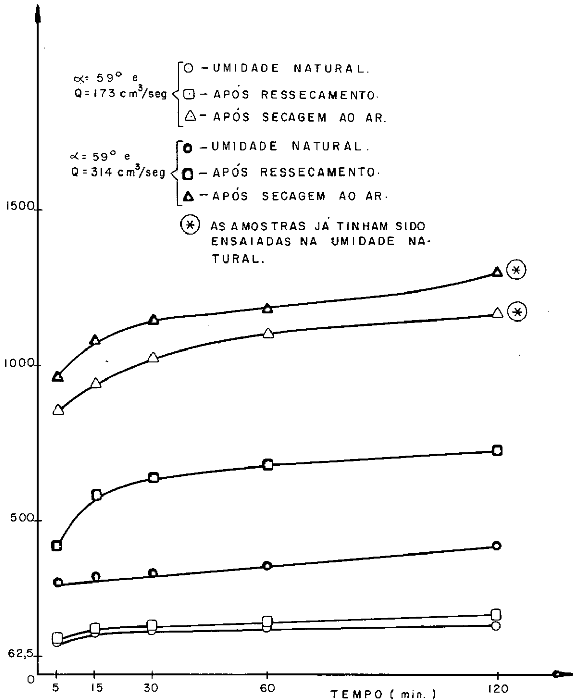
FIGURA: VI-15-EROSÃO x TEMPO - HORIZONTE IA. INFLUÊNCIA DO CICLO: ENSAIO-SECAGEM-ENSAIO.
