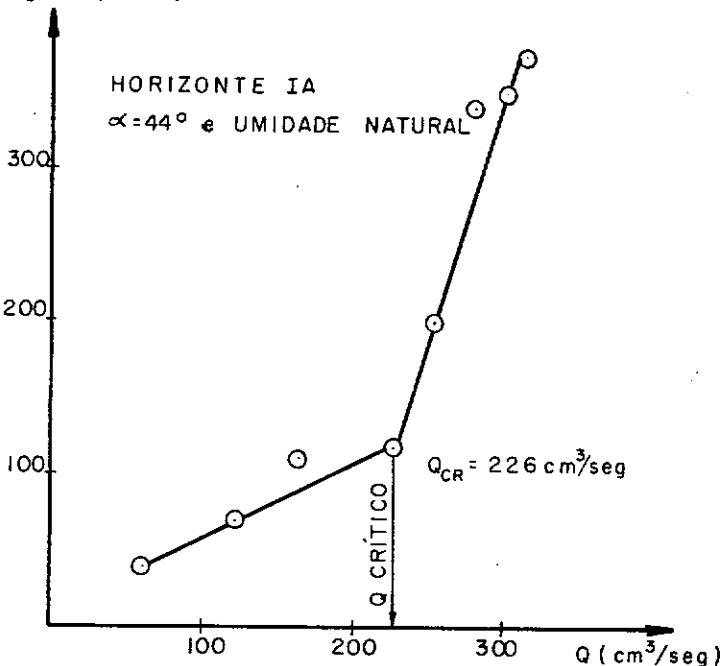
FIGURA: VI-17-EROSÃO x VAZÃO DE ENSAIO. DETERMINAÇÃO DA VAZÃO CRÍTICA.
