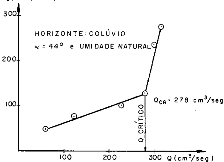
FIGURA: VI-16-EROSÃO x VAZÃO DE ENSAIO. DETERMINAÇÃO DA VAZÃO CRÍTICA.
