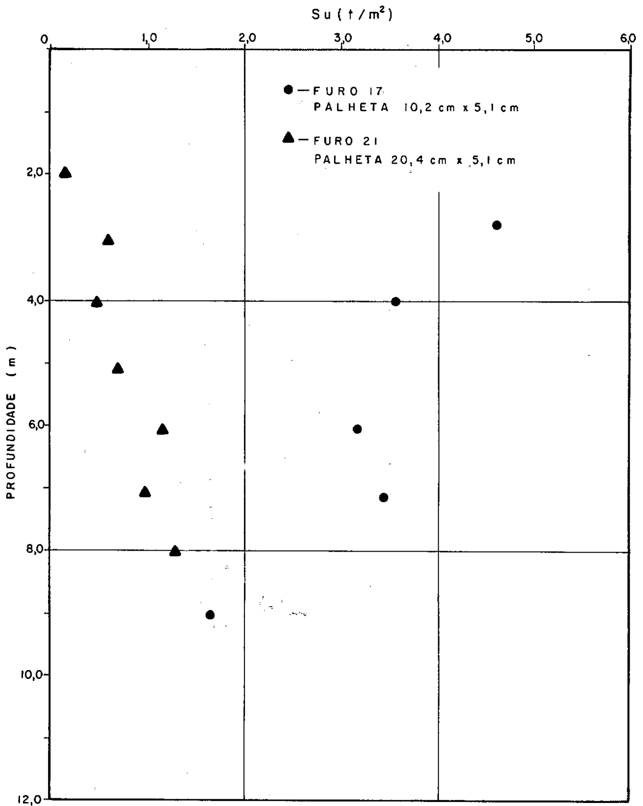
FIGURA 8.3 — VARIAÇÃO DA RESISTÊNCIA NÃO DRENADA COM A PROFUNDIDADE EM ENSAIOS EXPERIMENTAIS. ( ARGILA INDEFORMADA. ) LOCAL: SARAPUÍ
