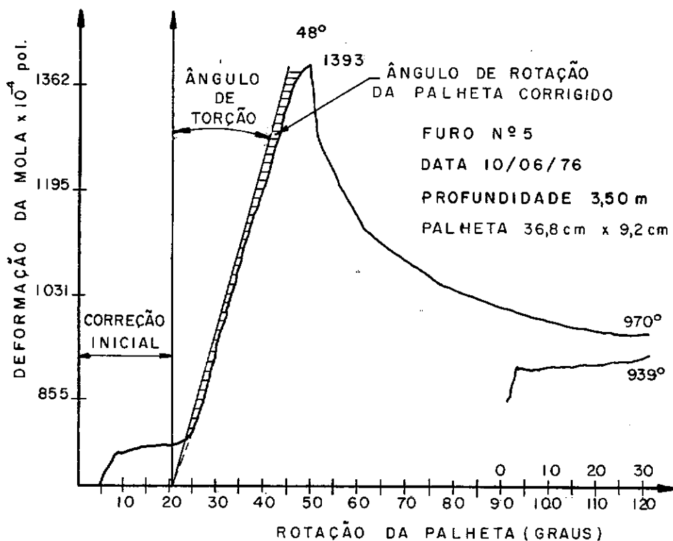
FIGURA 6.3 - CURVAS DEFORMAÇÃO DA MOLA \times ÂNGULO DE ROTAÇÃO DA PALHETA (NÃO CORRIGIDO). LOCAL: MAGÉ
