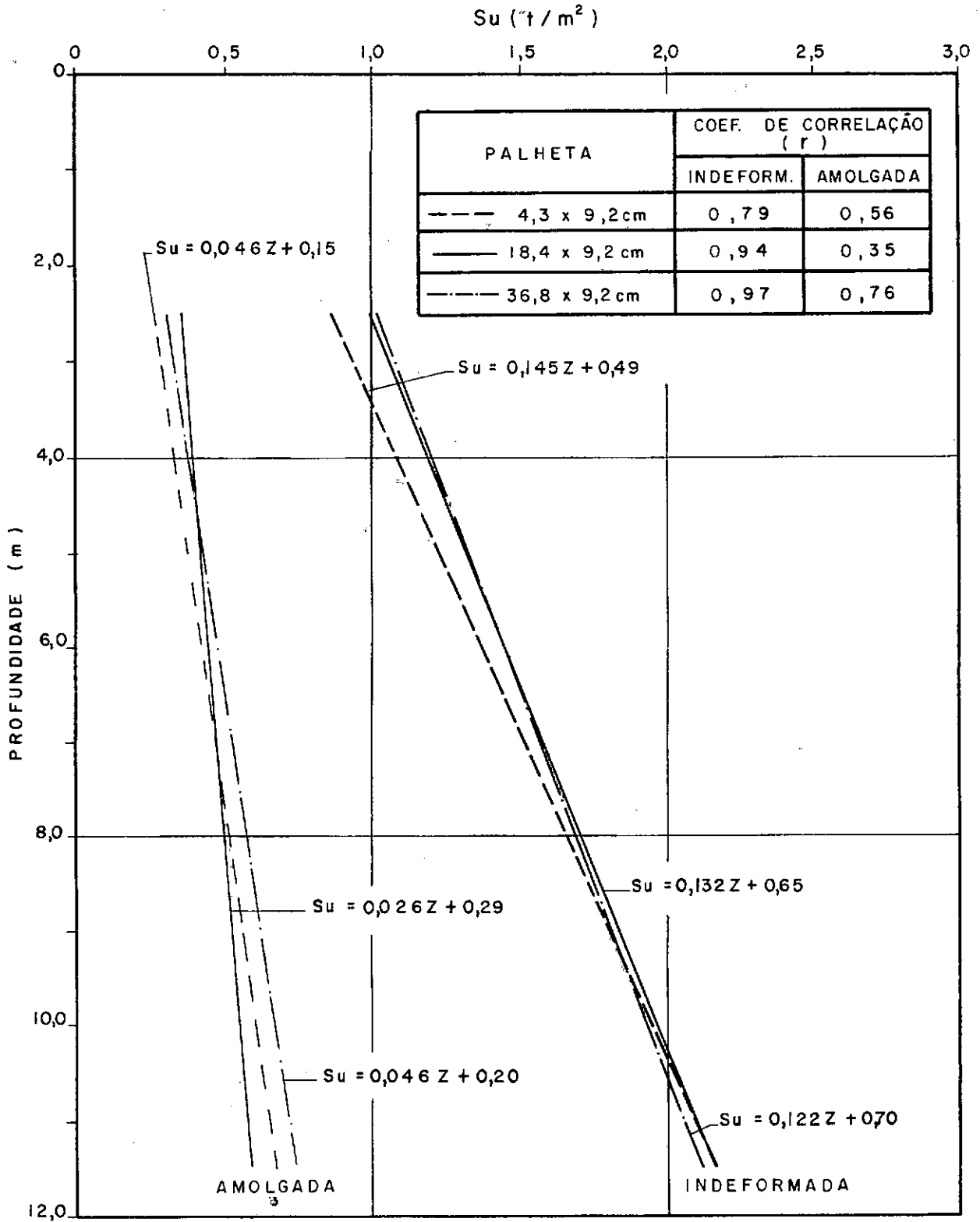
FIGURA 6-19— VARIAÇÃO DA RESISTÊNCIA NÃO DRENADA COM A PROFUNDIDADE. RETAS OBTIDAS POR REGRESSÃO. LOCAL: MAGÉ
