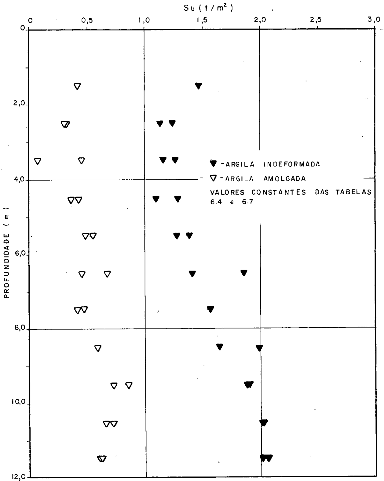
FIGURA 6.18 - VARIAÇÃO DA RESISTÊNCIA NÃO DRENADA 28 COM A PROFUNDIDADE.
