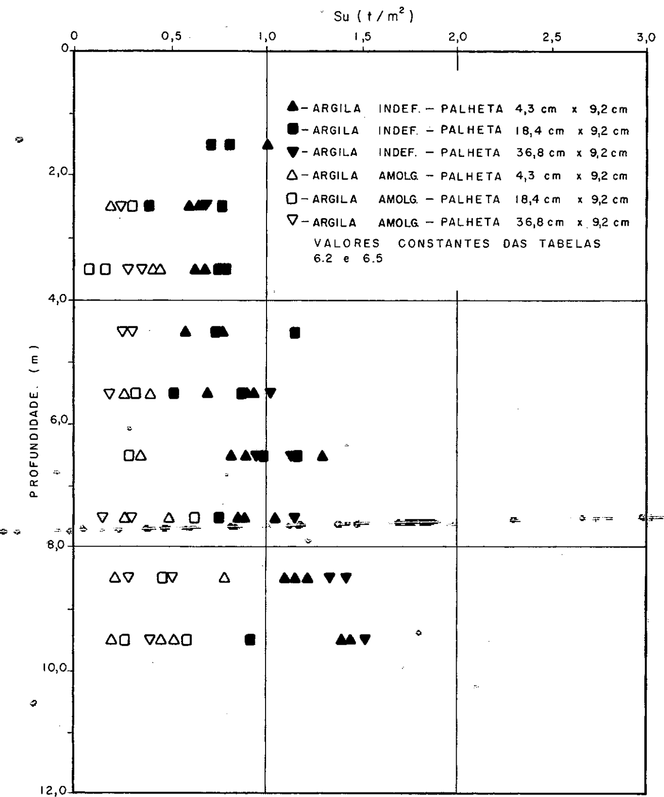
FIGURA 6-8- VARIAÇÃO DA RESISTÊNCIA NÃO DRENADA COM A PROFUNDIDADE.
