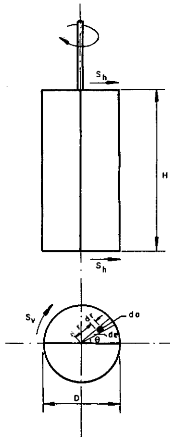
FIGURA 3-7- DESENVOLVIMENTO DA RESISTÊNCIA NÃO DRENADA.
