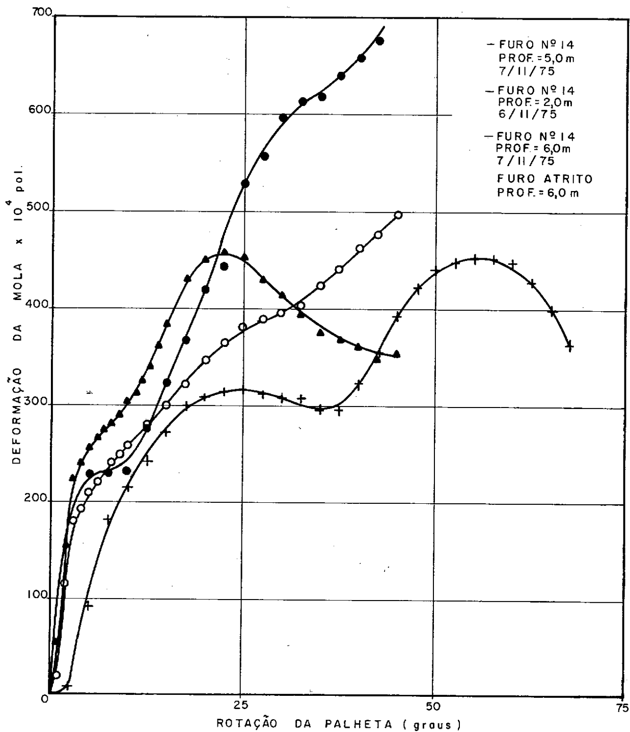
FIGURA 5.8- CURVAS DEFORMAÇÃO DA MOLA \times ÂNGULO DE ROTAÇÃO DA PALHETA LOCAL: SARAPUI
