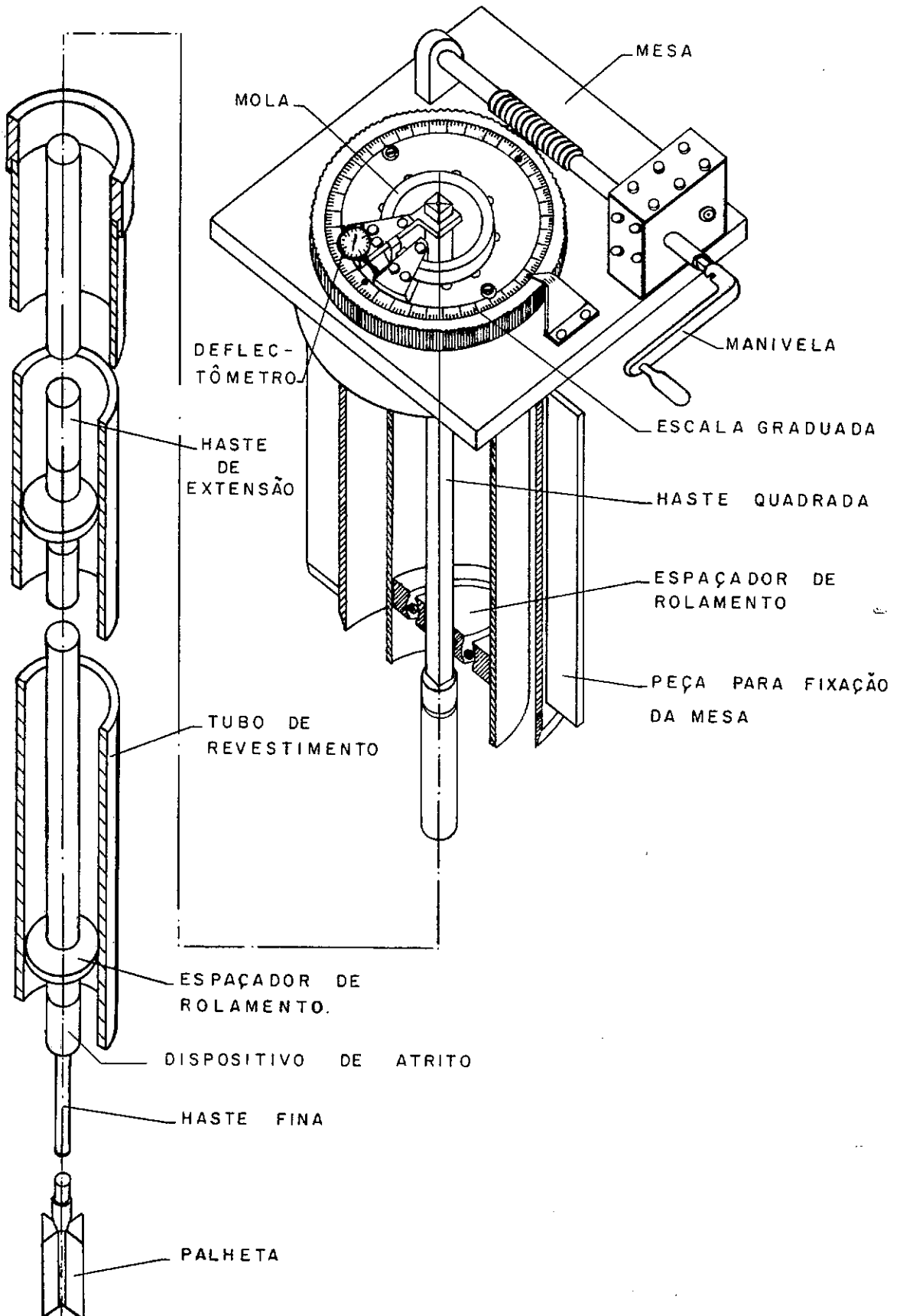
FIGURA 5-4 - COMPONENTES DO EQUIPAMENTO UTILIZADO NOS ENSAIOS.
