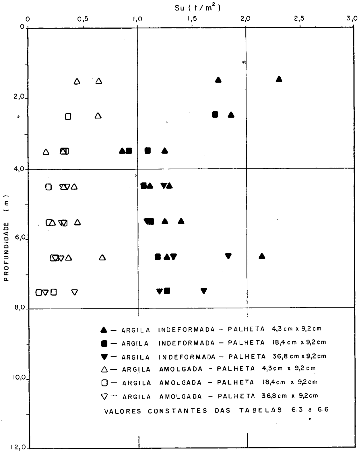
FIGURA 9 6-14- VARIAÇÃO DA RESISTÊNCIA NÃO DRENADA COM A PROFUNDIDADE. VALORES OBTIDOS CONSIDERANDO-SE TODOS OS ENSAIOS. LOCAL: ALCÂNTARA .
