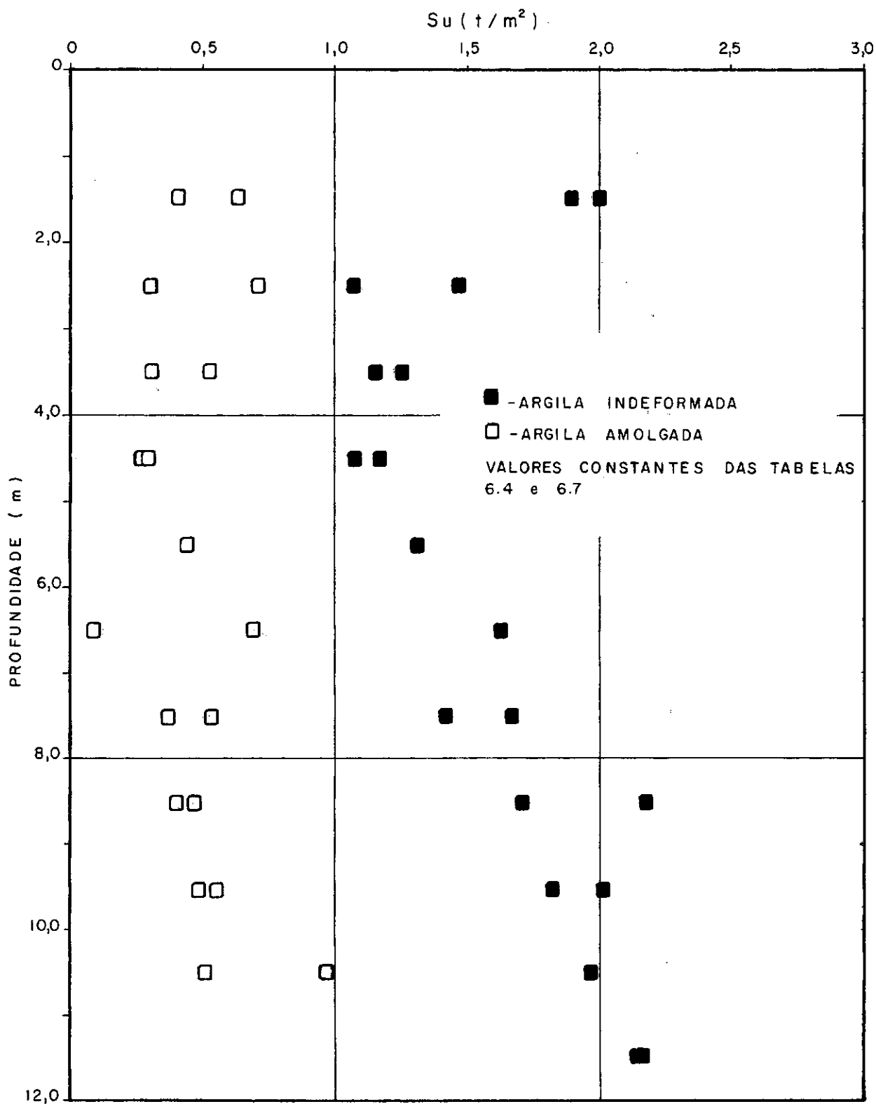
FIGURA 6.17 - VARIAÇÃO DA RESISTÊNCIA NÃO DRENADA COM A PROFUNDIDADE.
