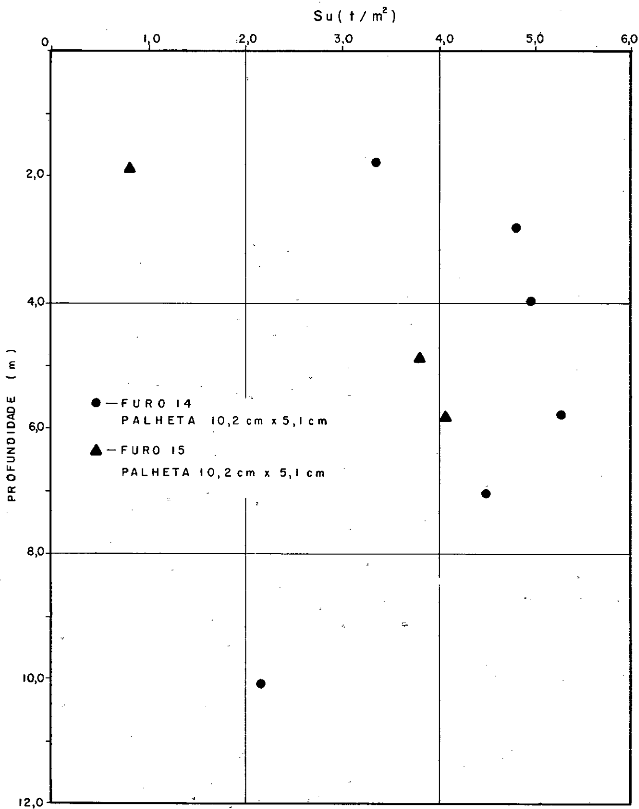
FIGURA 8-2 - VARIAÇÃO DA RESISTÊNCIA NÃO DRENADA COM A PROFUNDIDADE EM ENSAIOS EXPERIMENTAIS. ( ARGILA INDEFORMADA.) LOCAL: SARAPUI
