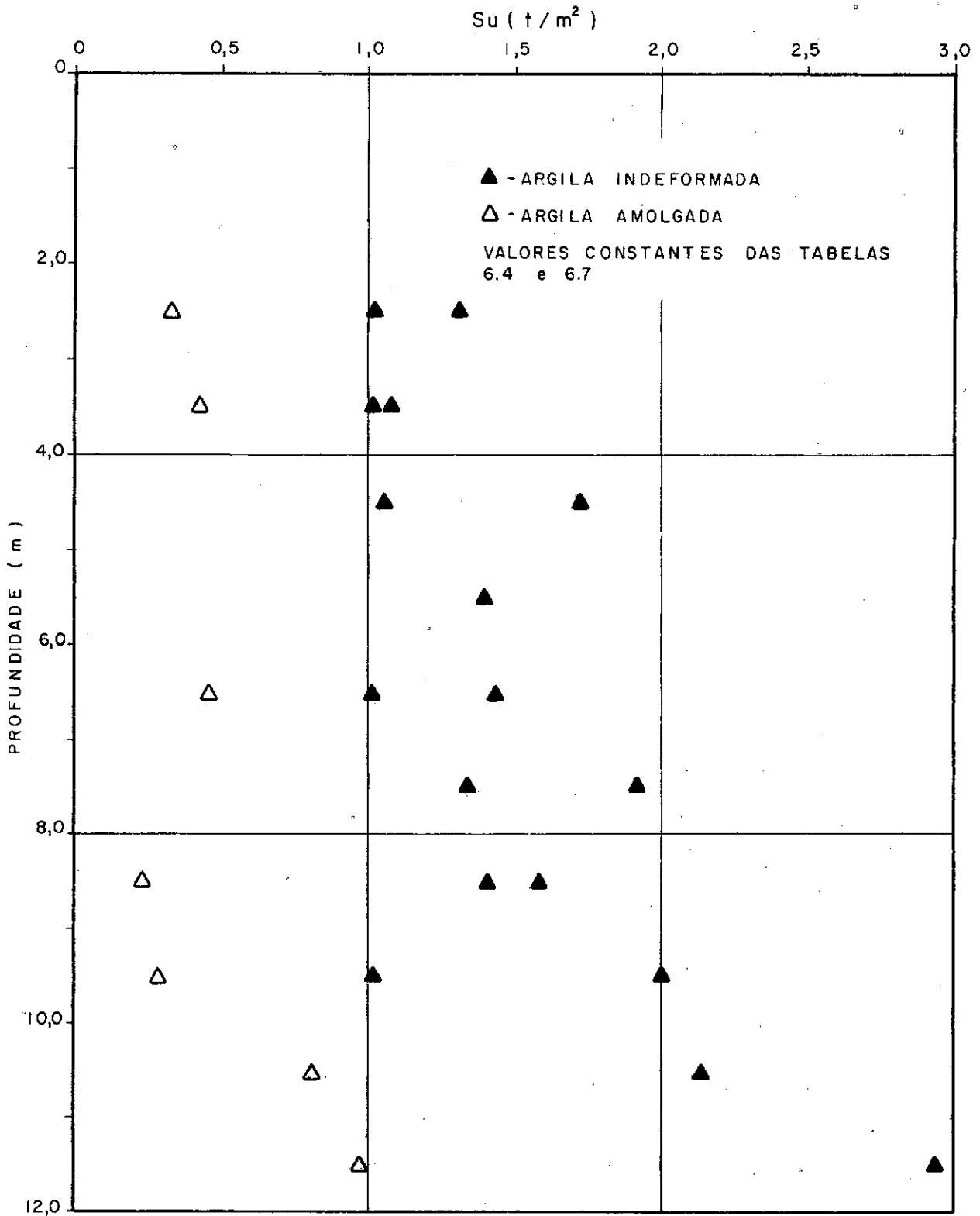
FIGURA 6-16 - VARIAÇÃO DA RESISTÊNCIA NÃO DRENADA COM A PROFUNDIDADE.
