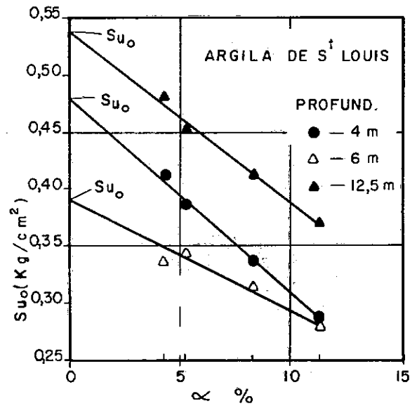
FIGURA 3-3 - RESISTÊNCIA S_{u0} , PARA PALHETA DE ESPESSURA NULA (LA ROCHELLE, ROY e TAVENAS -1973.)
