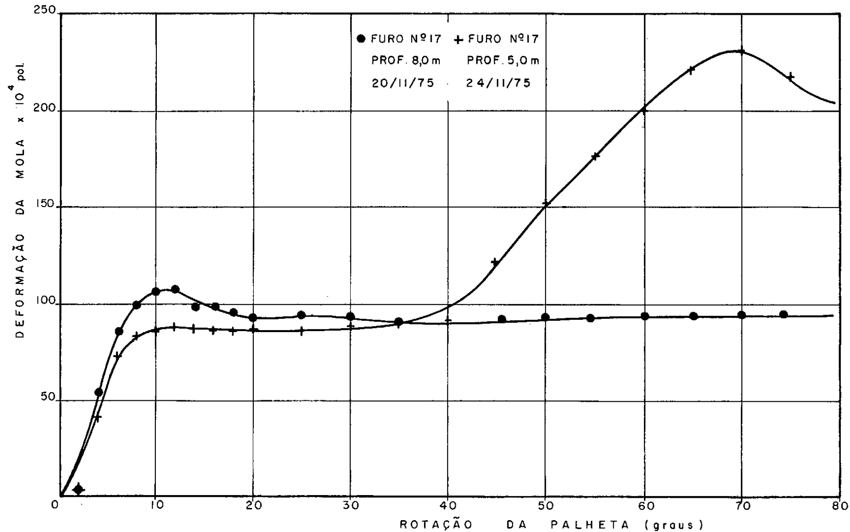
FIGURA 5-10- CURVAS DEFORMAÇÃO DA MOLA \times ÂNGULO DE ROTAÇÃO DA PALHETA. LOCAL: SARAPUI
