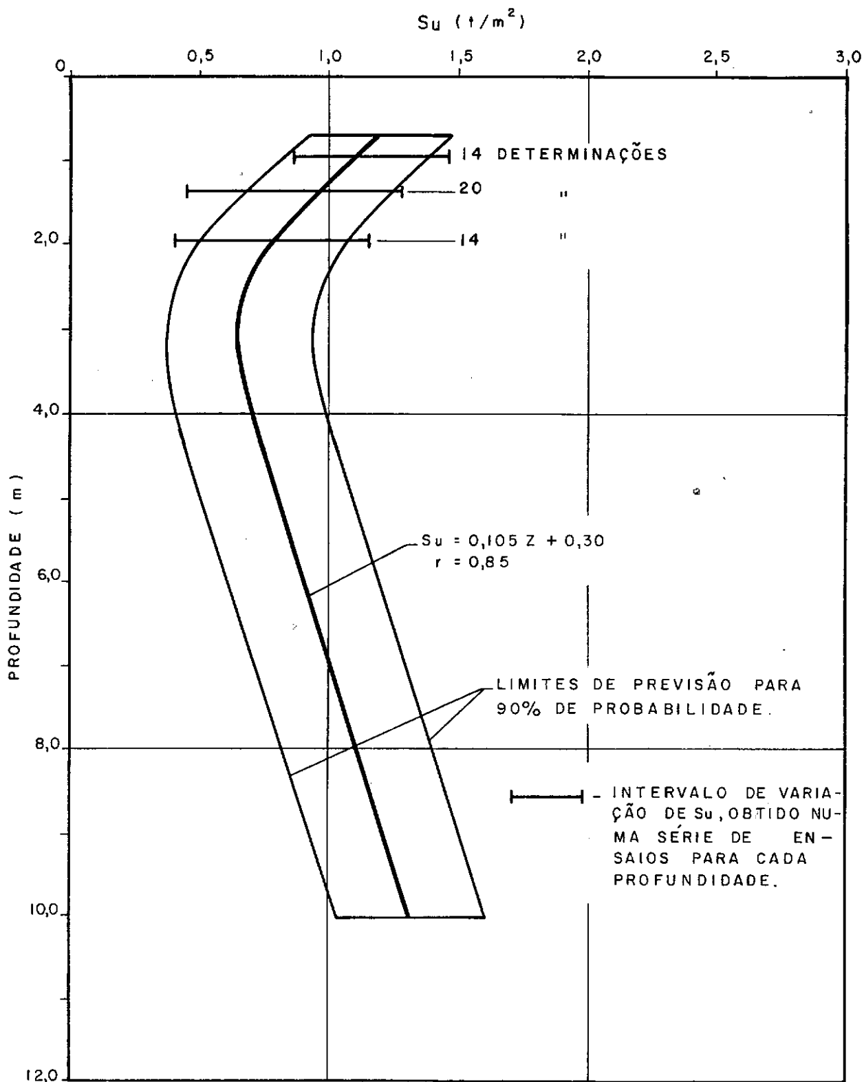
FIGURA 6-9 - VARIAÇÃO DA RESISTÊNCIA NÃO DRENADA COM A PROFUNDIDADE.
