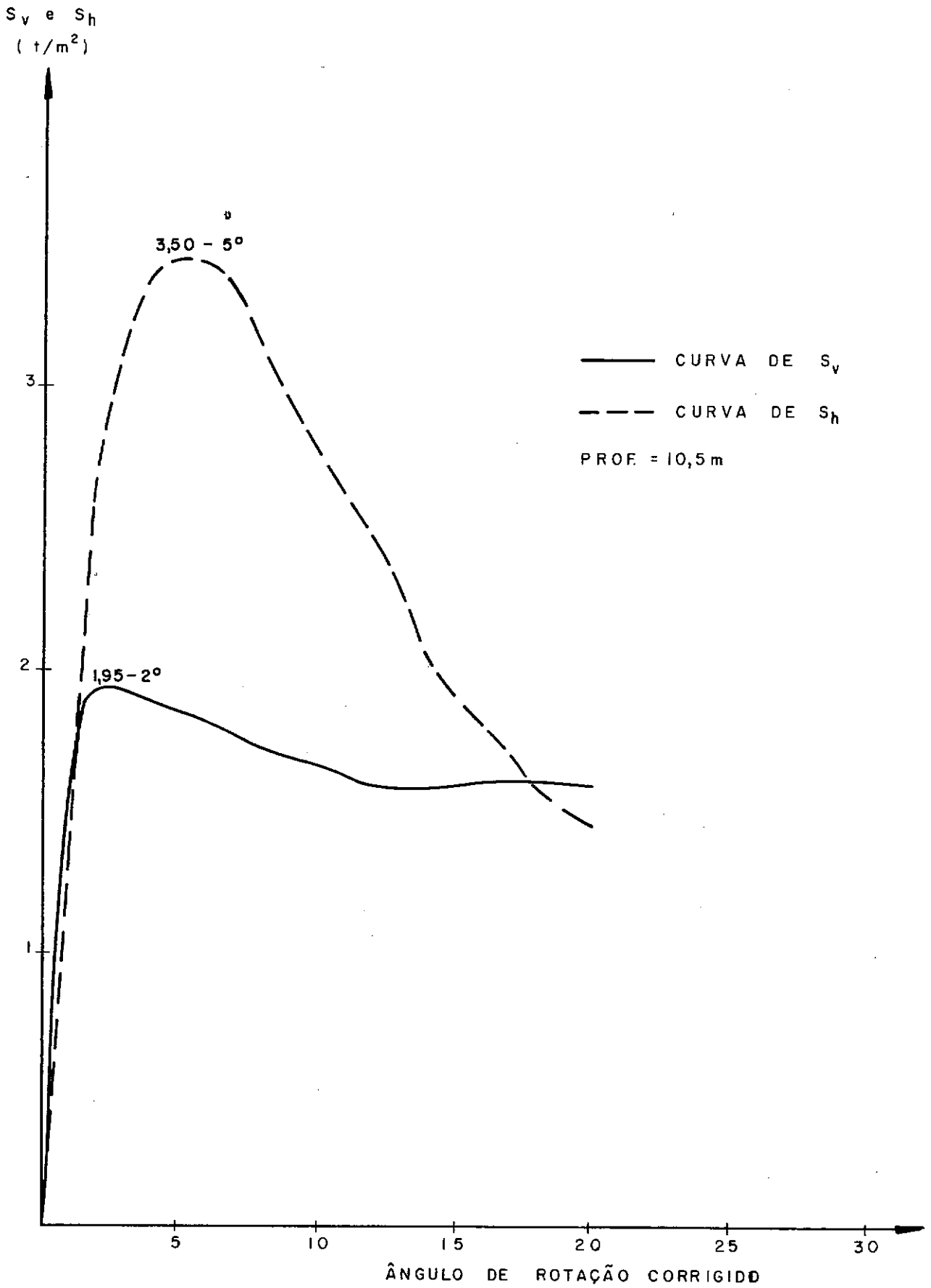
FIGURA 7.17 — CURVAS S_v e S_h x ÂNGULO DE ROTAÇÃO CORRIGIDO. LOCAL: MAGÉ
