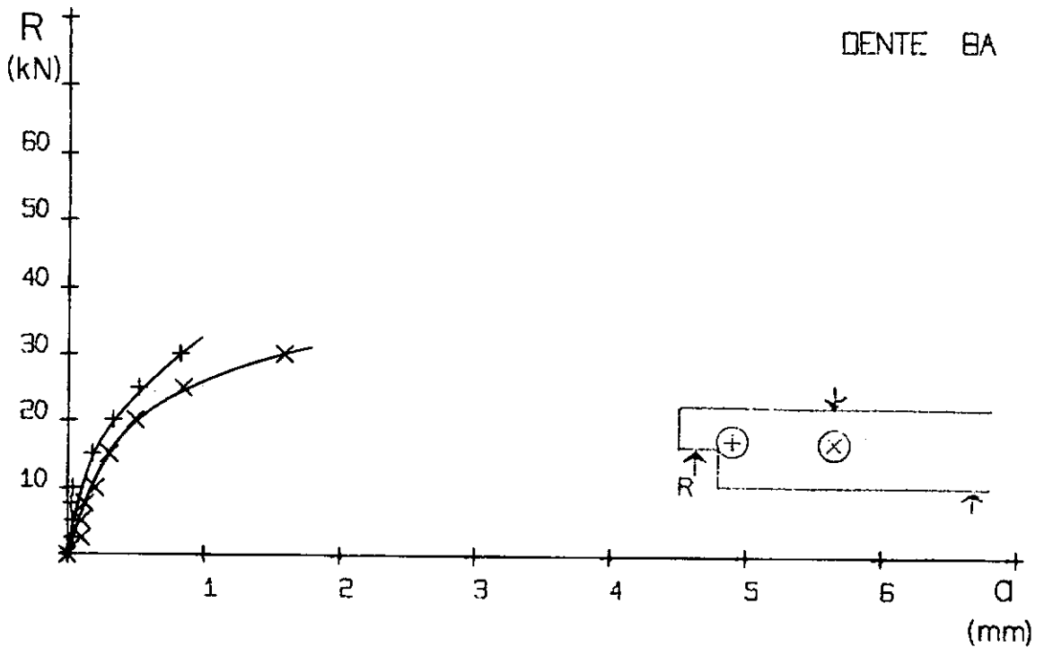
Fig. 40 e 41 - Gráficos reação de apoio - flecha nos pontos 2 e 3.
