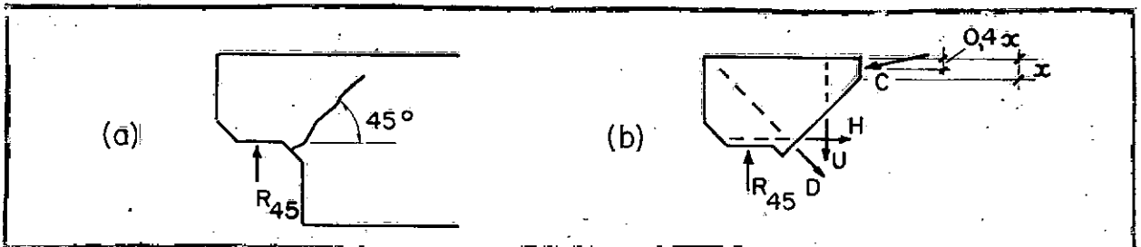
Fig. 2 - (a) Configuração de ruptura; (b) Forças no dente.
