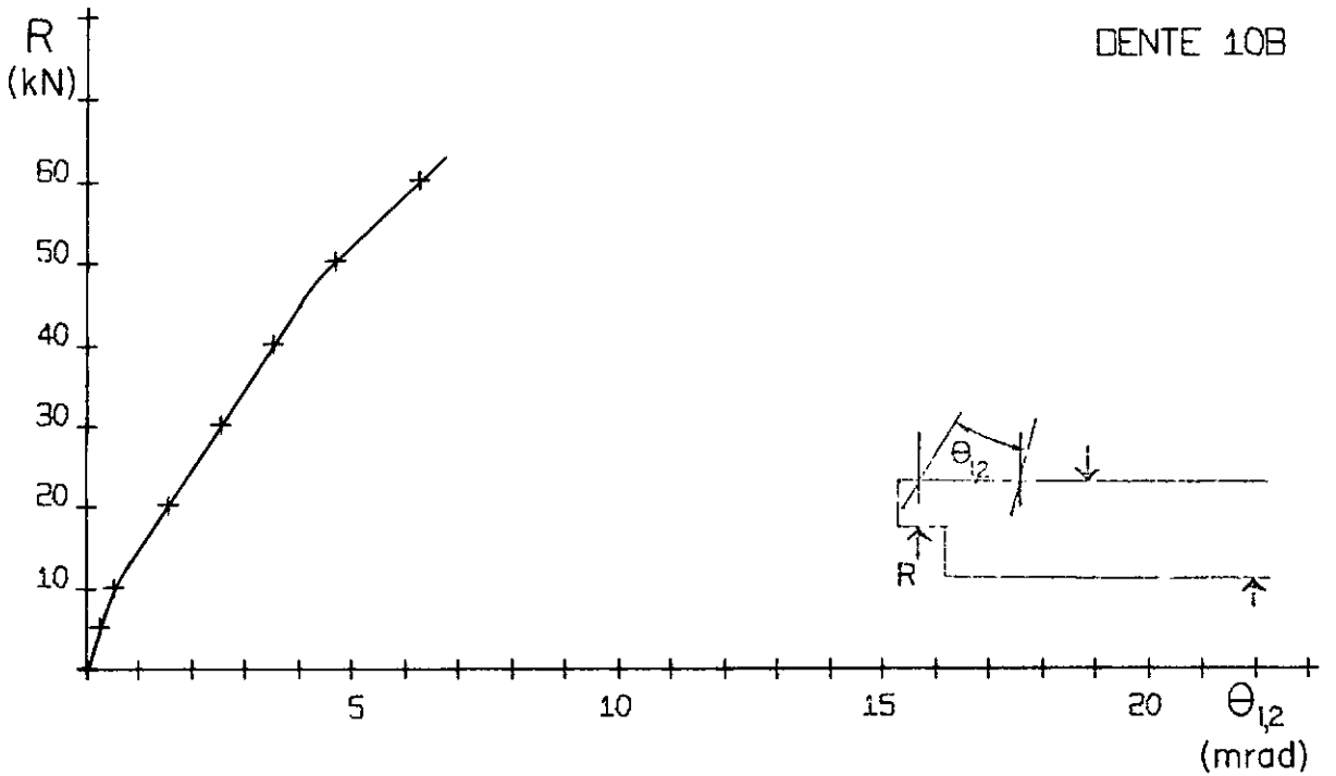
Fig. 72 e 73 - Gráficos reação de apoio - rotação relativa das seções 1 e 2.
