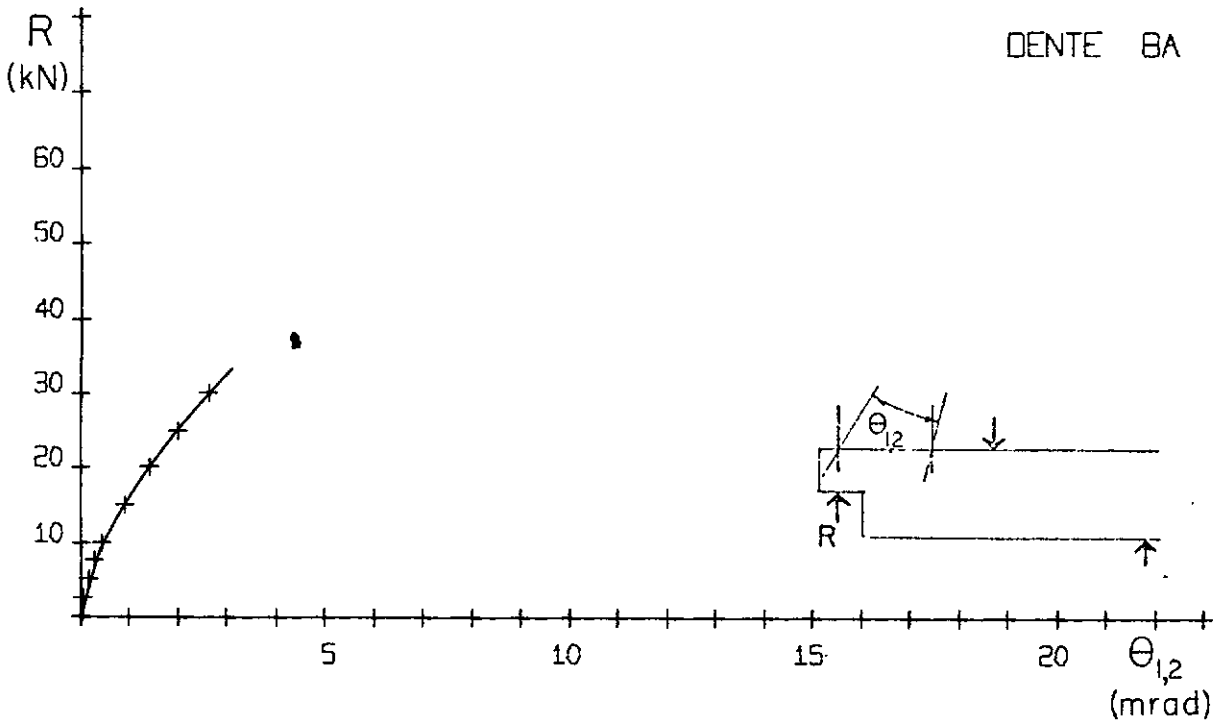
Fig.60 e 61 - Gráficos reação de apoio - rotação relativa das seções 1 e 2.
