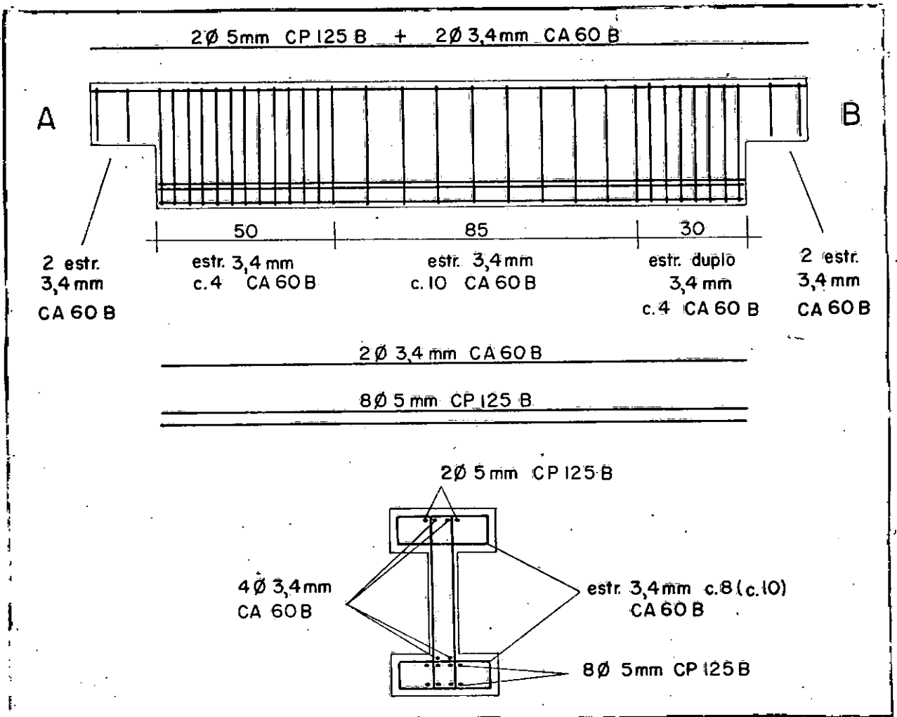
Fig. 10 - Armadura das vigas.
