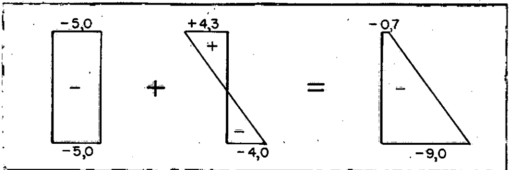
Fig. 9 - Tensões no concreto devidas à protensão.
