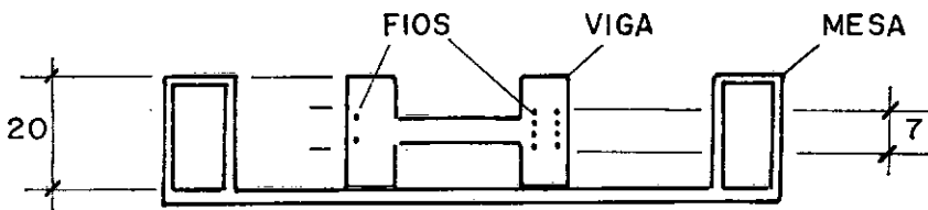
Fig. 21 - Seção transversal da mesa de protensão.
