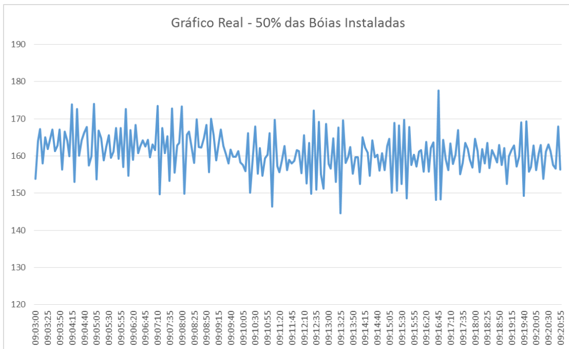
Figura 5.4-1 – Gráfico Real 50% das bóias instaladas
