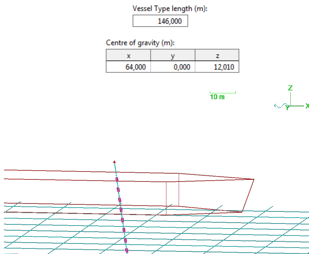
Figura 4.5-4 – Contato entre Linha e Embarcação
