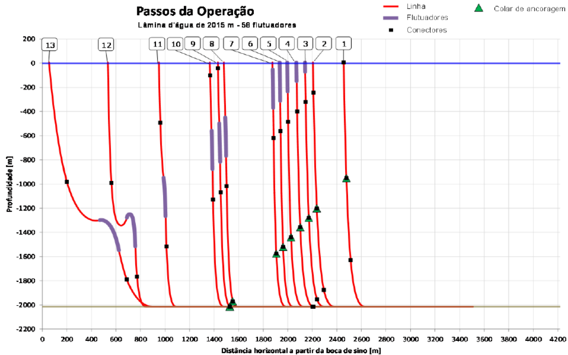
Figura 4.5-3 – Passos da Operação
