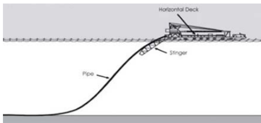
Figura 3.2-1 – S-Lay - [16]
