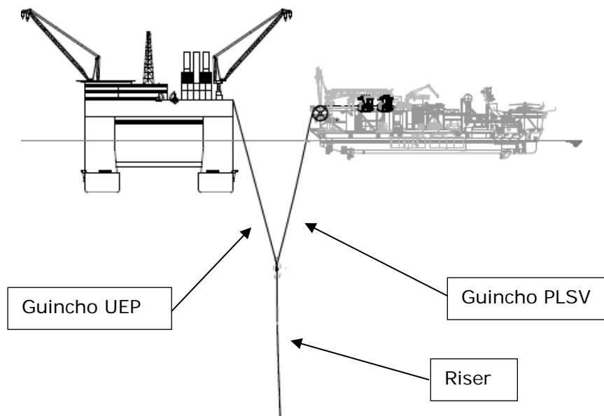
Figura 3.5-6 – Esquemático Pull in 2ª ext.
