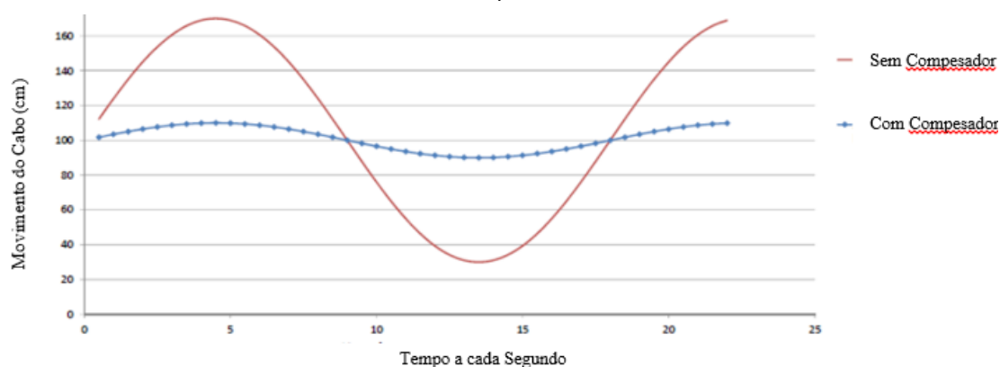
Figura 3.4-6 - Gráfico comparativo Com e Sem Compensador de Heave
