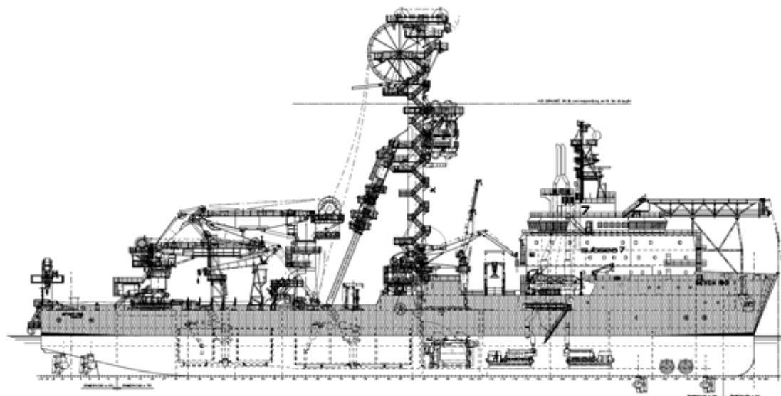
Figura 4.5-1 – Características do PLSV
