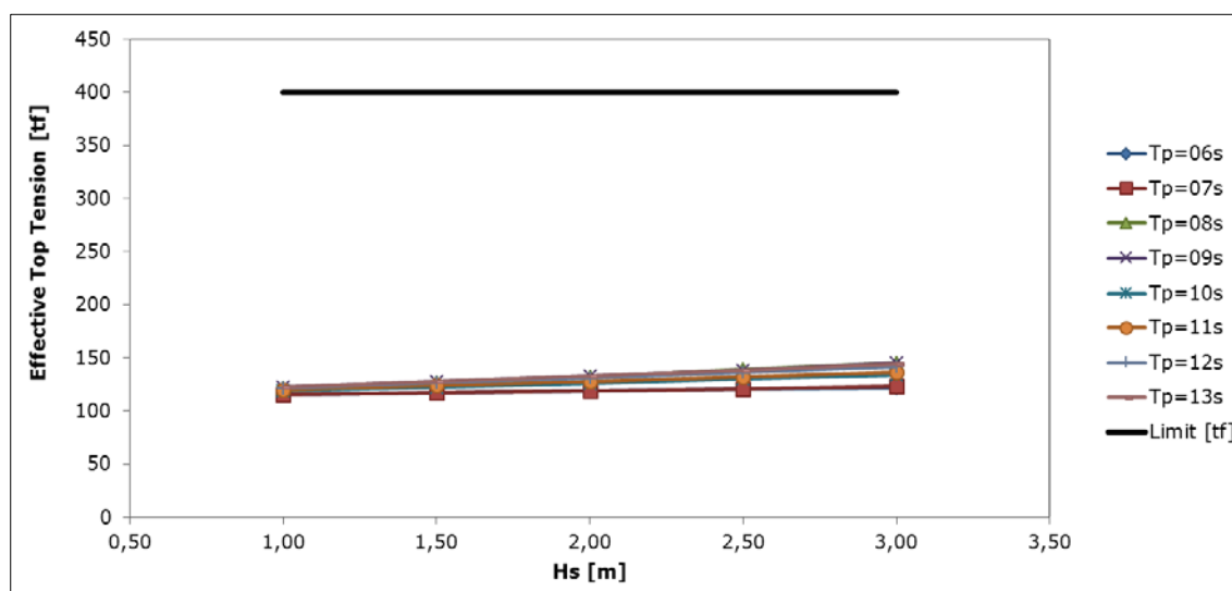
Figura 5.3-1 – Tensão de Topo x Hs 0° 50% dos flutuadores
