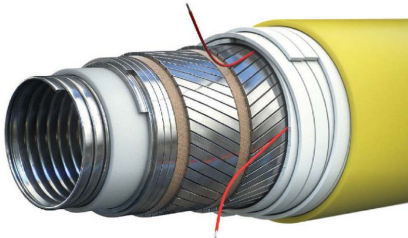
Figura 2.2-3 - Duto Flexível Tipo Unbonded - [8]
