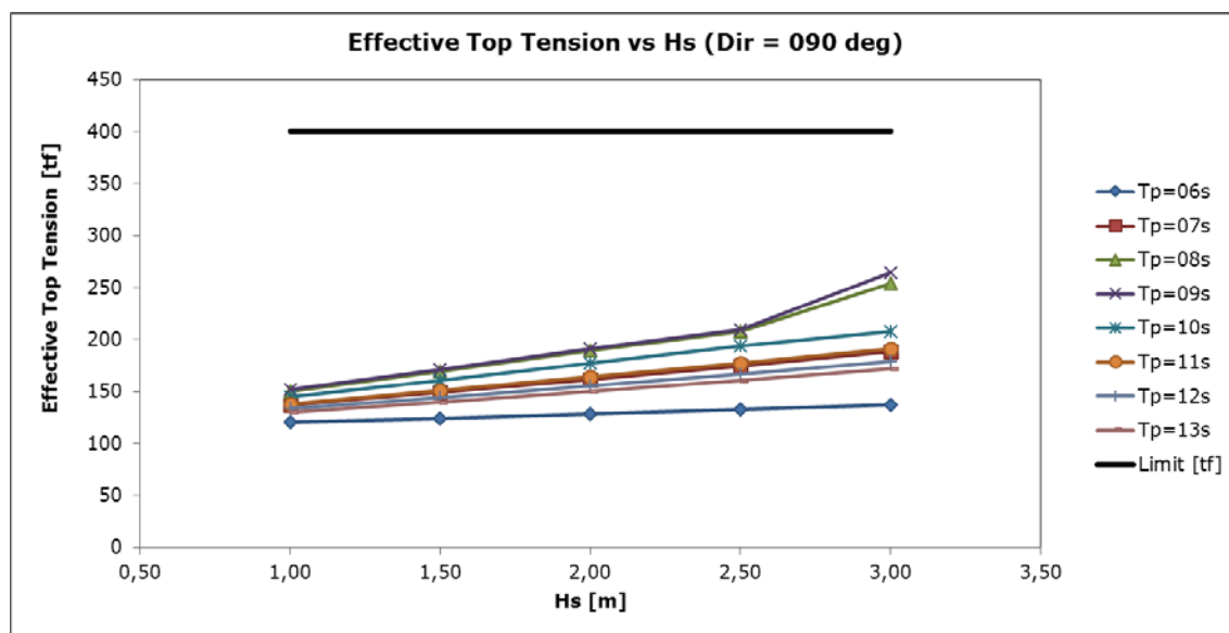
Figura 5.3-2 – Tensão de Topo x Hs 90° 50% dos flutuadores
