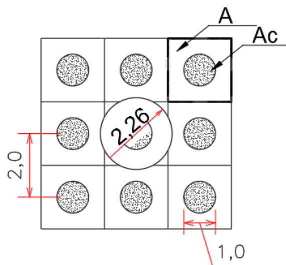
Figura 2.4 – Diâmetro da coluna ( d_c ), diâmetro de influência ( d_e ) e espaçamento ( s )
