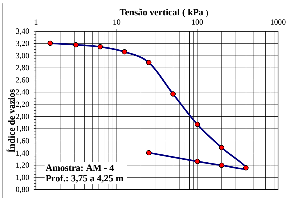
Figura A1.4 – Relação índice de vazios x tensão vertical efetiva ( e\sigma'_v ) – amostra 4
