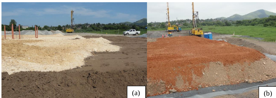
Figura 3.10 – (a) Lançamento da primeira camada e (b) lançamento da quinta camada
