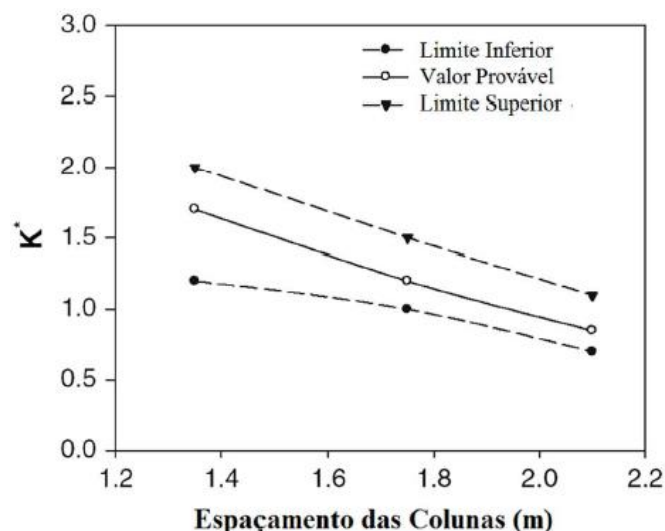
Figura 4.4 – Variação de K^* com o espaçamento de colunas (ELSHAZLY et al., 2008)
