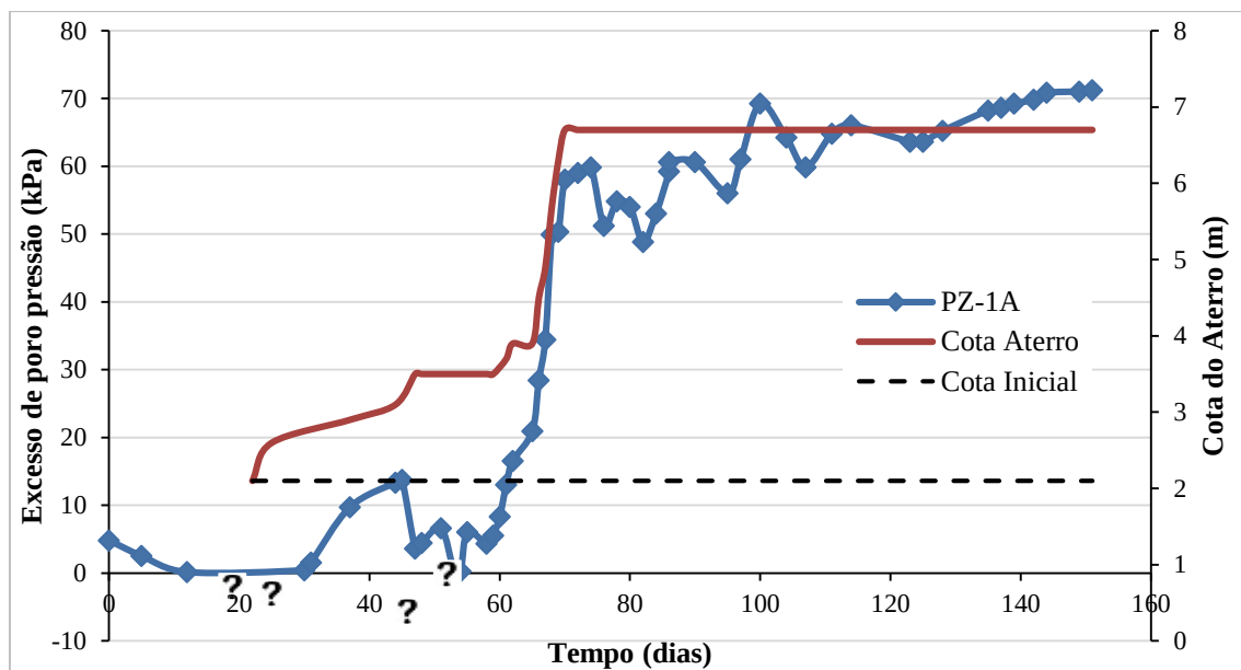
Figura 3.23 – Dados de campo do piezômetro PZ-1A
