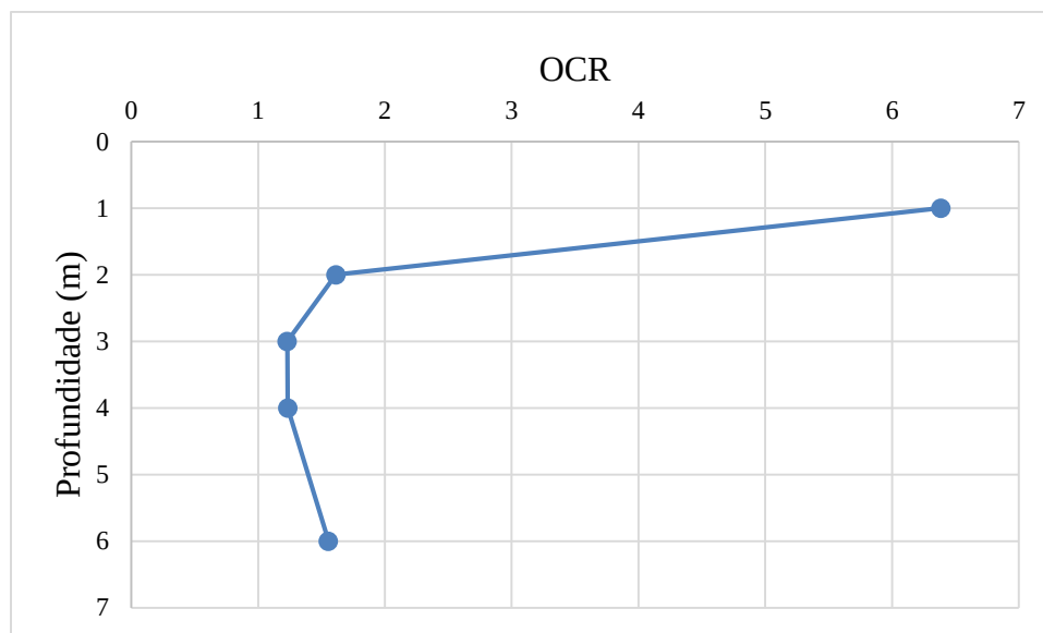
Figura 3.20 – Variação de OCR com a profundidade
