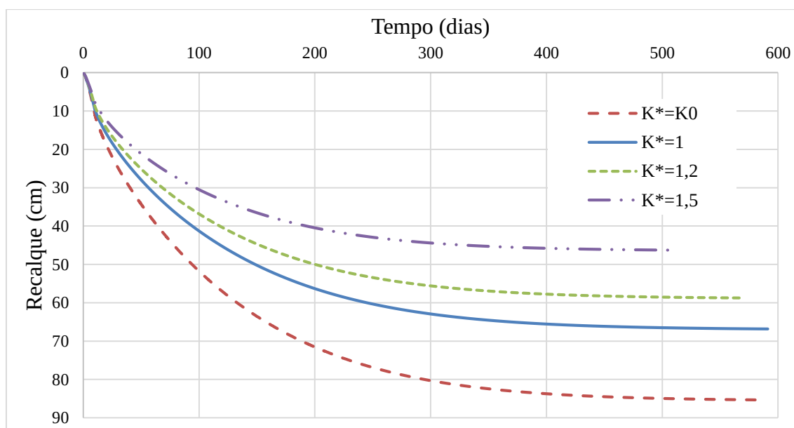
Figura 2.17 – Verificação dos valores de K^* para resultados de recalque
