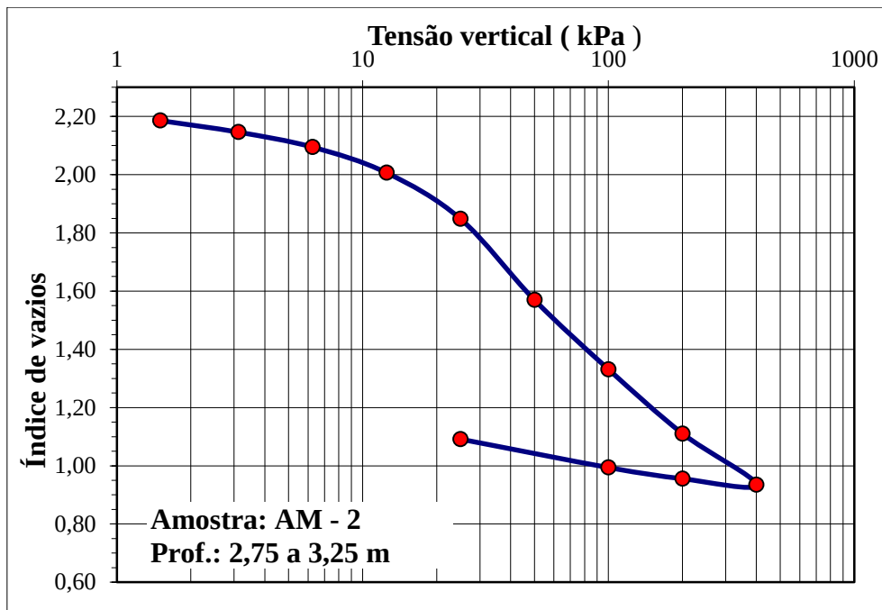
Figura A1.2 – Relação índice de vazios x tensão vertical efetiva- ( e\sigma'_v ) – amostra 2
