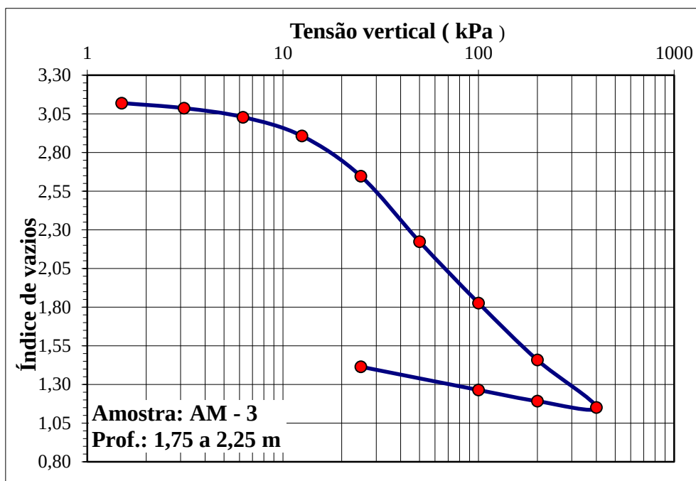
Figura A1.3 – Relação índice de vazios x tensão vertical efetiva- ( e\sigma'_v ) – amostra 3
