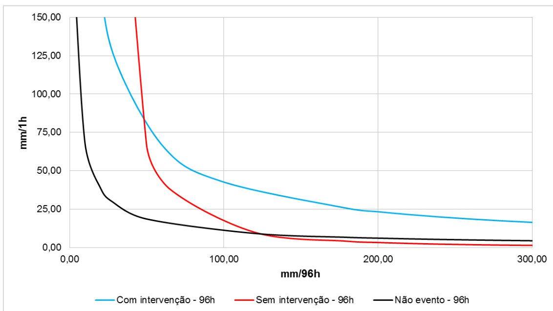
Figura 8.10 – Acumulado de 96hs (mm/96h) versus intensidade horária (mm/1h) para EPS ocorridos na sub-região Grande Méier (Média e desvios padrão) em escala natural para intervenção humana
