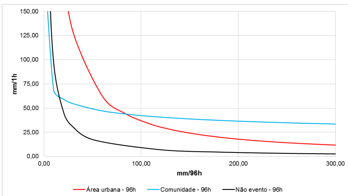
Figura 9.14 – Acumulado de 96hs ( \text{mm/96h} ) versus intensidade horária ( \text{mm/1h} ) para EPS ocorridos na sub-região Ilha do Governador (Média e desvios padrão) em escala natural para tipo de ocupação
