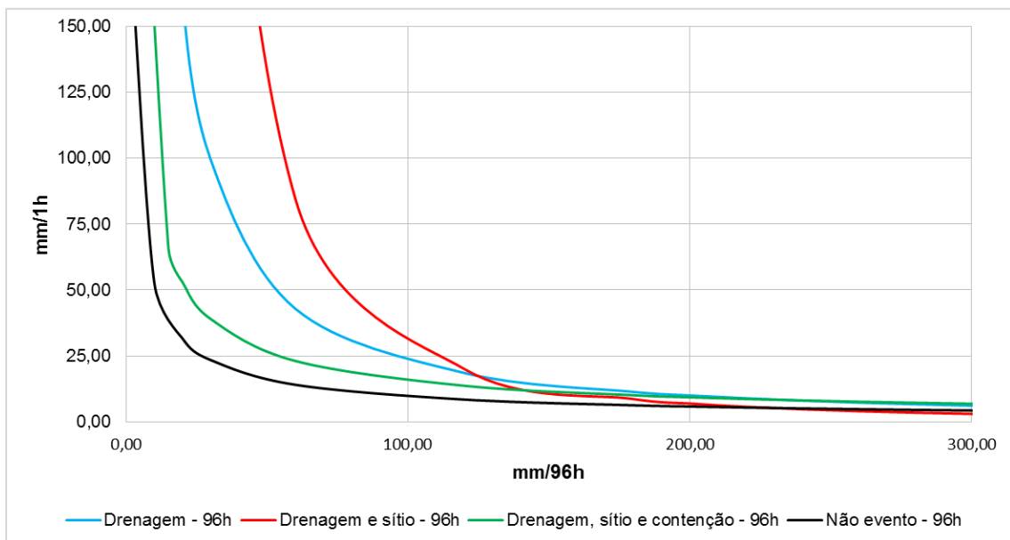
Figura 10.2 – Acumulado de 96hs (mm/96h) versus intensidade horária (mm/1h) para EPS ocorridos na sub-região Anchieta/Irajá (Média e desvios padrão) em escala natural para causas combinadas
