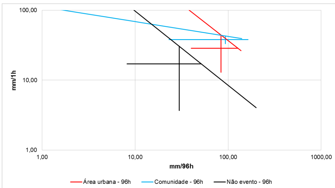
Figura 9.13 – Acumulado de 96hs ( \text{mm/96h} ) versus intensidade horária ( \text{mm/1h} ) para EPS ocorridos na sub-região Ilha do Governador (Média e desvios padrão) em escala logarítmica para tipo de ocupação
