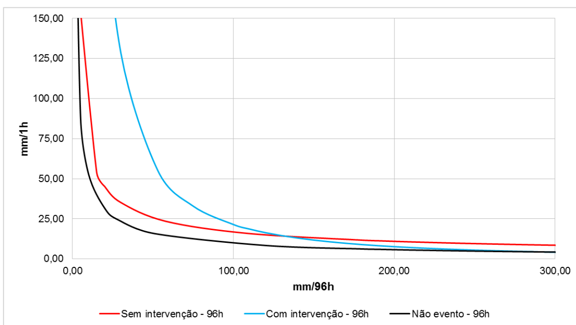
Figura 4.17 – Acumulado de 96hs (mm/96h) versus intensidade horária (mm/1h) para EPS ocorridos na sub-região Anchietá/Irajá (Média e desvios padrão) em escala natural para intervenção humana
