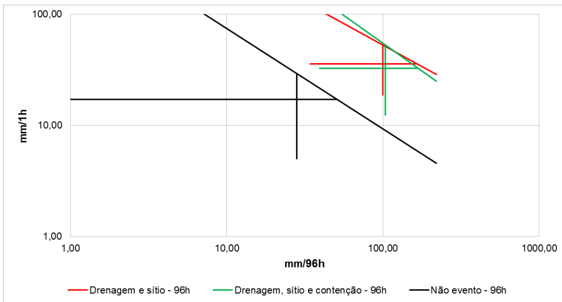
Figura 10.15 – Acumulado de 96hs (mm/96h) versus intensidade horária (mm/1h) para EPS ocorridos na sub-região Jacarepaguá (Média e desvios padrão) em escala logarítmica para causas combinadas
