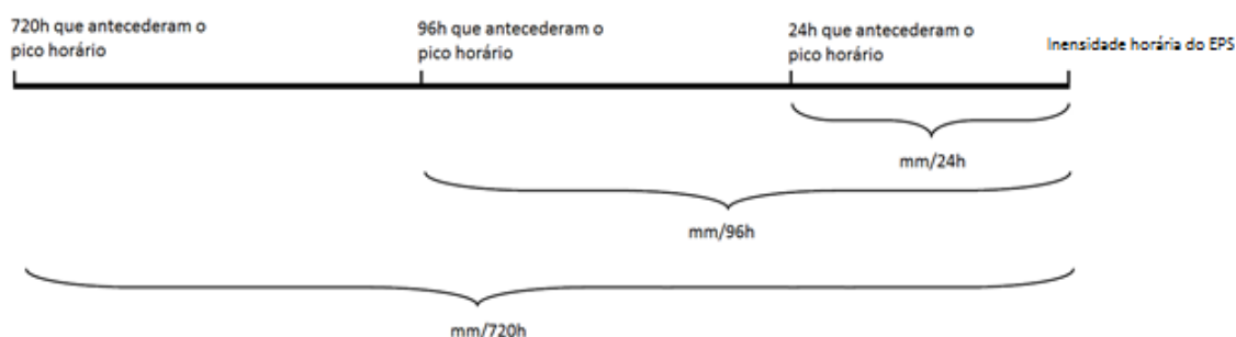
Figura 3.5 – Esquematização exemplificando os acumulados de chuva para mm/24h, mm/96h e mm/720h (Fonte: MENDES, 2016)
