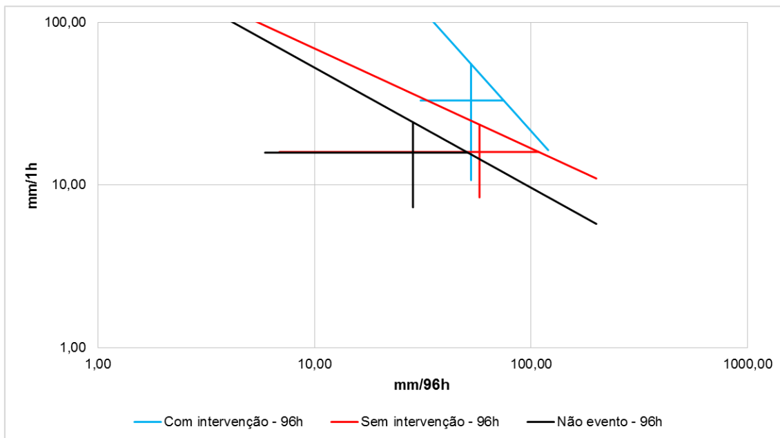
Figura 4.16 – Acumulado de 96hs (mm/96h) versus intensidade horária (mm/1h) para EPS ocorridos na sub-região Anchietá/Irajá (Média e desvios padrão) em escala logarítmica para intervenção humana
