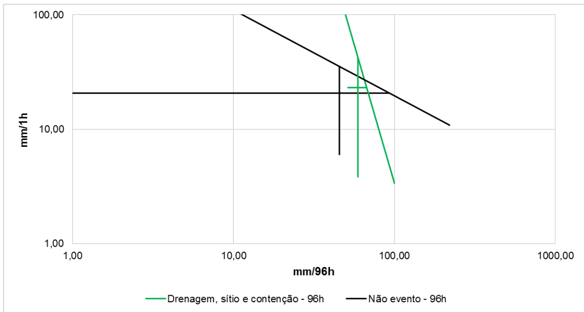
Figura 10.3 – Acumulado de 96hs (mm/96h) versus intensidade horária (mm/1h) para EPS ocorridos na sub-região Barra/Recreio (Média e desvios padrão) em escala logarítmica para causas combinadas
