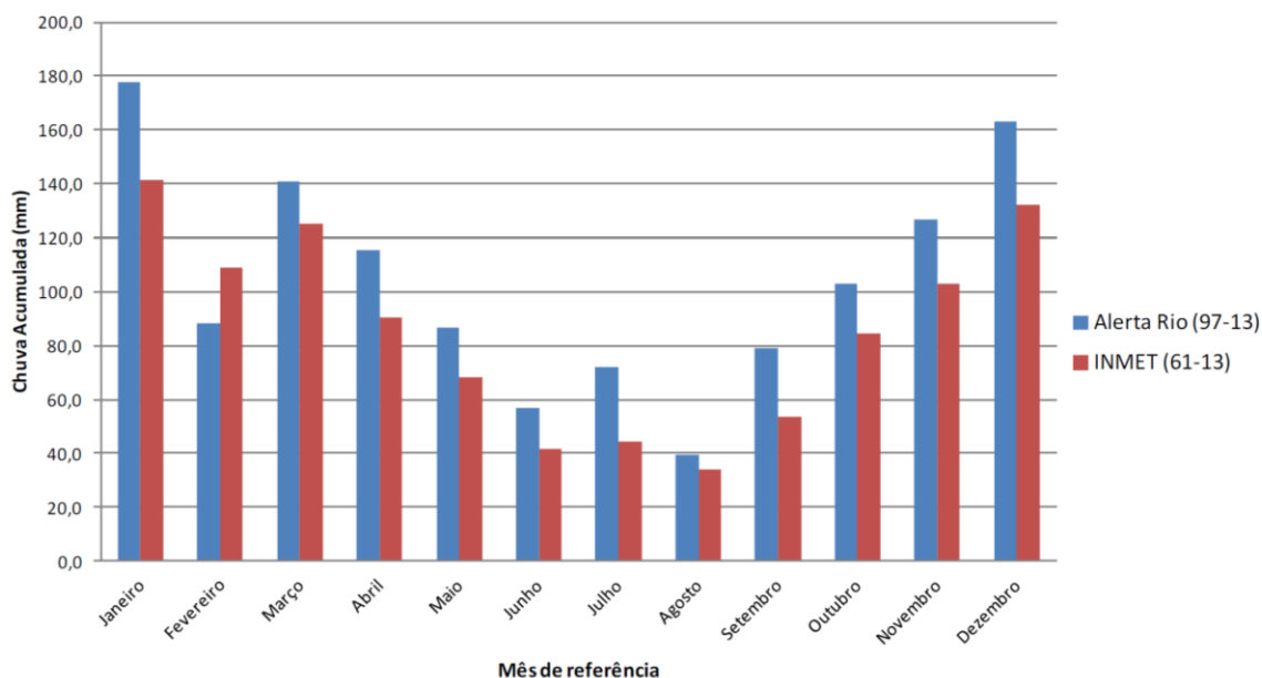
Figura 2.3 - Comparação entre a pluviometria mensal do Alerta Rio e INMET. (Fonte: MARTINS 2014)
