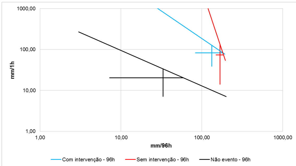
Figura 8.19 - Acumulado de 96hs (mm/96h) versus intensidade horária (mm/1h) para EPS ocorridos na sub-região Zona Oeste (Média e desvios padrão) em escala logarítmica para intervenção humana
