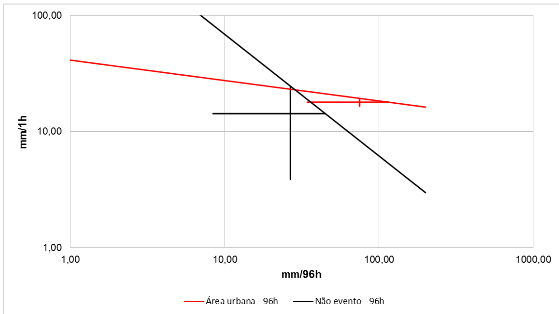
Figura 9.3 – Acumulado de 96hs ( \text{mm/96h} ) versus intensidade horária ( \text{mm/1h} ) para EPS ocorridos na sub-região Bangu (Média e desvios padrão) em escala logarítmica para tipo de ocupação
