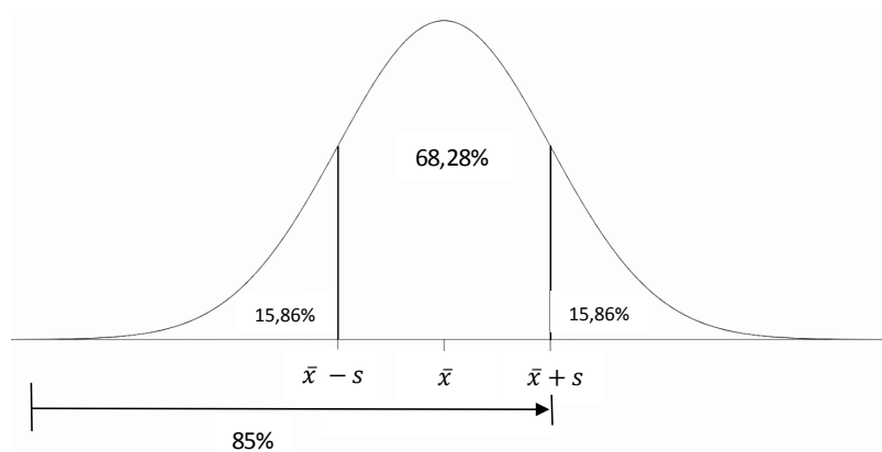
Figura 3.8 – Gráfico de desvio padrão
