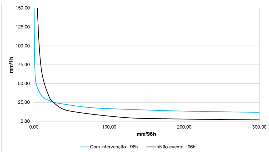
Figura 8.4 – Acumulado de 96hs (mm/96h) versus intensidade horária (mm/1h) para EPS ocorridos na sub-região Bangu (Média e desvios padrão) em escala natural para intervenção humana
