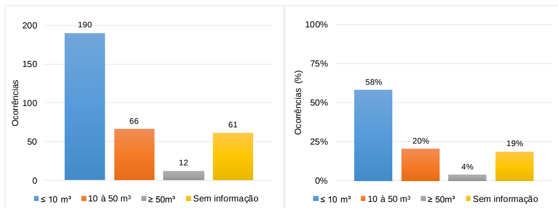
Figura 4.3 – Volumes deslizados das ocorrências de 1998 a 2002
