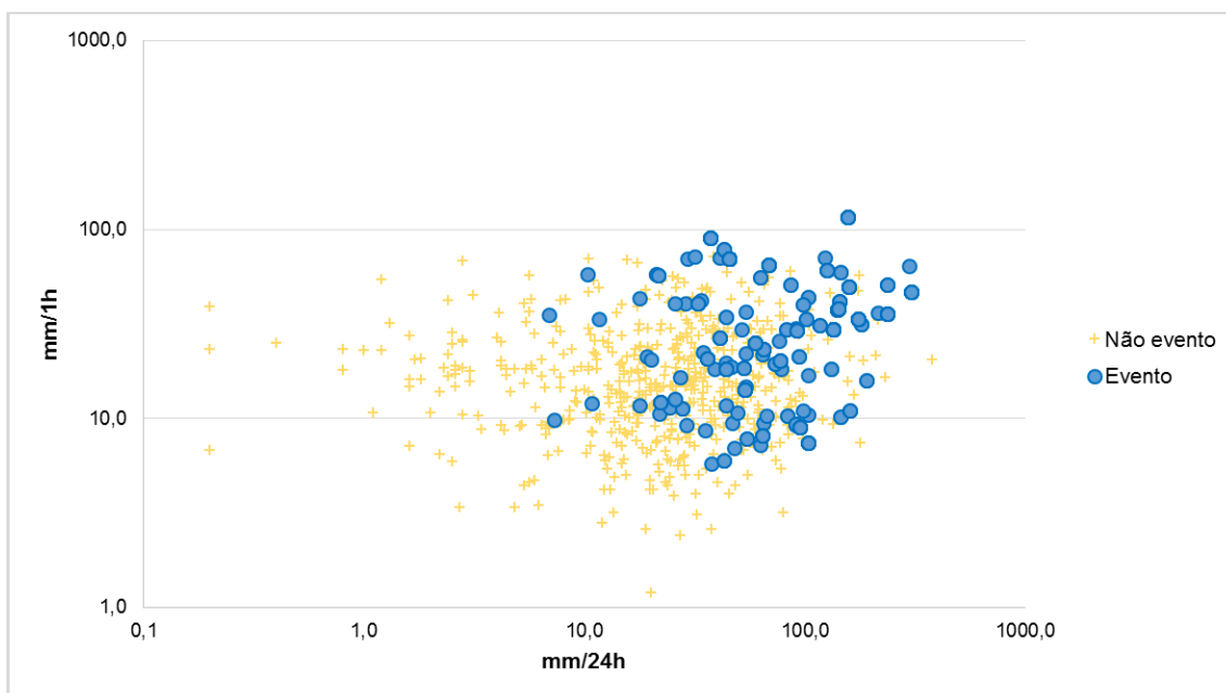
Figura 14.2 - Acumulado de 96h (mm/96h) versus intensidade horária (mm/1h) para categoria “Evento” e “Não evento” na cidade do Rio de Janeiro
