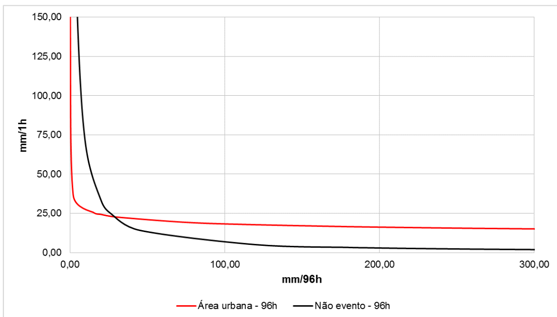
Figura 9.4 – Acumulado de 96hs ( \text{mm/96h} ) versus intensidade horária ( \text{mm/1h} ) para EPS ocorridos na sub-região Bangu (Média e desvios padrão) em escala natural para tipo de ocupação
