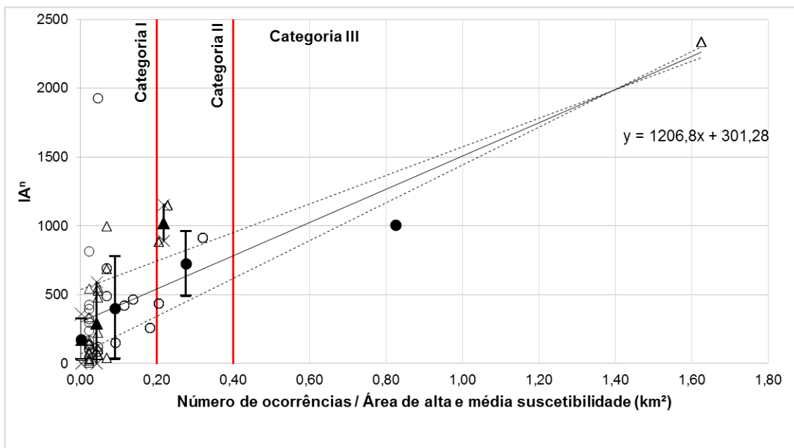
Figura 12.9 – Número de ocorrência/área de suscetibilidade versus IA^n (96hs) da sub-região de Grande Méier, acumulados de 96h para 1998-2002 e 2010-2012
