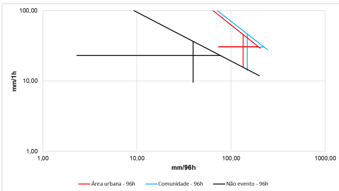
Figura 9.7 – Acumulado de 96hs (mm/96h) versus intensidade horária (mm/1h) para EPS ocorridos na sub-região Centro (Média e desvios padrão) em escala logarítmica para tipo de ocupação
