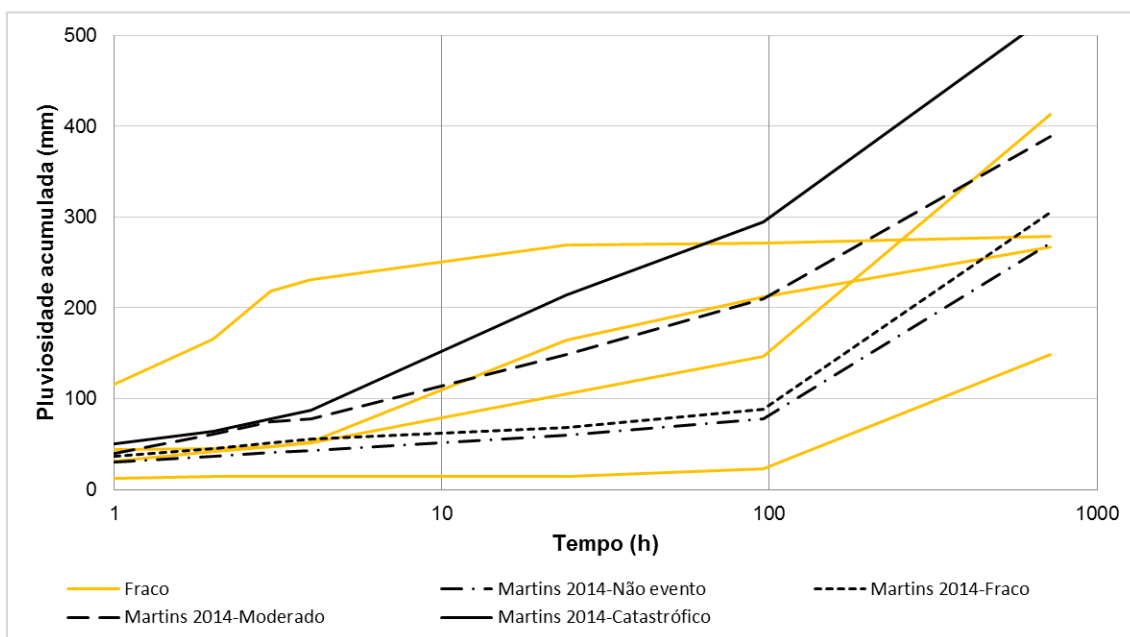
Figura 7.9 – Comparação dos limiares determinados por MARTINS (2014) com as curvas de pluviosidade acumulada (mm) por tempo (h) para sub-região Zona Oeste
