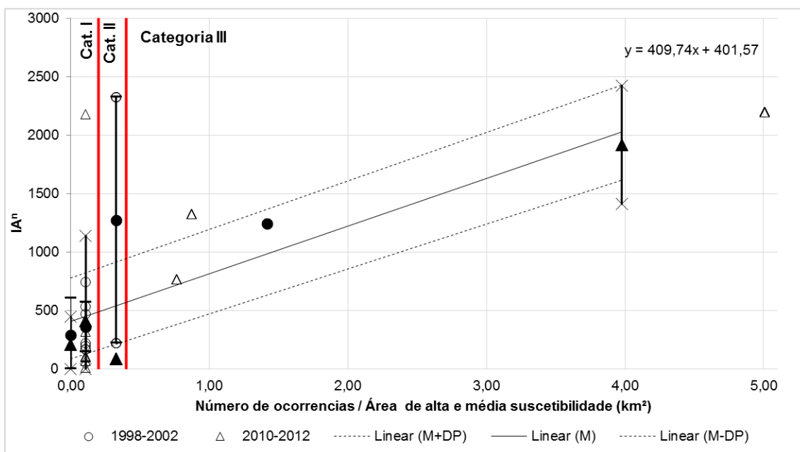
Figura 12.7 – Número de ocorrência/área de suscetibilidade versus IA^n (96hs) da sub-região de Centro, acumulados de 96h para 1998-2002 e 2010-2012
