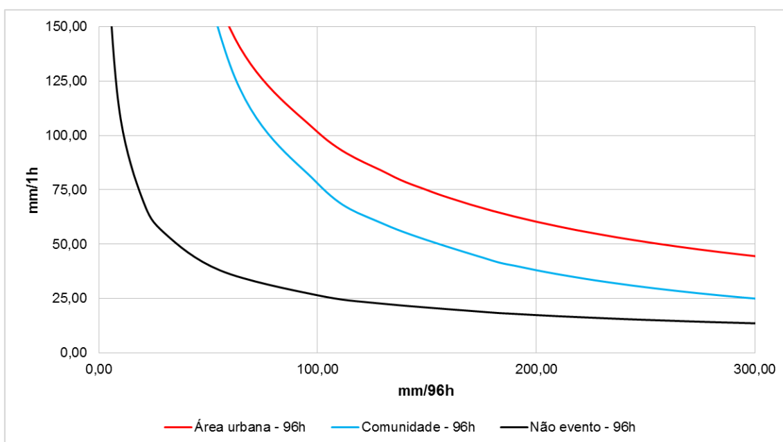
Figura 9.12 – Acumulado de 96hs (mm/96h) versus intensidade horária (mm/1h) para EPS ocorridos na sub-região Grande Tijuca (Média e desvios padrão) em escala natural para tipo de ocupação
