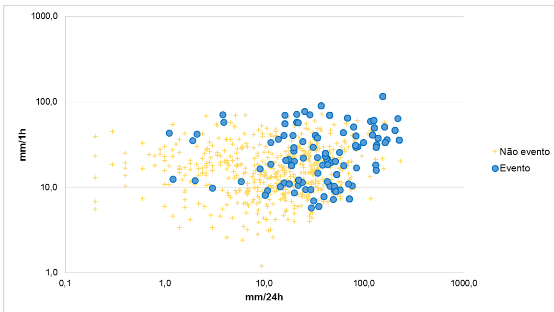
Figura 14.1 – Acumulado de 24h (mm/24h) versus intensidade horária (mm/1h) para categoria “Evento” e “Não evento” na cidade do Rio de Janeiro
