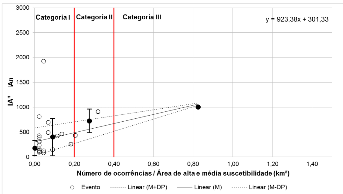
Figura 4.37 – Número de ocorrências por área de suscetibilidade (km²) versus IA^n , sub-região Grande Méier para acumulados de 96h
