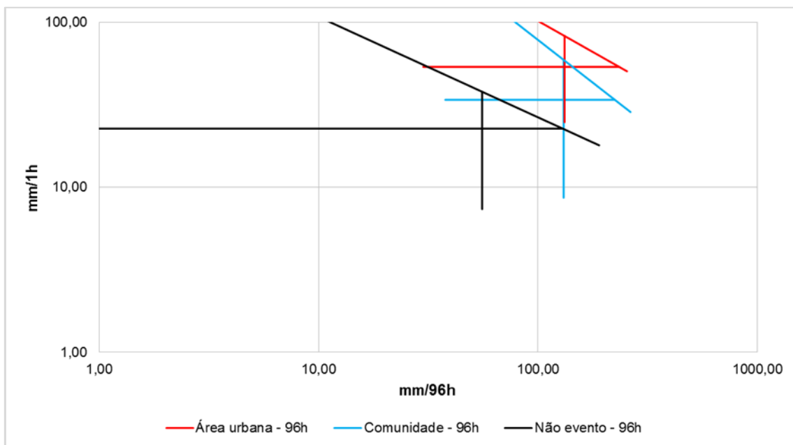
Figura 4.14 – Acumulado de 96hs (mm/96h) versus intensidade horária (mm/1h) para EPS ocorridos na sub-região Grande Tijuca (Média e desvios padrão) em escala logarítmica para tipo de ocupação
