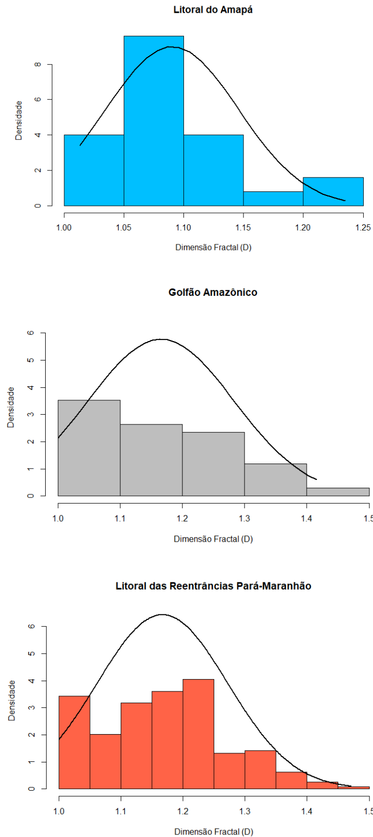
Figura 23- Histogramas dos valores da dimensão fractal dos manguezais por macrocompartmento.
