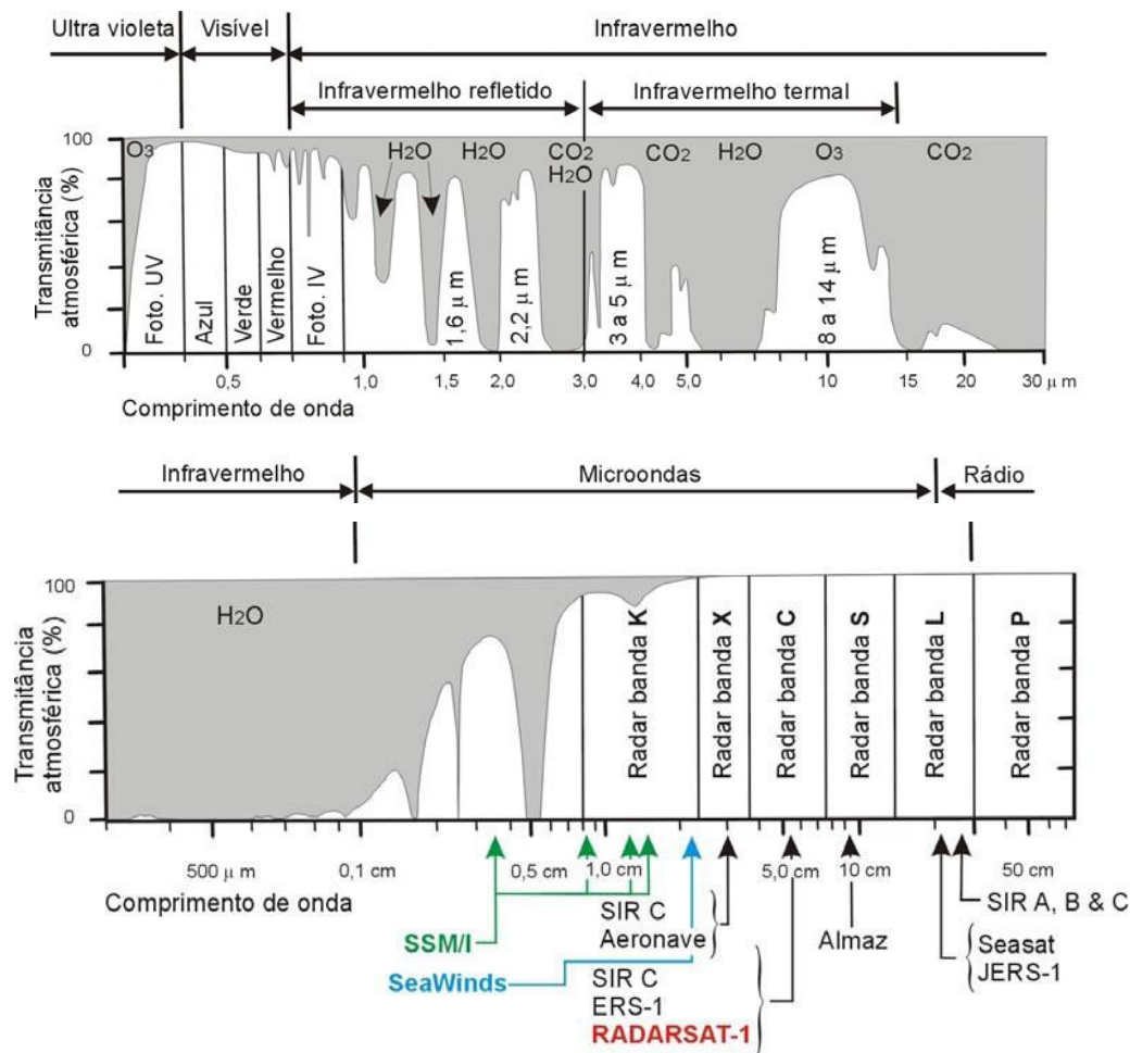
Figura 9- Diagrama apresentando o espectro eletromagnético versus a transmitância atmosférica. Fonte: RORIZ (2006).
