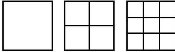
Figura 18 - Quadrados divididos em N^2 partes iguais, com N=1, 2 e 3 . Fonte: SILVA & SOUZA (2010).
