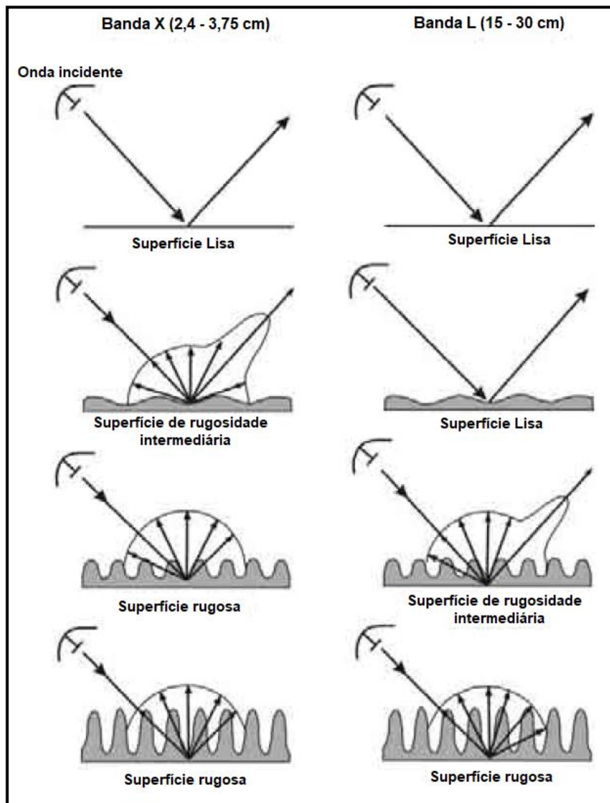
Figura 12 – Mecanismos de interação com o terreno do pulso do radar para as bandas X e L em diferentes superfícies. Fonte: RORIZ (2006). A reflexão especular ocorre nas superfícies lisas; o retroespalhamento difuso, nas rugosas.
