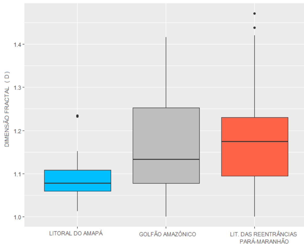
Figura 24- Boxplot dos valores da dimensão fractal dos manguezais por macrocompartmento.
