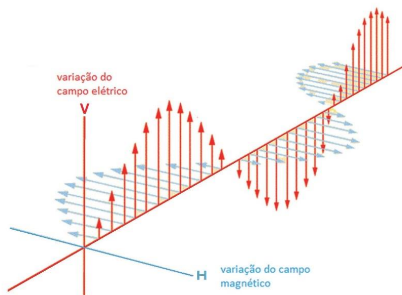
Figura 7 – Propagação da onda eletromagnética. Adaptado de BAGNATO & PRATAVIEIRA (2015).
