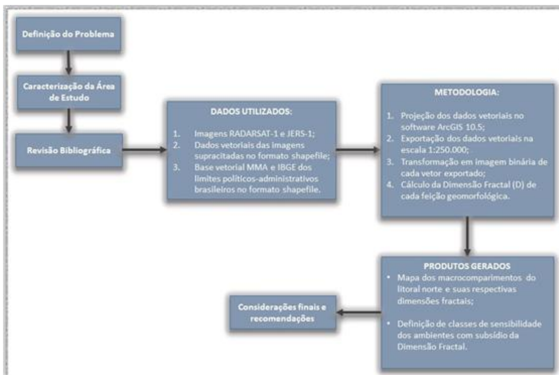
Figura 2 - Fluxograma da metodologia proposta para a presente na dissertação.
