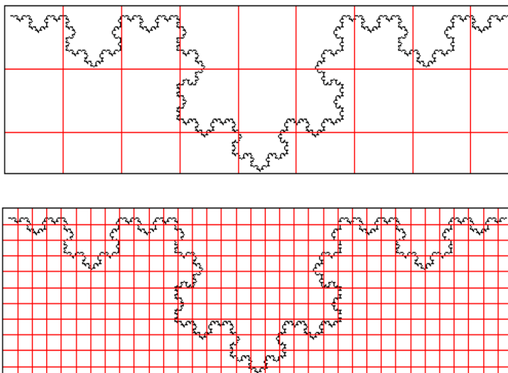
Figura 21- Exemplo de um objeto coberto pelas “caixas” do método box counting . Fonte: (MACEDO et al. , 2017).
