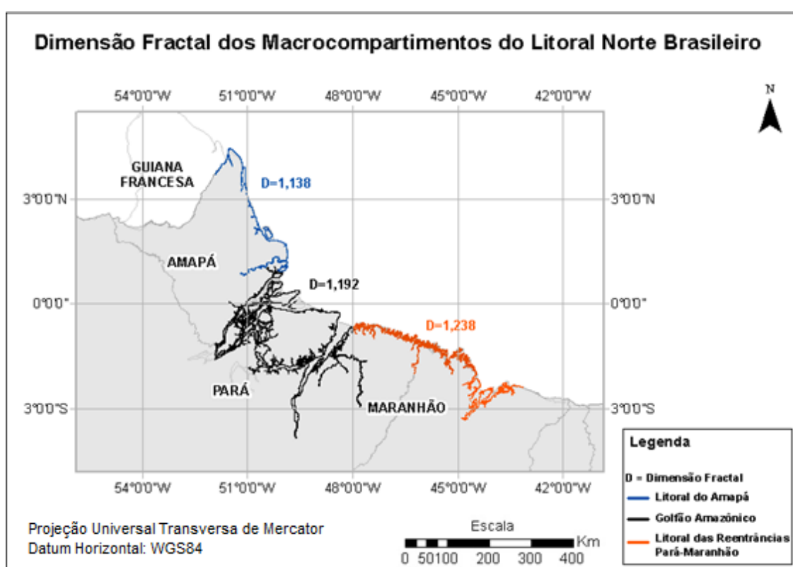
Figura 25– Dimensão fractal dos macrocompartimentos do Litoral Norte Brasileiro.
