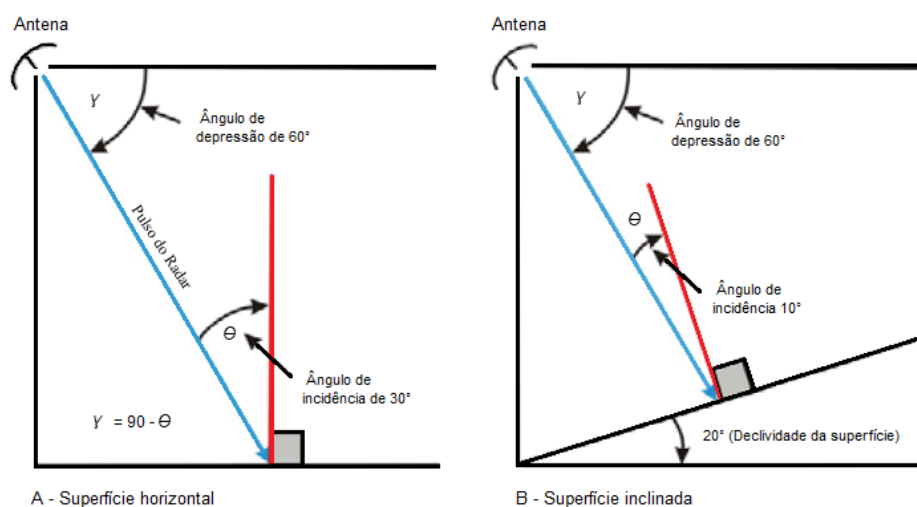
Figura 11– Diagrama ilustrando os conceitos de ângulo de incidência e ângulo de depressão. Adaptado de SABINS (1997).
