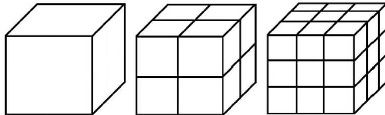
Figura 19- Cubos divididos em N^3 partes iguais, com N = 1, 2 e 3 . Fonte: SILVA & SOUZA (2010).
