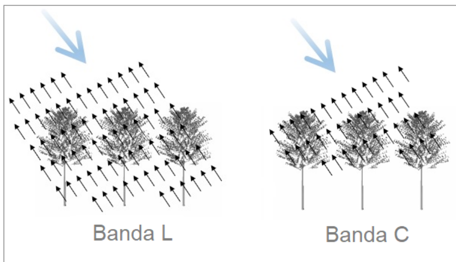
Figura 10- Penetração no dossel vegetal do pulso incidente para diferentes sistemas de radar (bandas L e C). Adaptado de (BITENCOURT, 2011).
