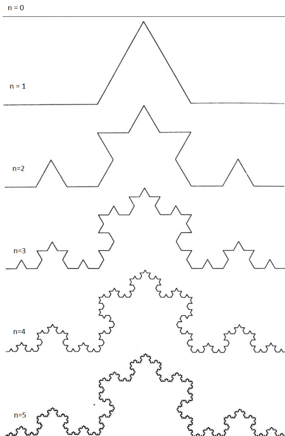
Figura 20- Construção da curva triádica de Koch. Fonte: FEDER (1989)
