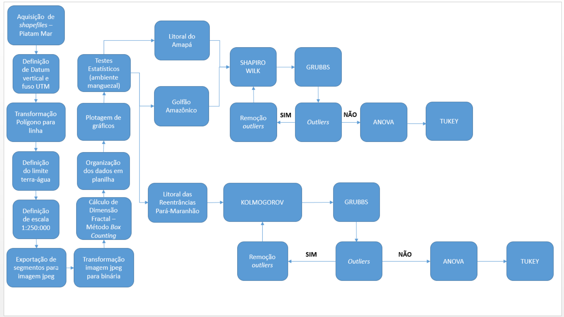
Figura 22- Fluxograma da metodologia empregada na pesquisa.
