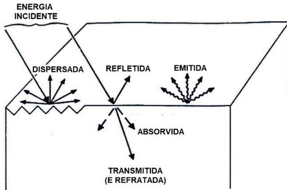
Figura 8 - Processos de interação entre a energia eletromagnética e os alvos. Modificada de SABINS (1997).
