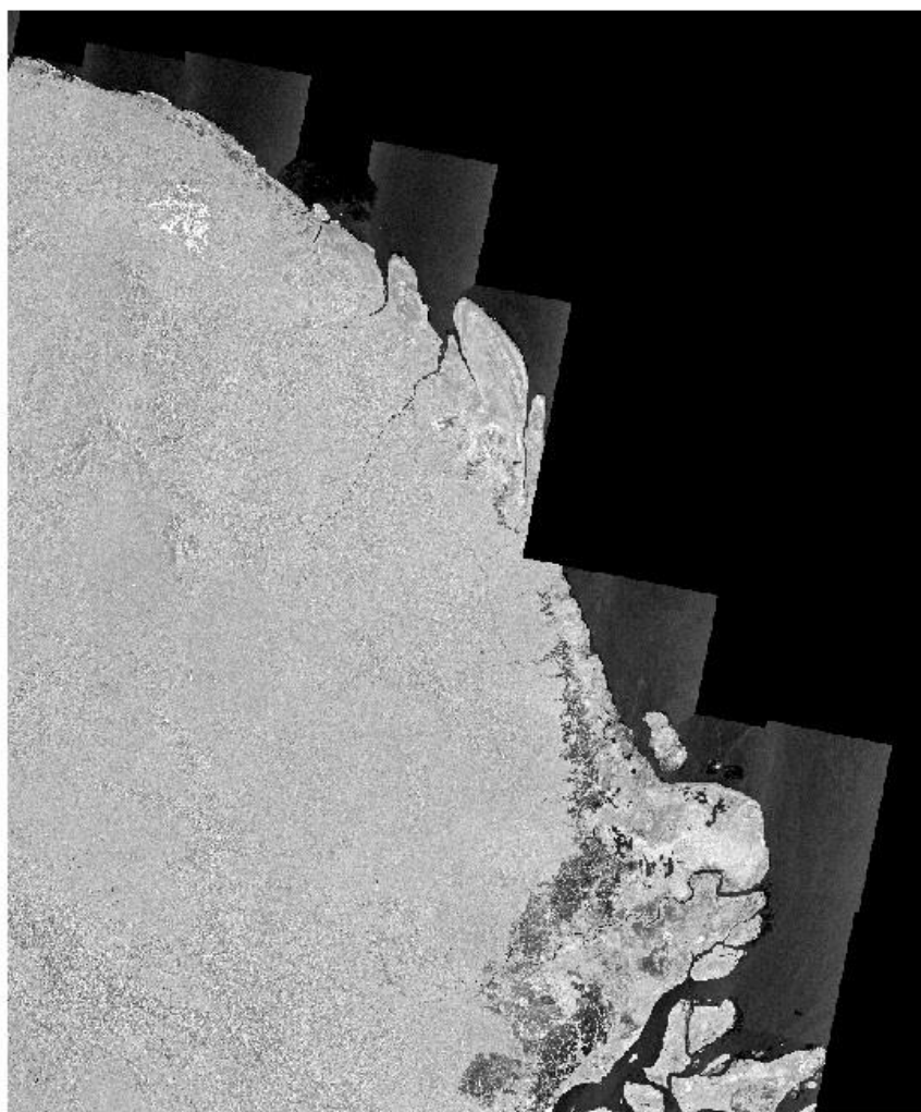
Figura 13 - Mosaico JERS-1 SAR de parte da costa do Amapá elaborado pelo JERS-1 Global Rain Forest Mapping Project (NASA et al. , 2000).
