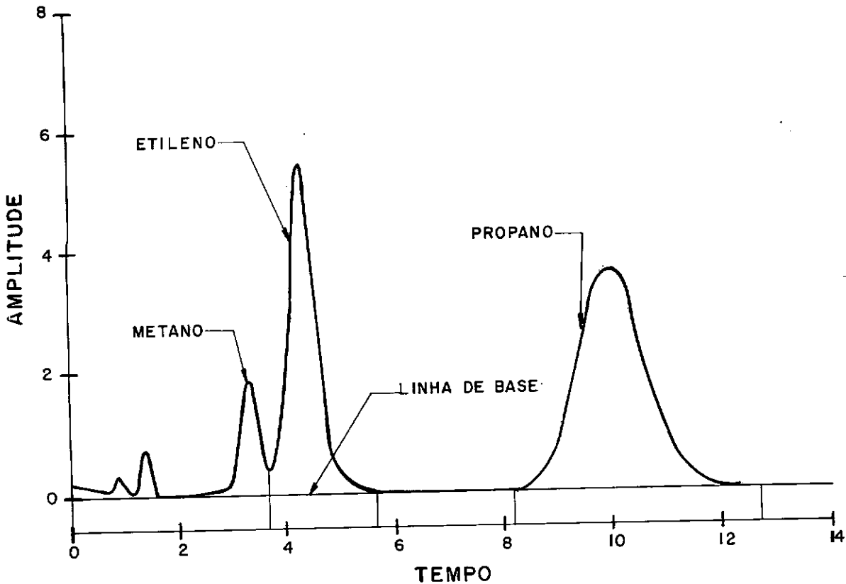
FIGURA IV.5 - Cromatograma Típico
