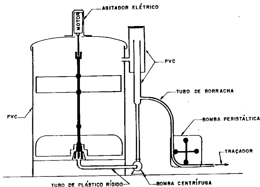
FIGURA IV.3 - Esquema do injetor contínuo de traçador fluorescente desenvolvido no L.T./COPPE-UFRJ
