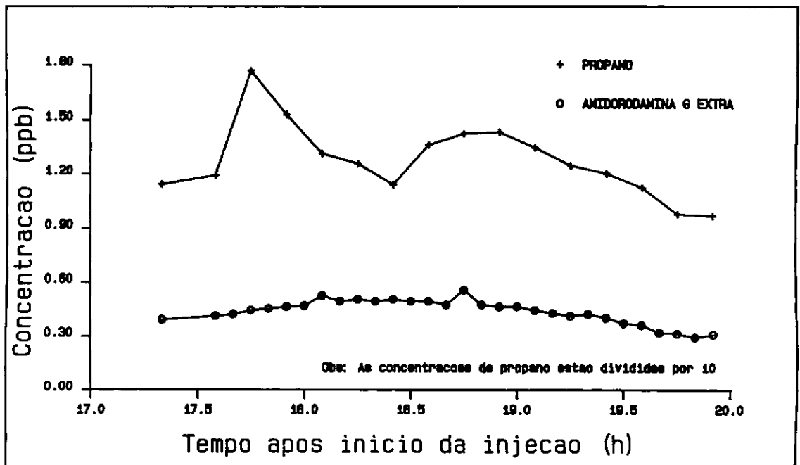
FIGURA V.5 - Curvas de Passagem de Amidorodamina G Extra e Propano na Seção 4 (36,7 km) - rio Paraíba do Sul
