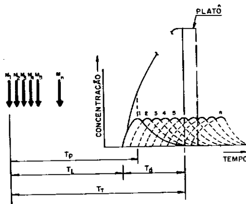
FIGURA II.3 - Superposição das curvas de passagem de uma injeção instantânea (Adaptada de Kilpatrick et alli, 1987).
