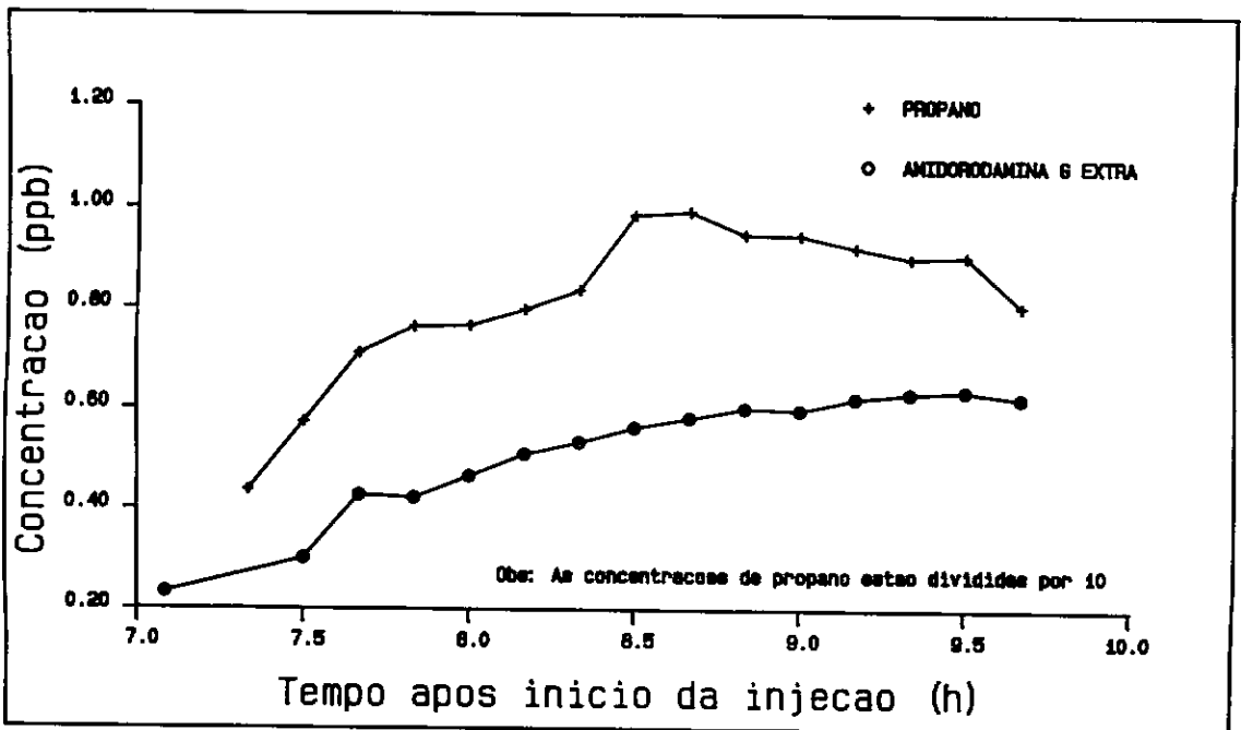
FIGURA V.3 - Curvas de Passagem de Amidorodamina G Extra e Propano na Seção 2 (16,7 km) - rio Paraíba do Sul
