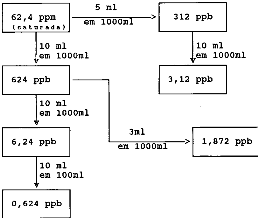
FIGURA IV.7 - Esquema de diluição dos padrões de propano.
