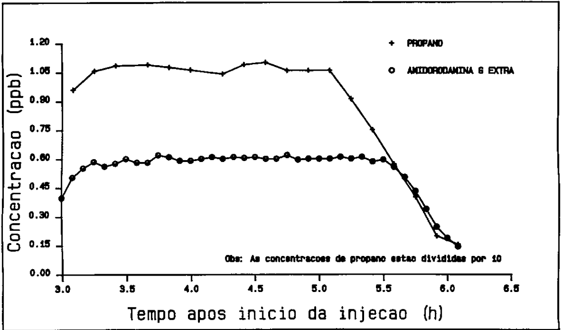
FIGURA V.2 - Curvas de Passagem de Amidorodamina G Extra e Propano na Seção 1 (6,9 km) - rio Paraíba do Sul
