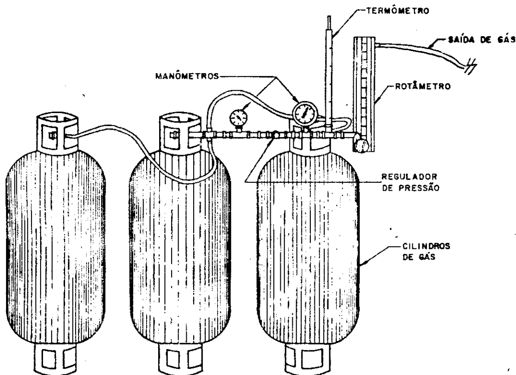
FIGURA IV.2 - Esquema de montagem dos equipamentos utilizados na injeção contínua de traçador gasoso.
