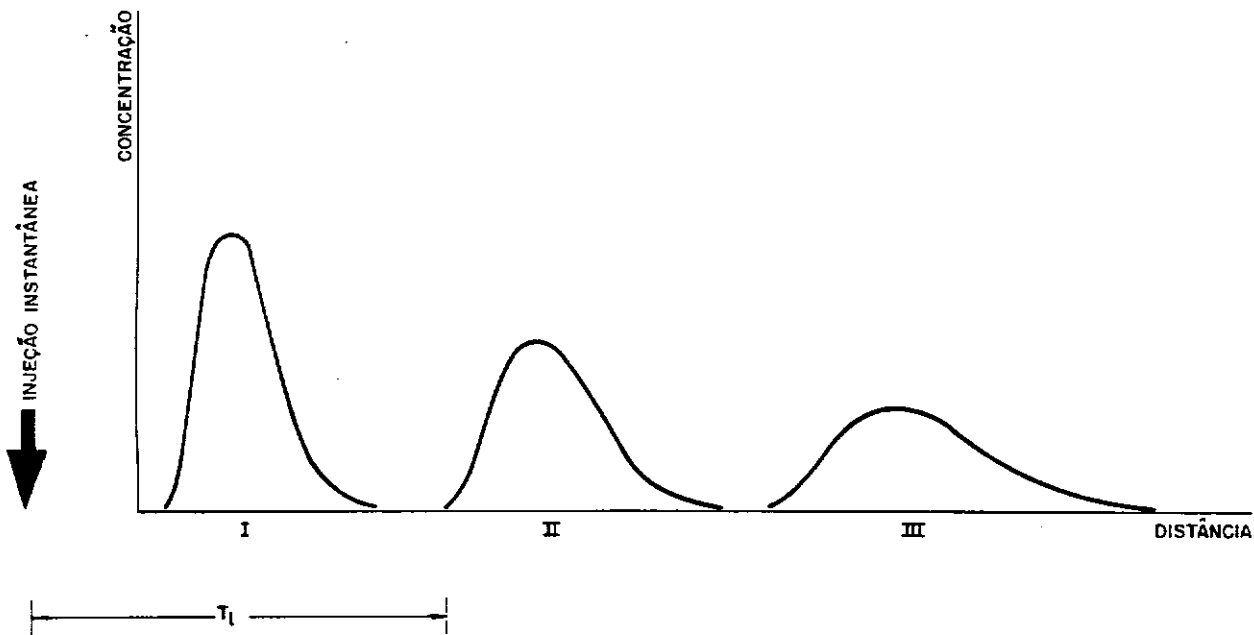
FIGURA II.2 - Curvas C \times t em três pontos ao longo do rio para uma injeção instantânea central.
