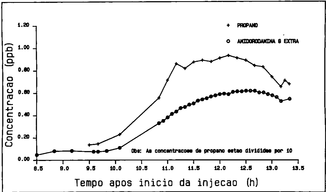
FIGURA V.4 - Curvas de Passagem de Amidorodamina G Extra e Propano na Seção 3 (25,4 km) - rio Paraíba do Sul
