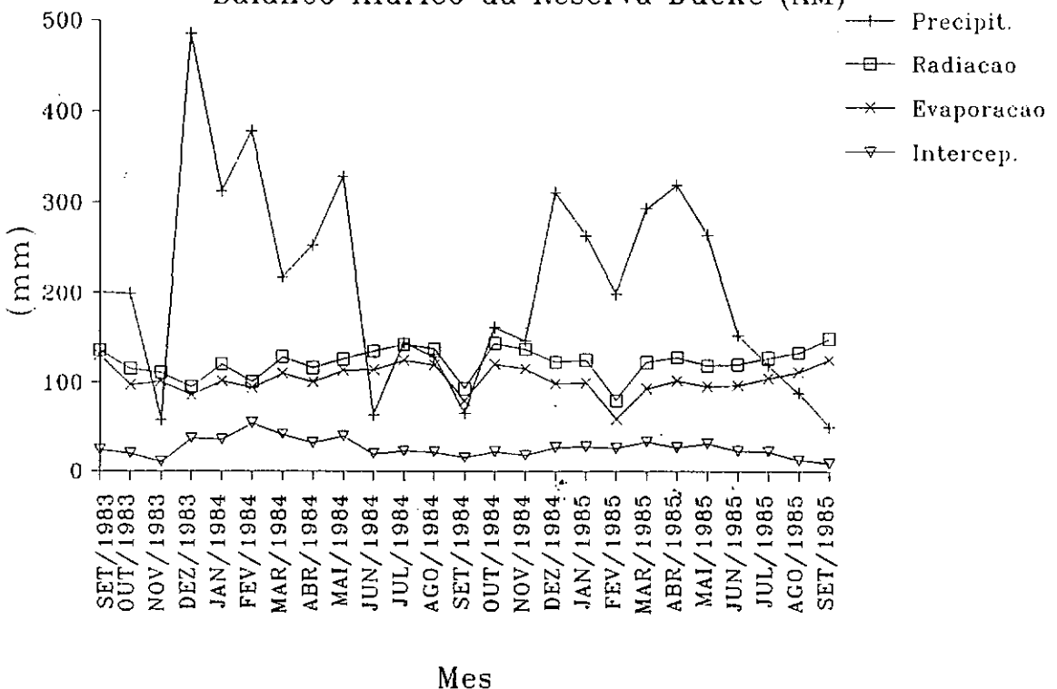
Figura 3.4 - Modelo SIMBAH Balanco Hidrico da Reserva Ducke (AM)
