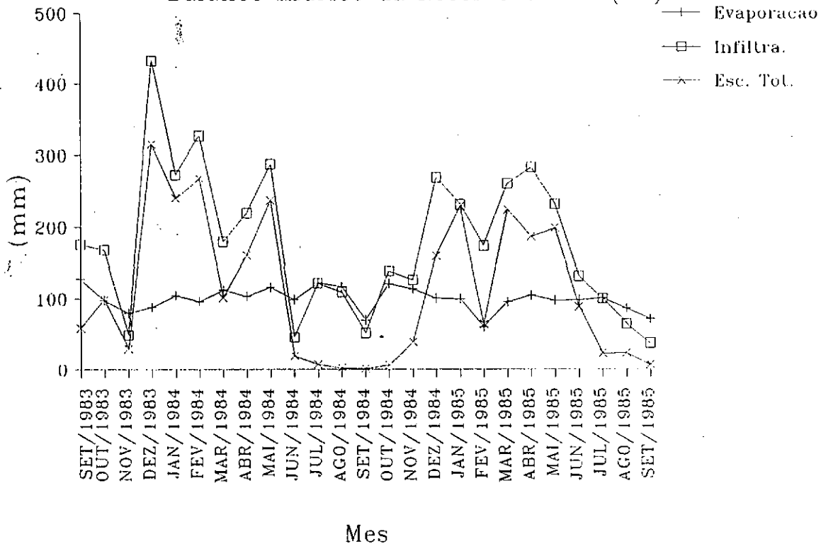
Figura 4.2 - Modelo SIMBAH Balanco Hidrico da Reserva Ducke (AM)
