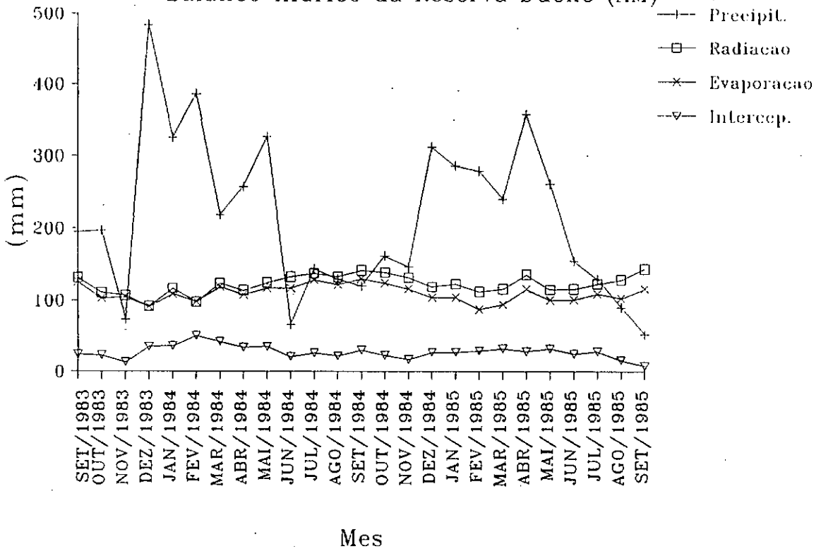
Figura 3.3 - Modelo Shuttleworth Balanco Hidrico da Reserva Ducke (AM)
