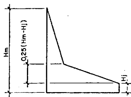
FIGURA II.3.b – DIAGRAMAS DE SUBPRESSÕES PROPOSTOS PELO T.V.A. APUD ANDRADE (2)
