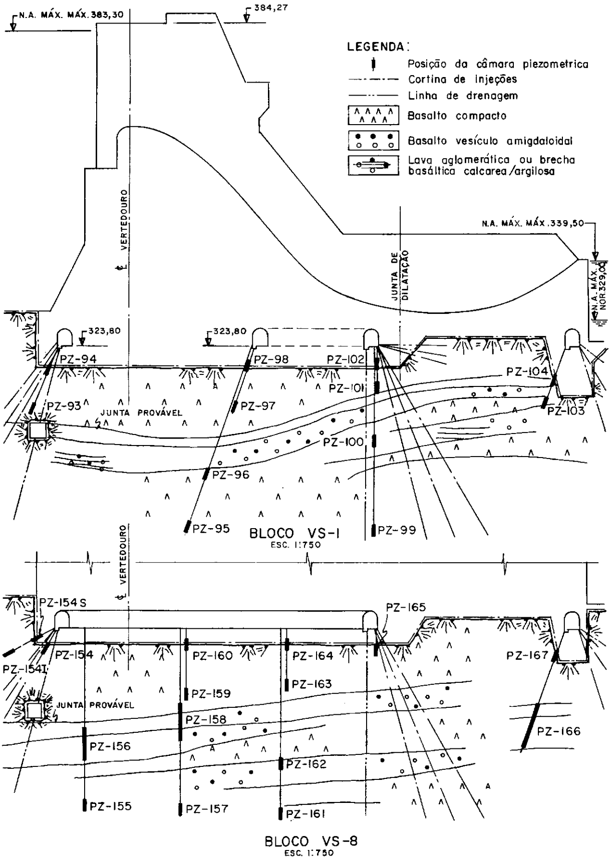
FIGURA III. 15 - USINA ÁGUA VERMELHA - VERTEDOURO SEÇÕES TRANSVERSAIS ESQUEMA DE INSTALAÇÃO DOS PIEZÔMETROS
