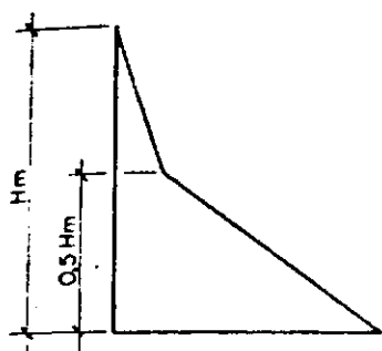
FIGURA II.3.b – DIAGRAMAS DE SUBPRESSÕES PROPOSTOS PELO T.V.A. APUD ANDRADE (2)
