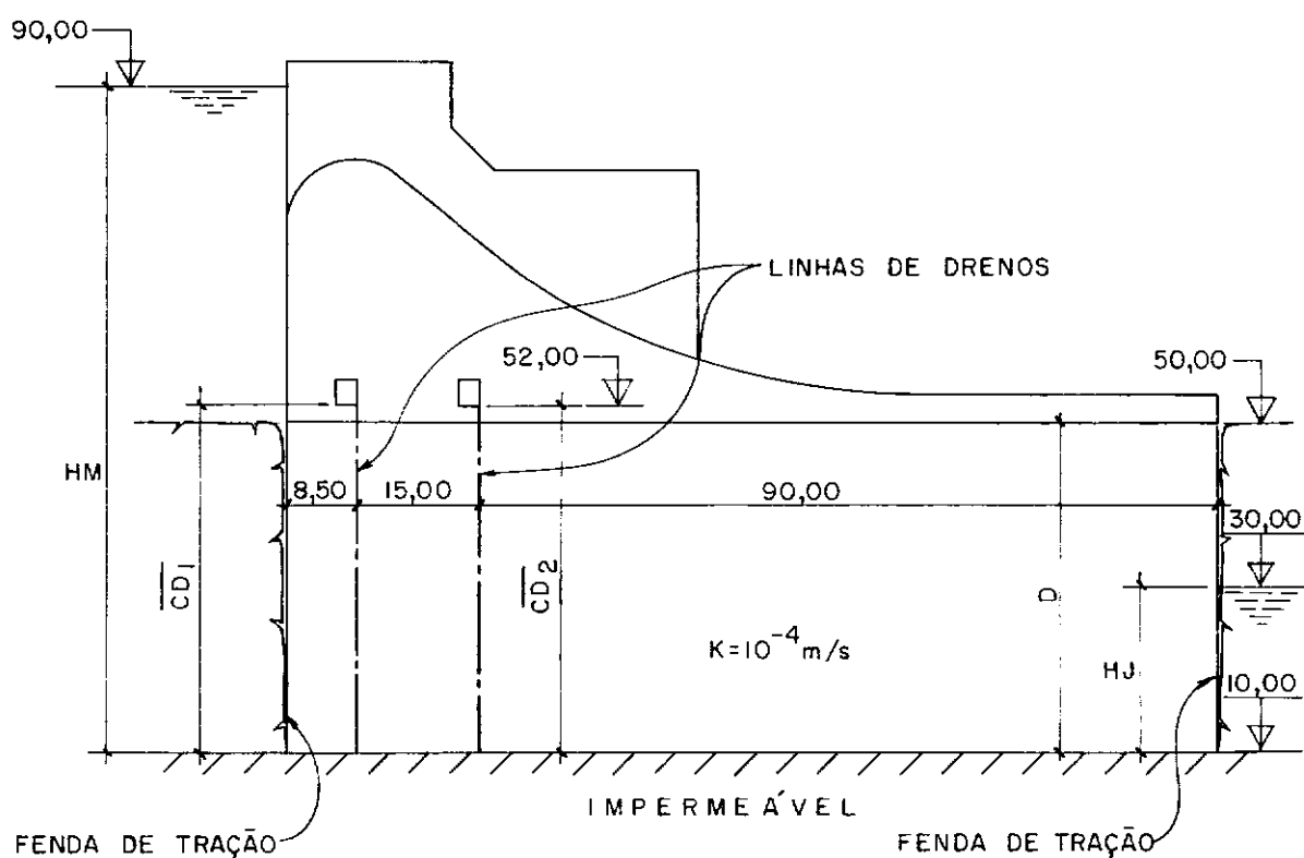
FIG.3.b - 2 LINHAS DE DRENOS COM PENETRAÇÃO TOTAL
