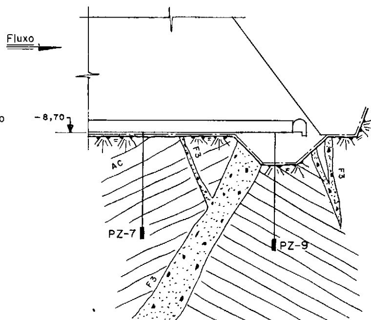
SEÇÃO 2-2
