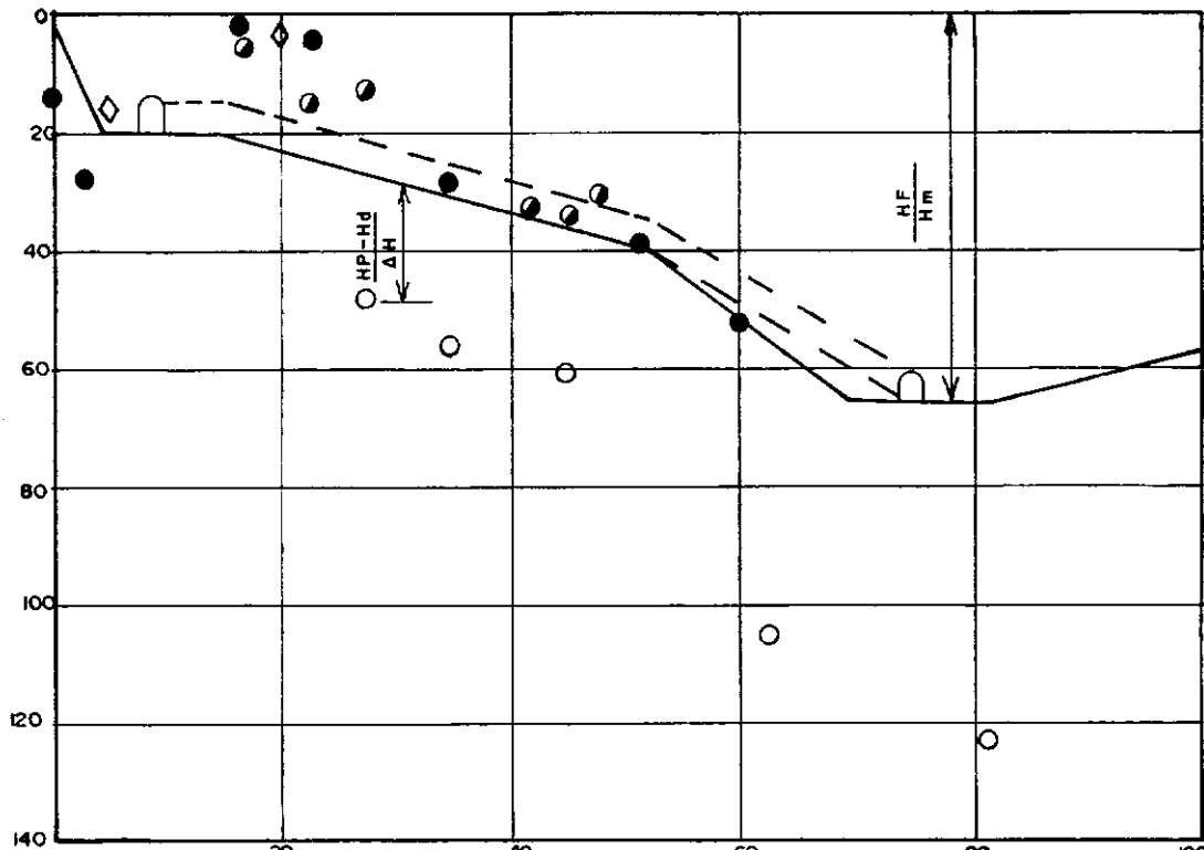
FIGURA III. 19 - SUBPRESSÕES EM DESCONTINUIDADES NA FUNDAÇÃO DE ESTR. DE CONCRETO COM B=2,0H E FUNDAÇÃO EM DIFERENTES NÍVEIS. (TOMADA D'ÁGUA/CASA DE FORÇA)
