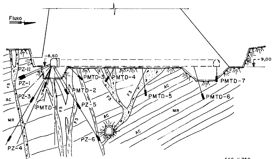
SEÇÃO 1-1
