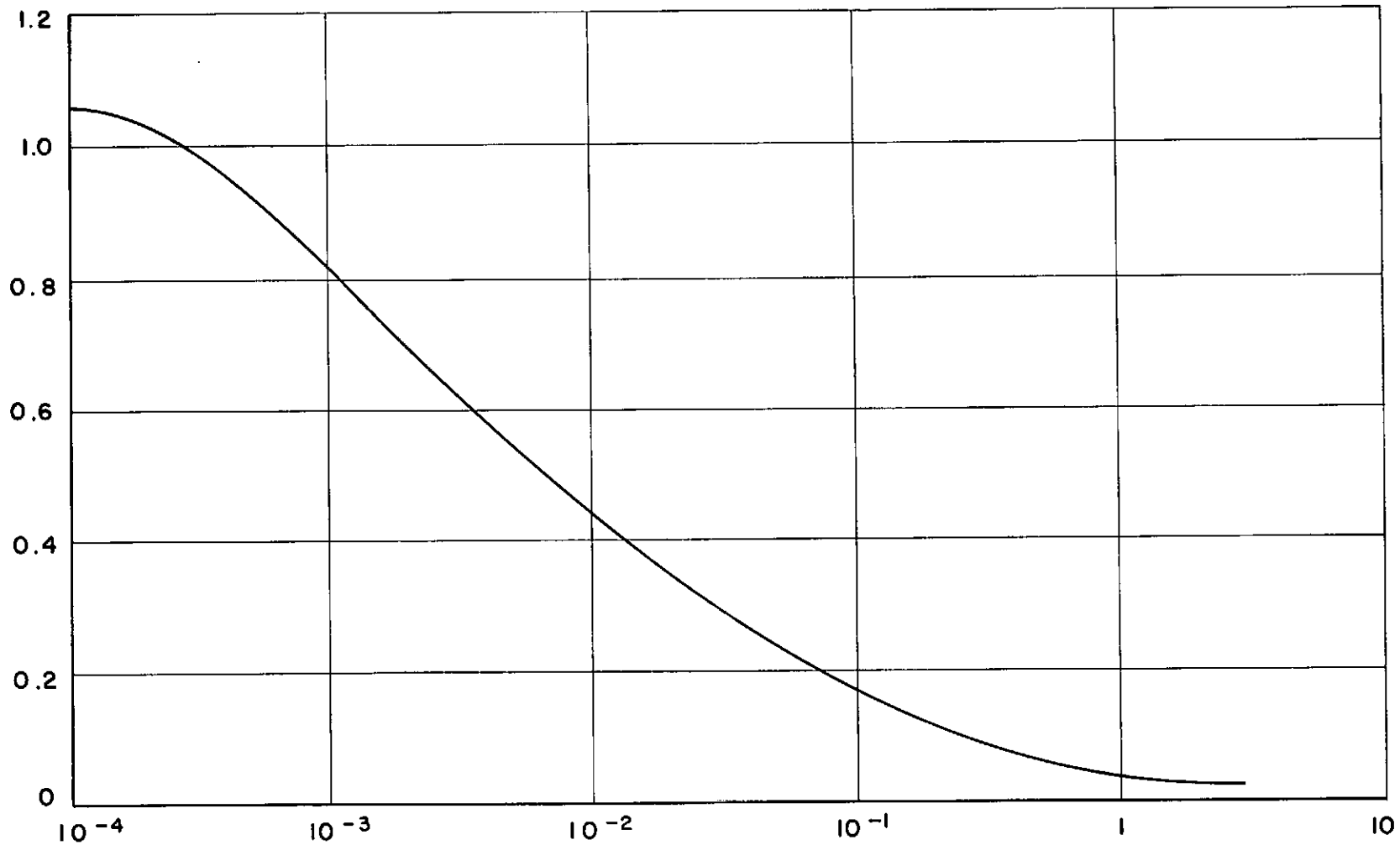
DEFORMAÇÃO CISCALHANTE - % FIGURA 3.4
