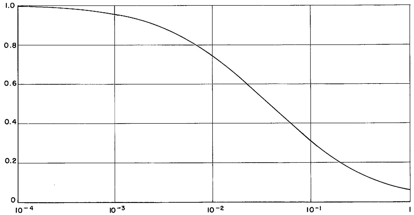
DEFORMAÇÃO CISALHANTE - % FIGURA 3.2
